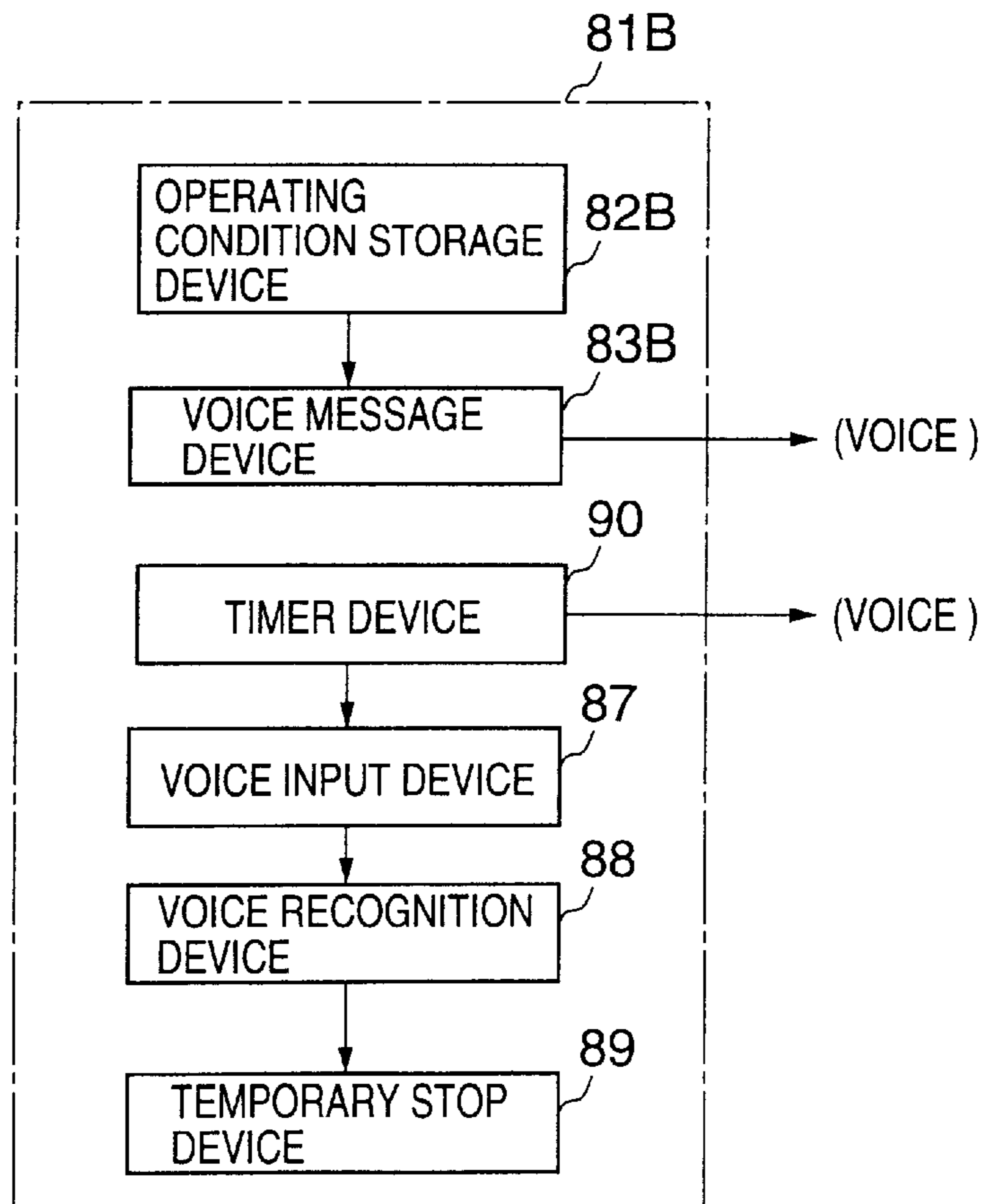
FIG. 44
