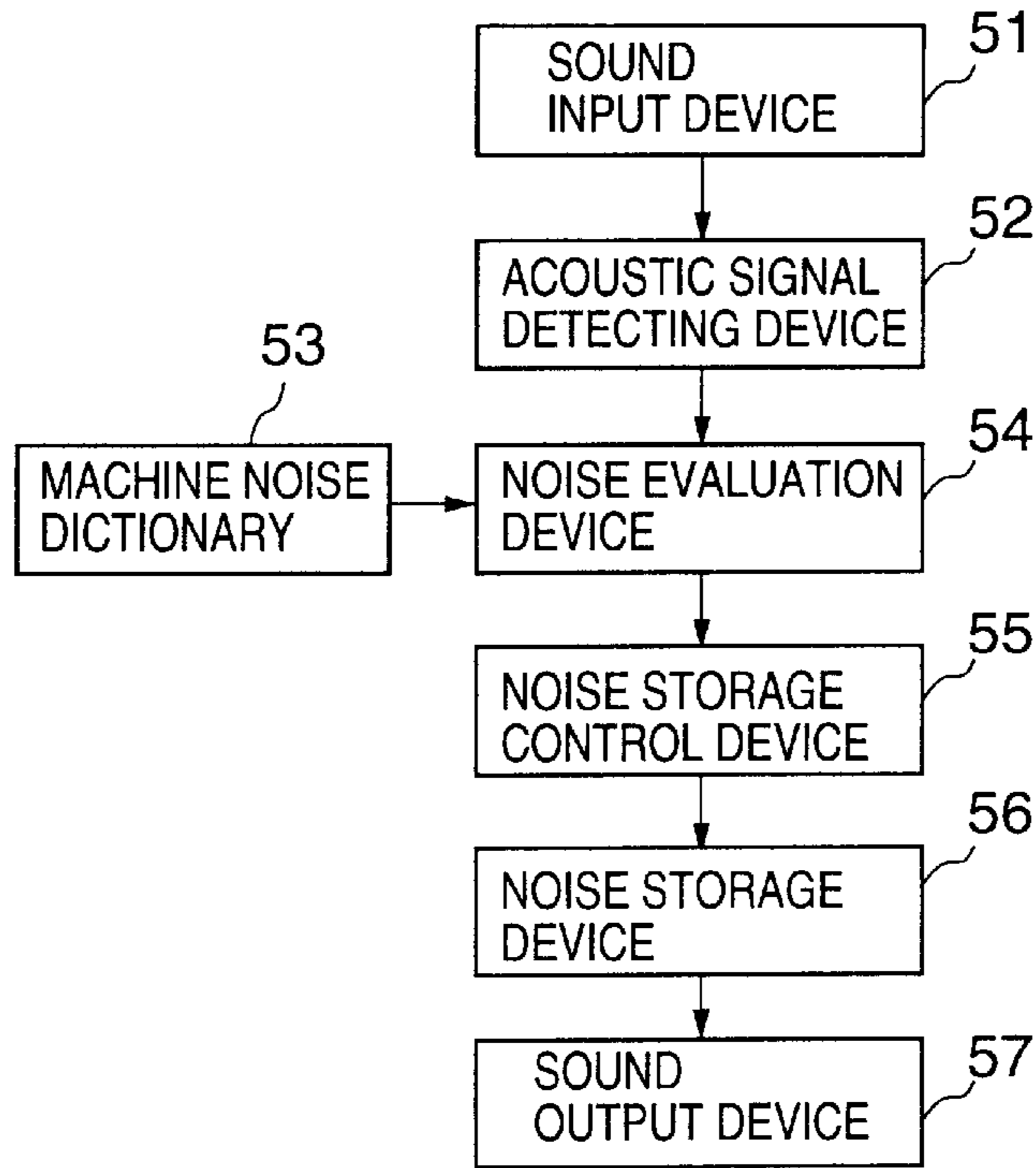
FIG. 32
