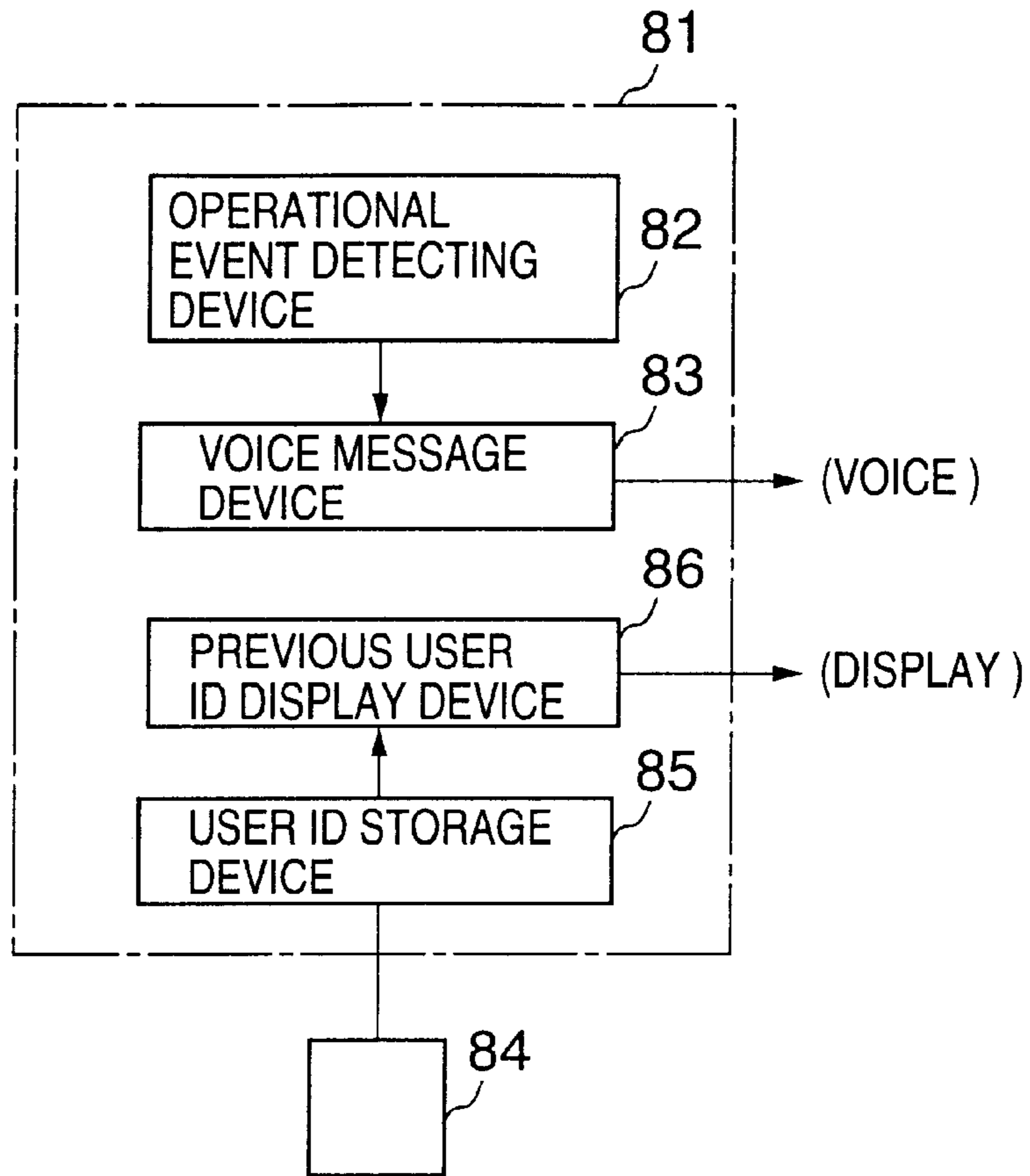
FIG. 41
