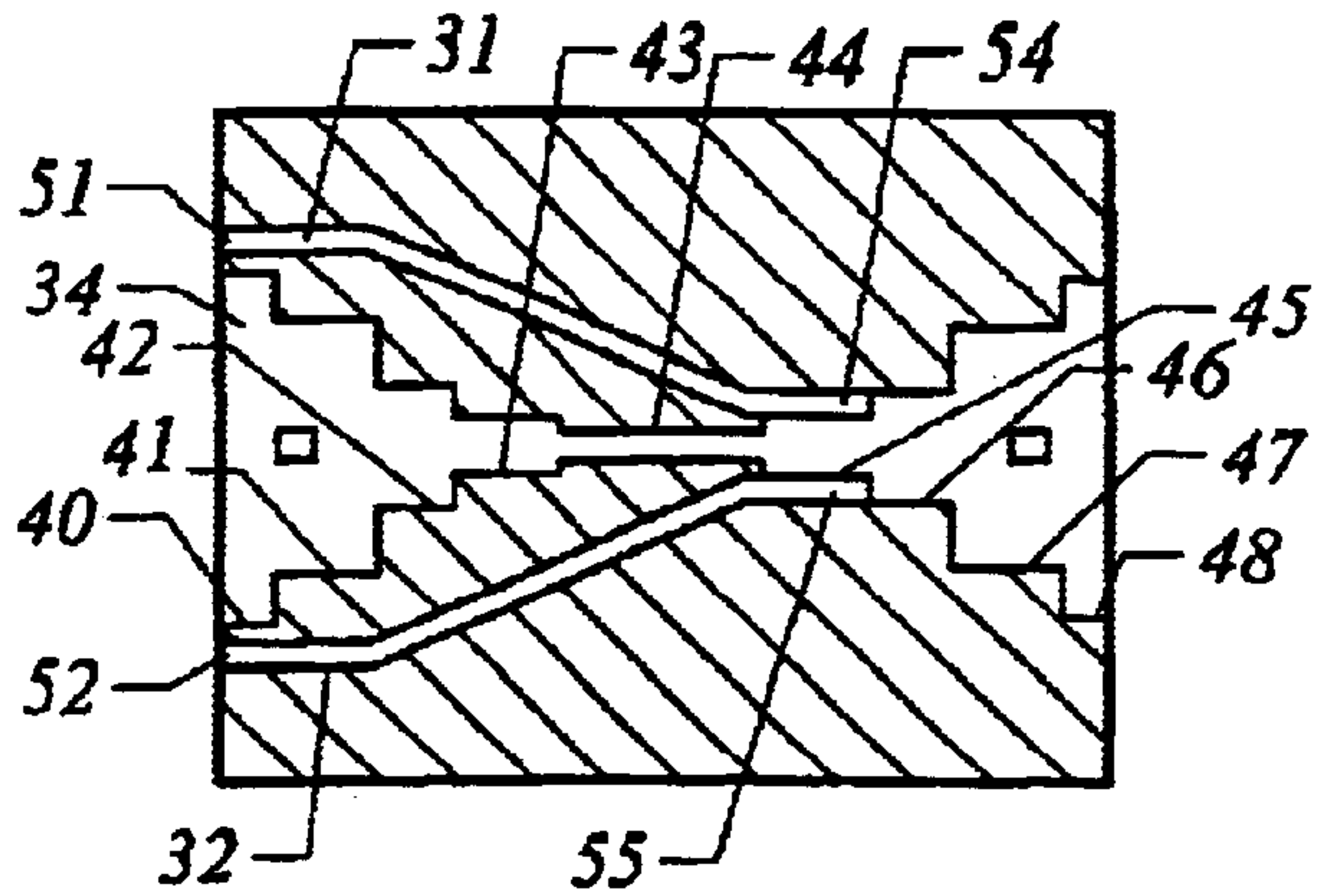
SECTION A-A FIG. 3B
