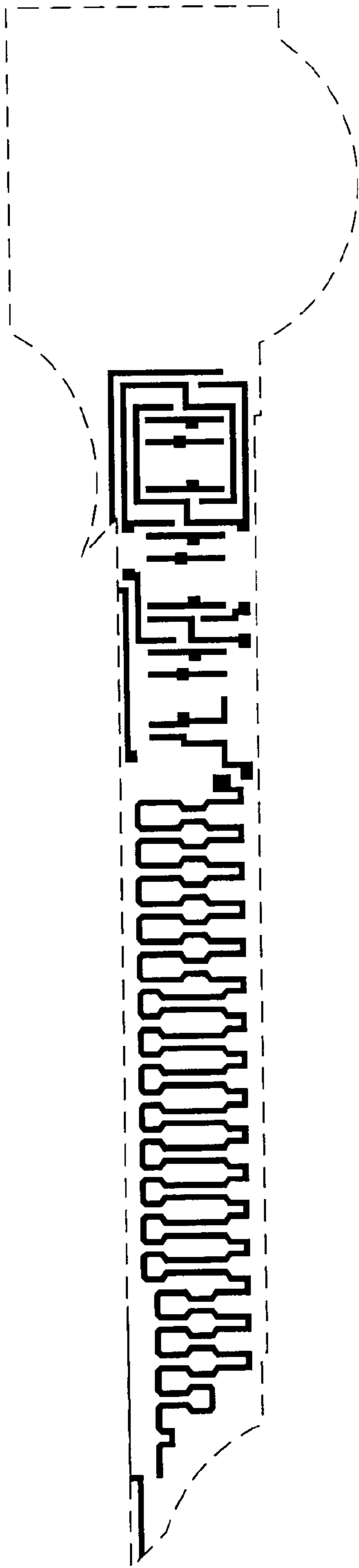
Poly mask
