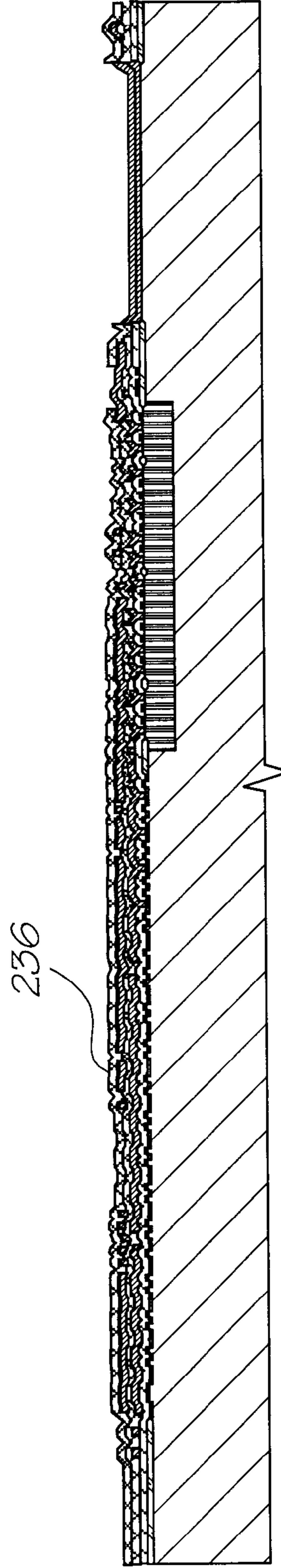
Deposit ILD 3, etch vias
