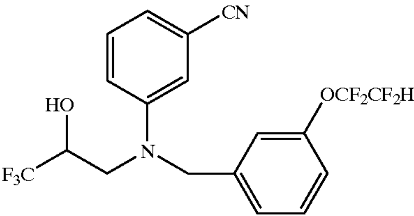
EXAMPLE 576
