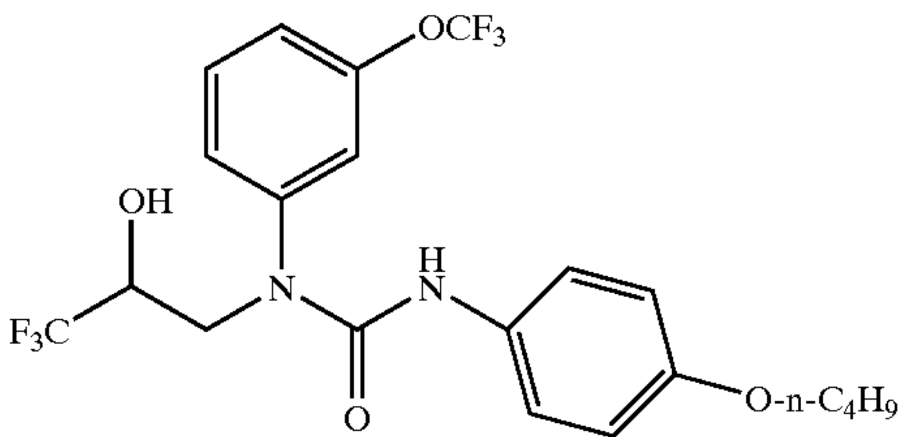
EXAMPLE 367
