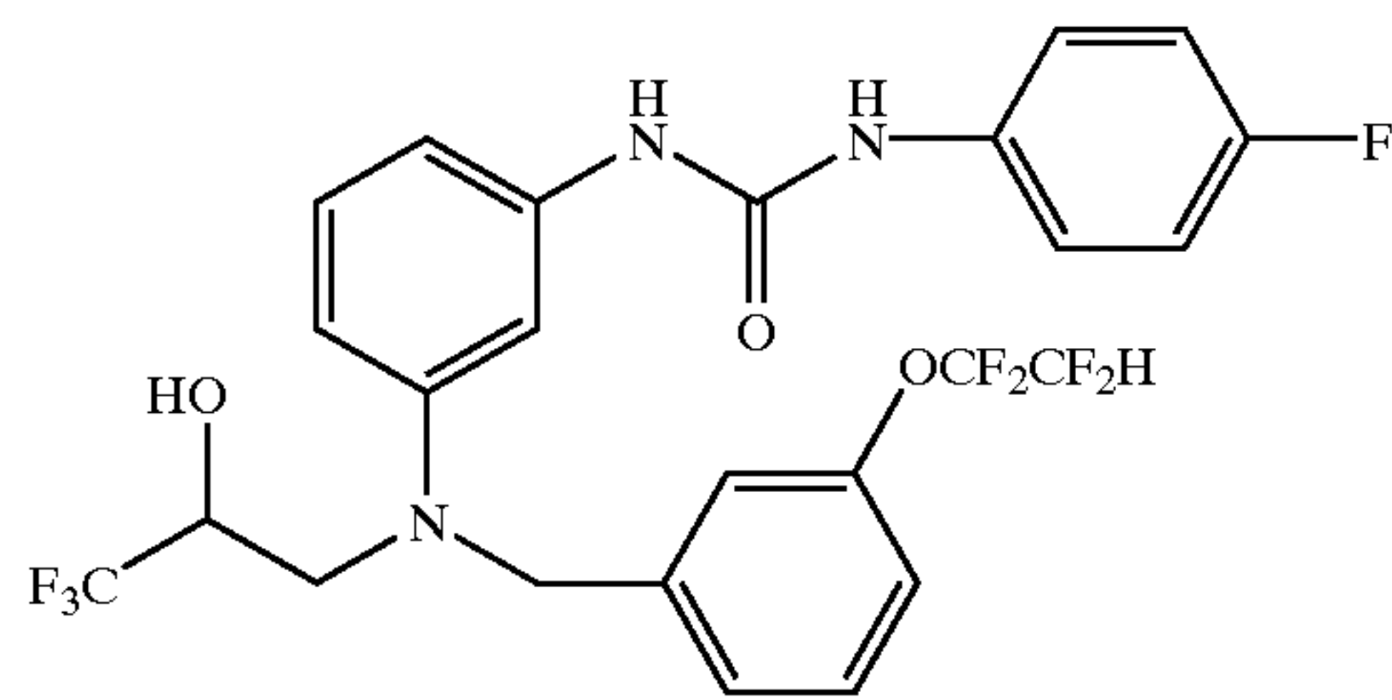
175 EXAMPLE 545
