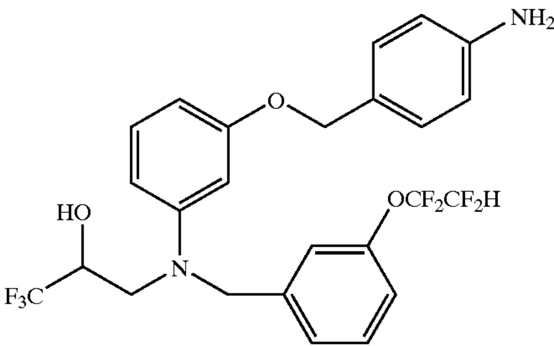
EXAMPLE 434
