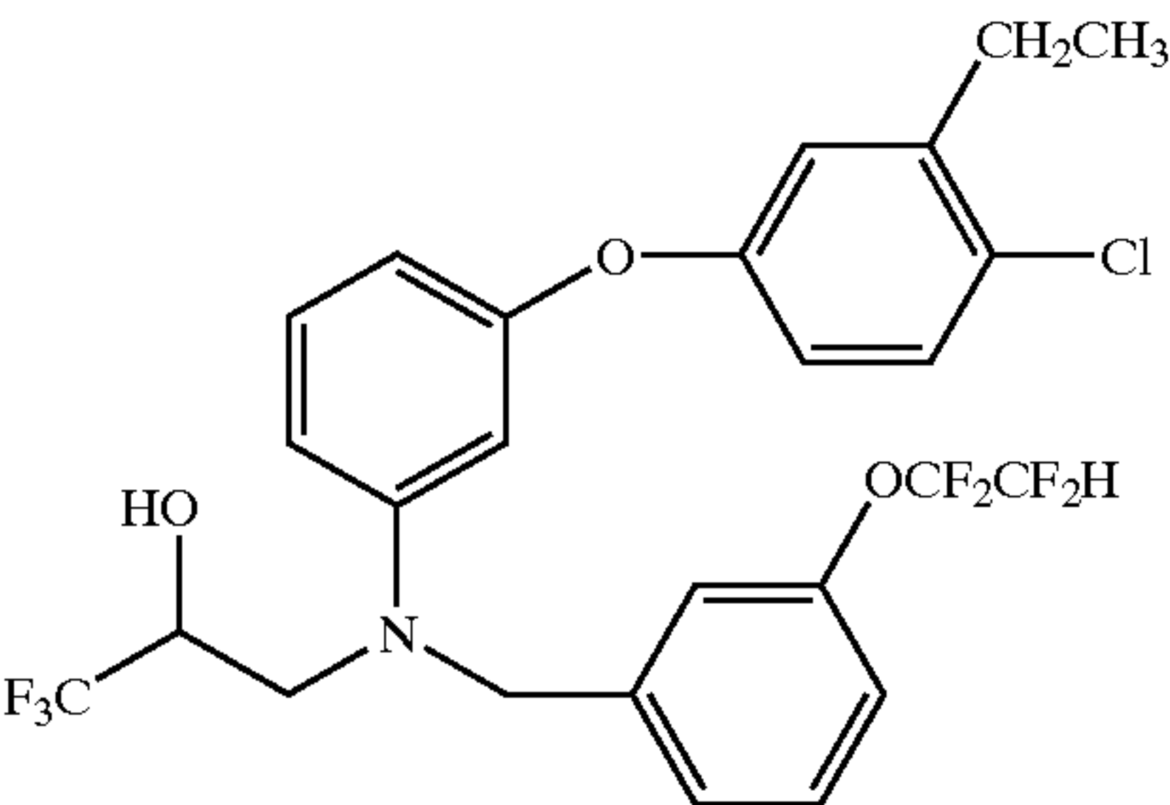
3-[[3-(4-chloro-3-ethylphenoxy)phenyl]-[[3-(1,1,2,2-tetrafluoroethoxy)phenyl]methyl]amino]-1,1,1-trifluoro-2-propanol
