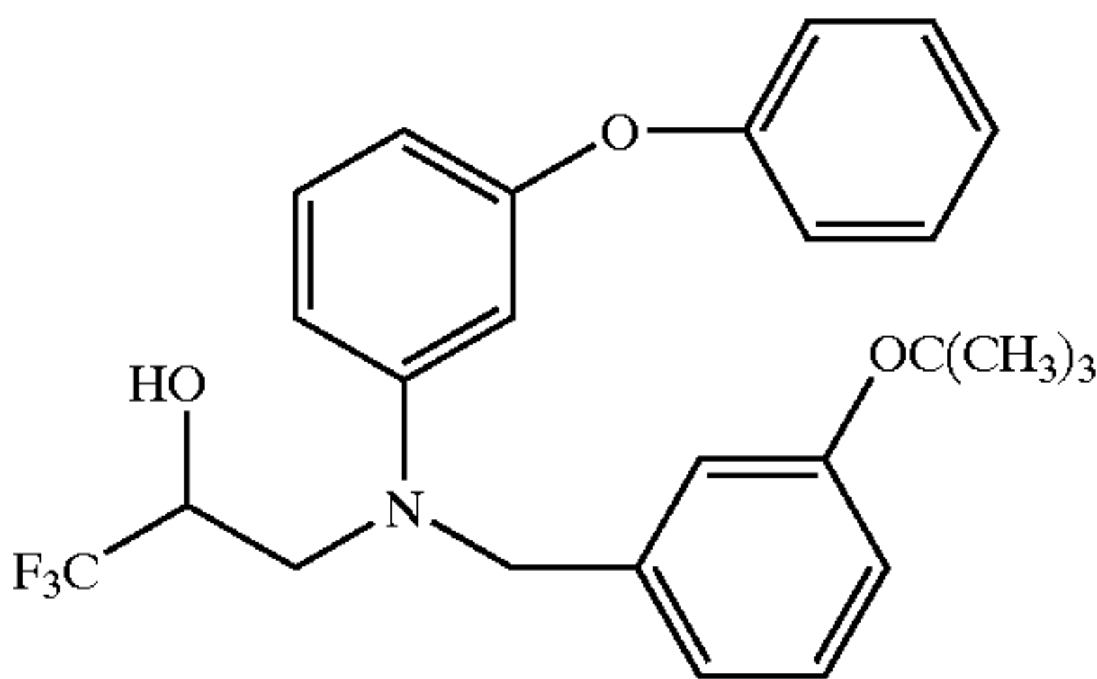
EXAMPLE 654
