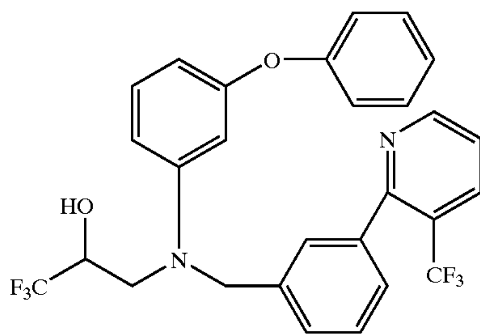
3-[(3-phenoxyphenyl)[[3-(3-trifluoromethyl)-2-pyridinyl]phenyl]methyl]amino]-1,1,1-trifluoro-2-propanol
