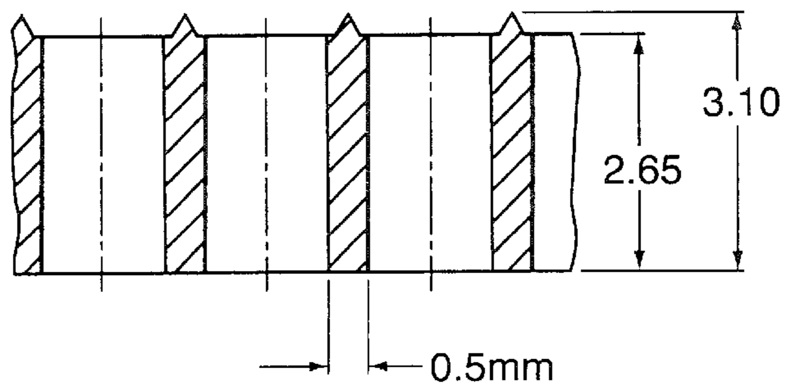
SECTION A-A
