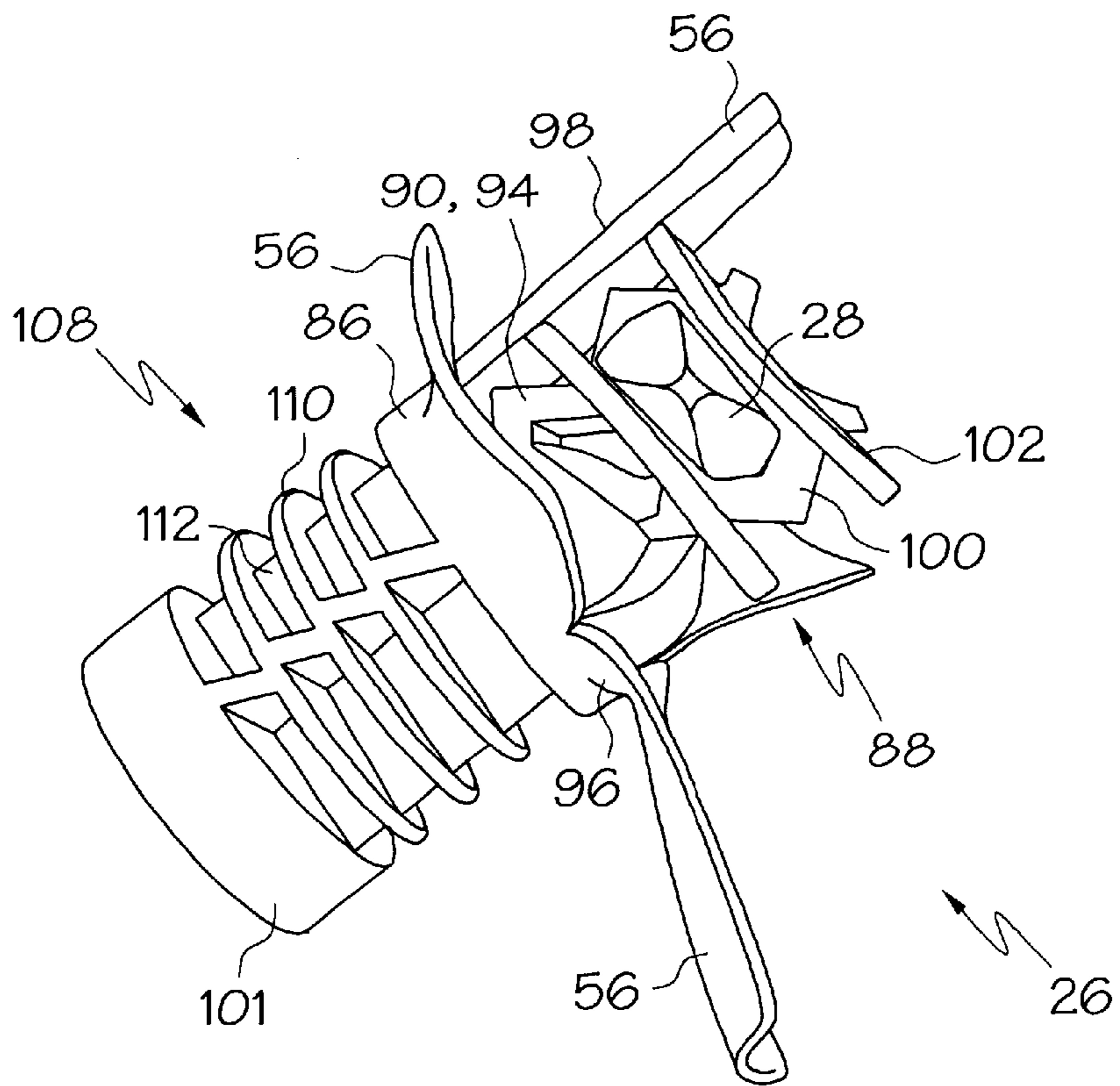
FIG. 23
