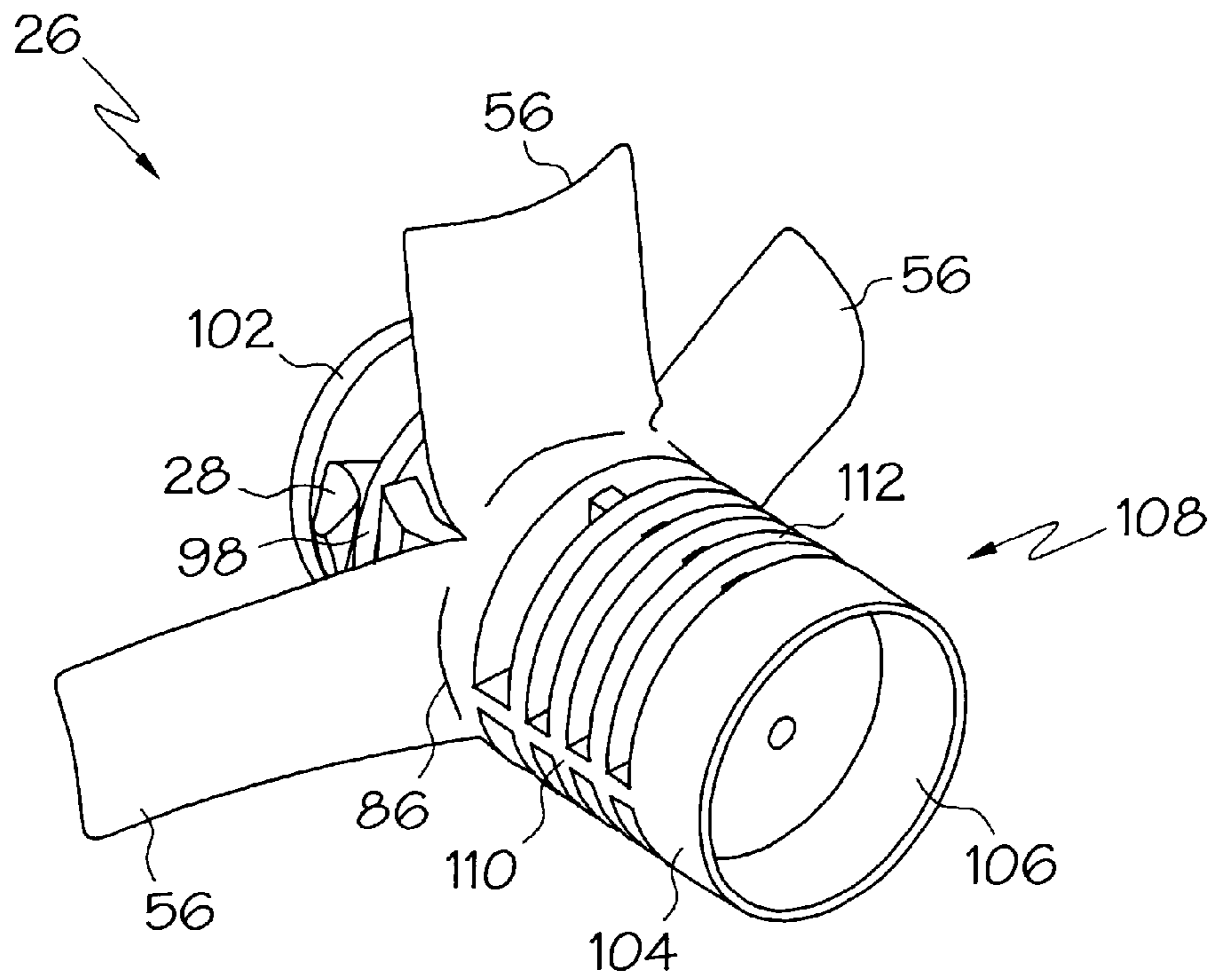
FIG. 21
