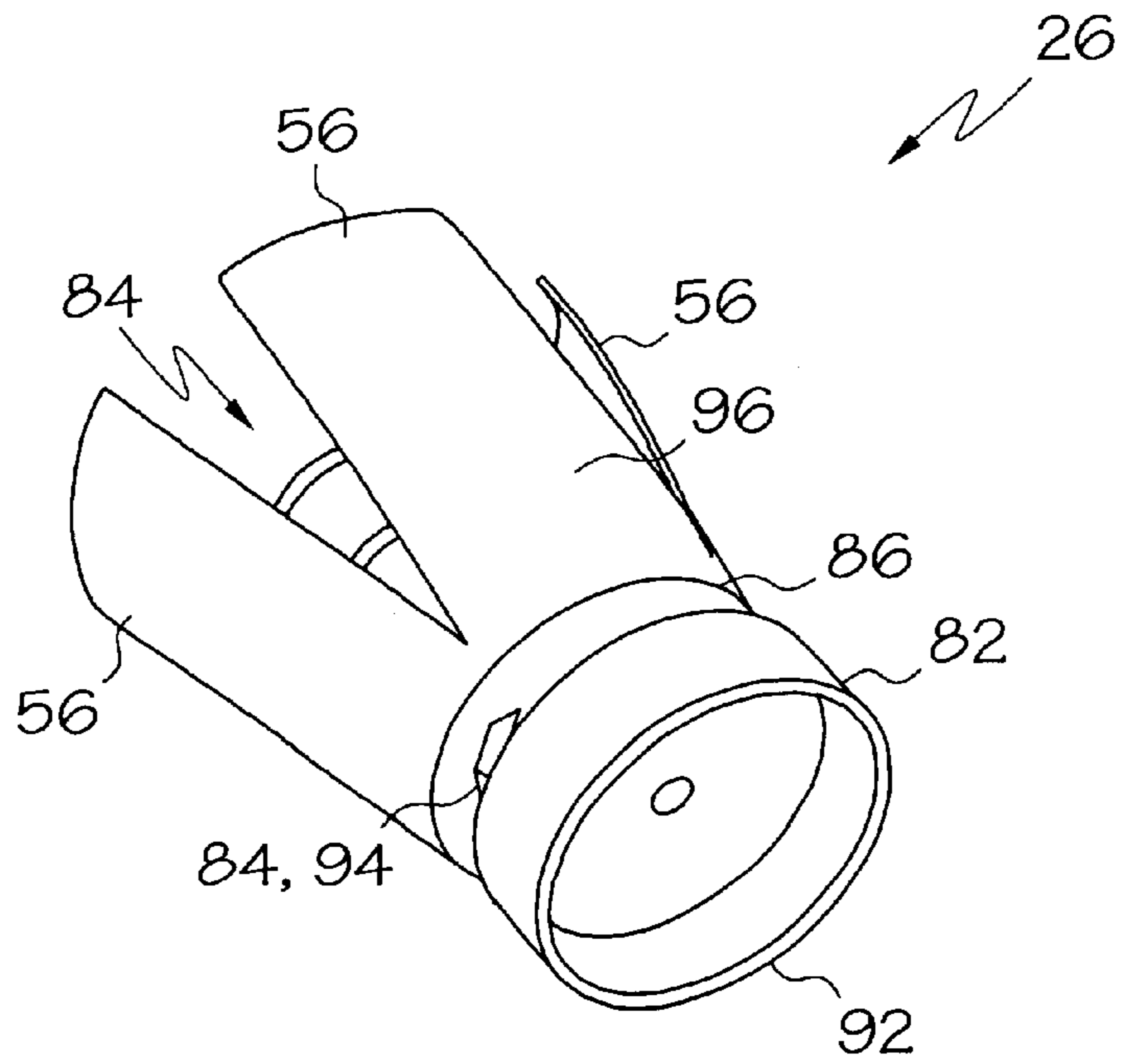
FIG. 20
