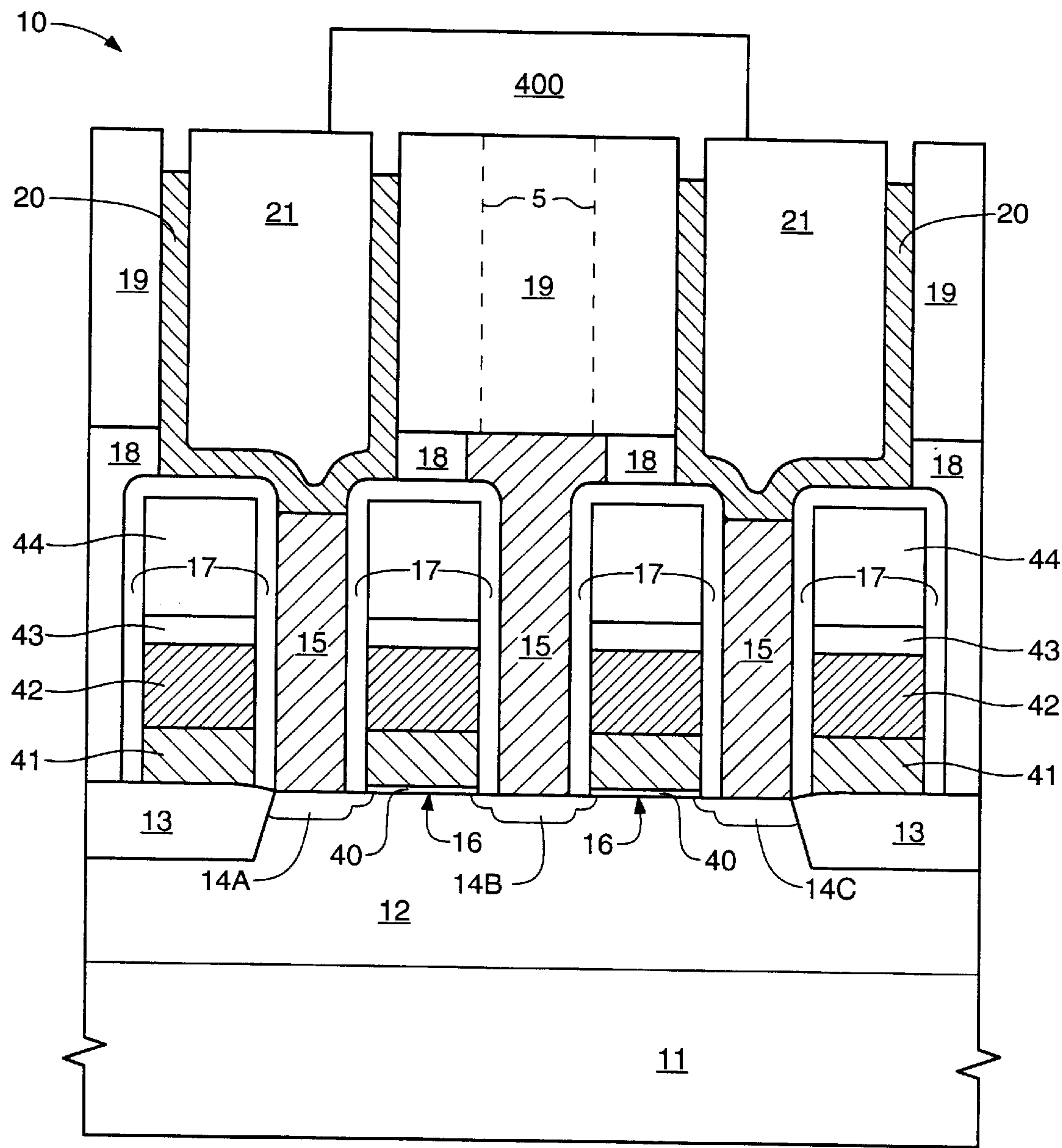
FIG. 15C
