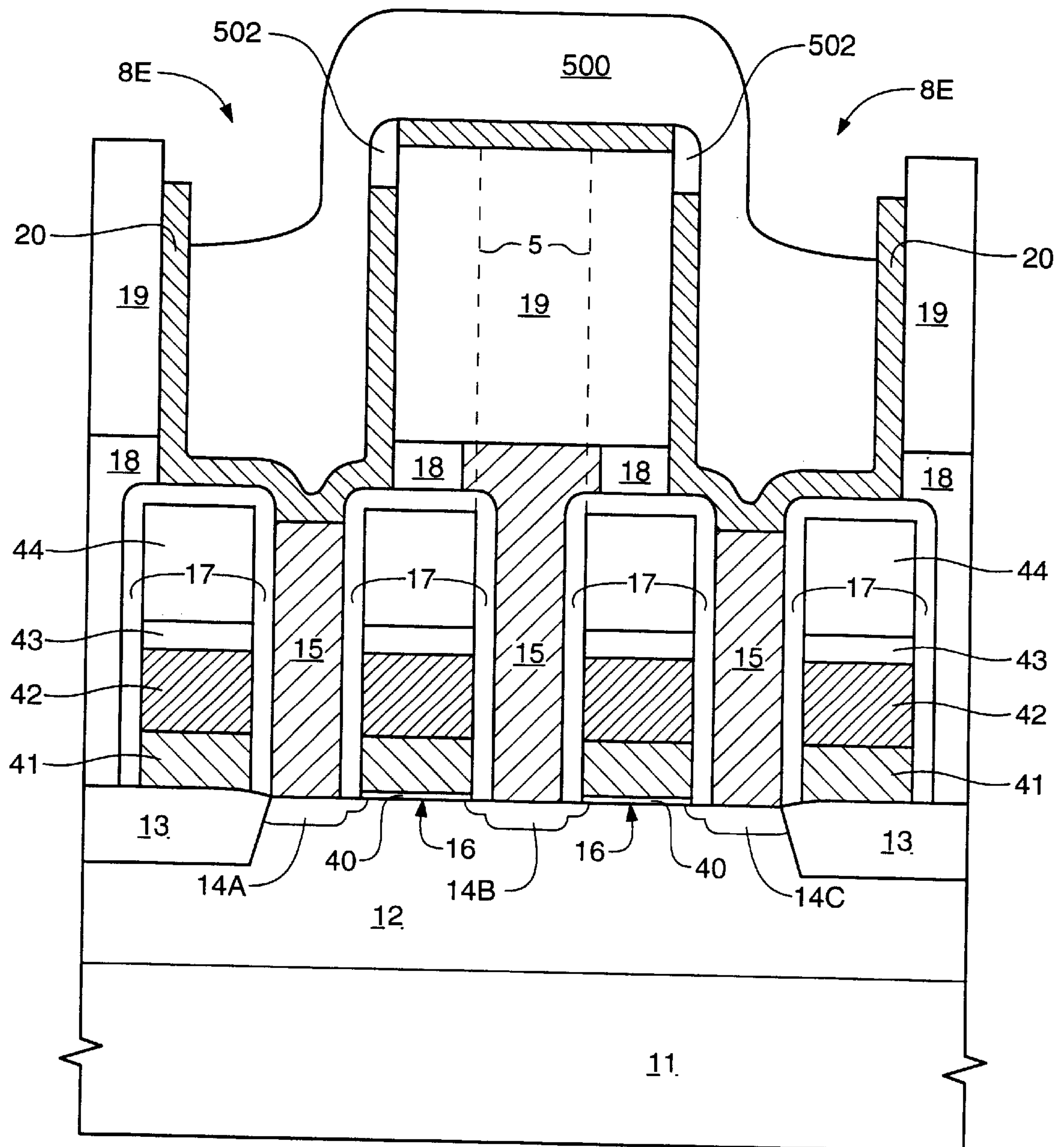
FIG. 18C
