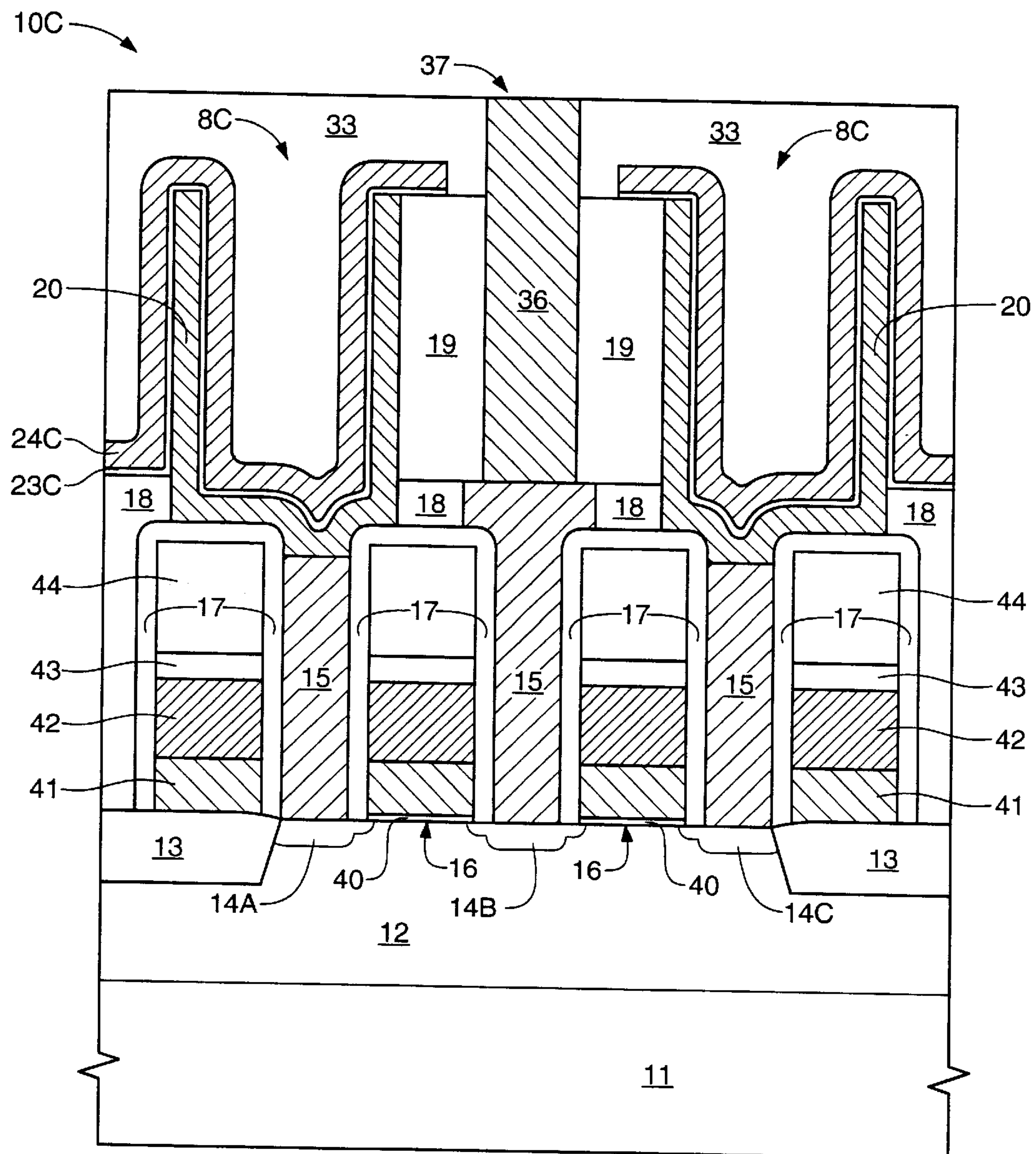
FIG. 11A
