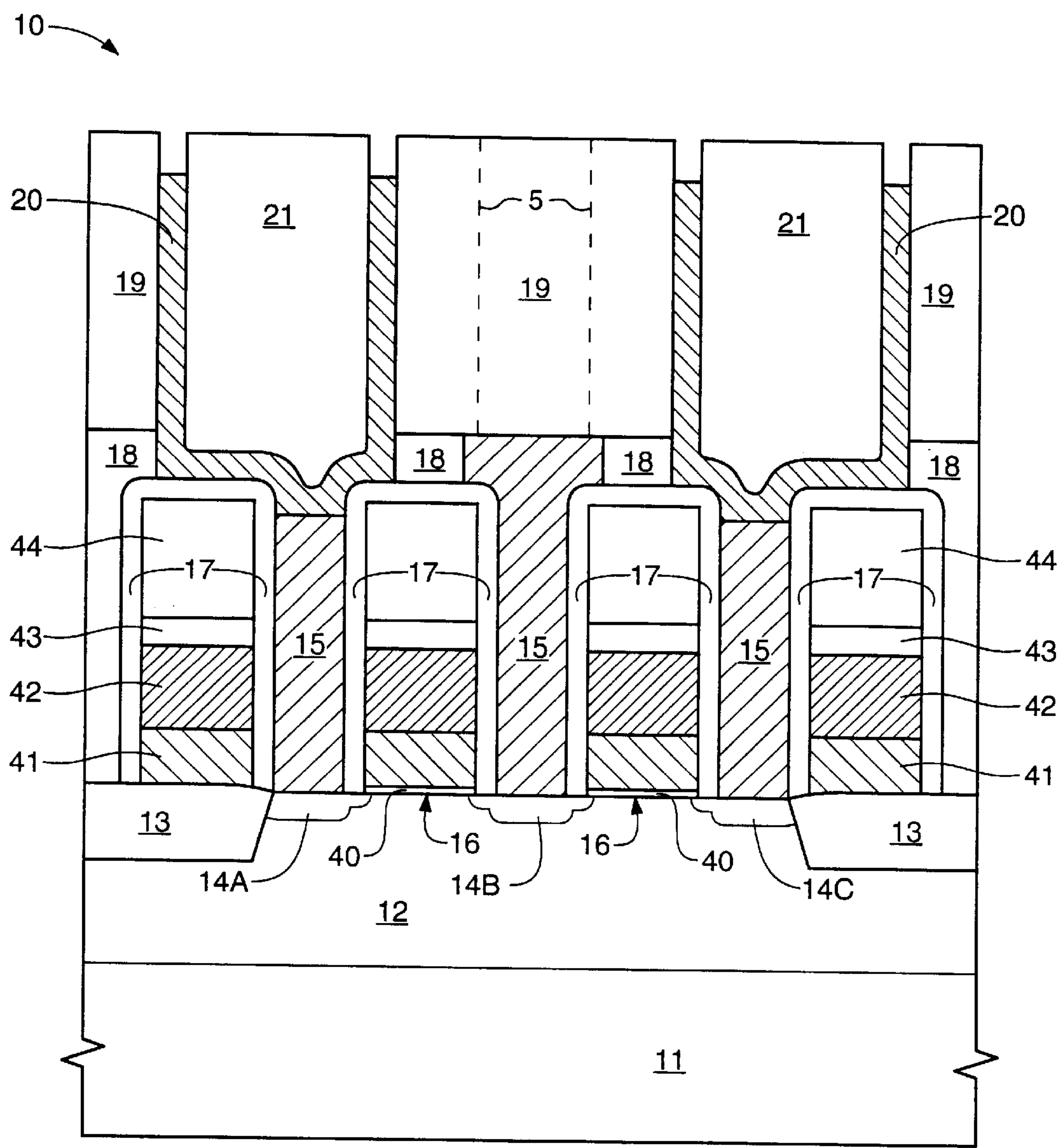
FIG. 15B
