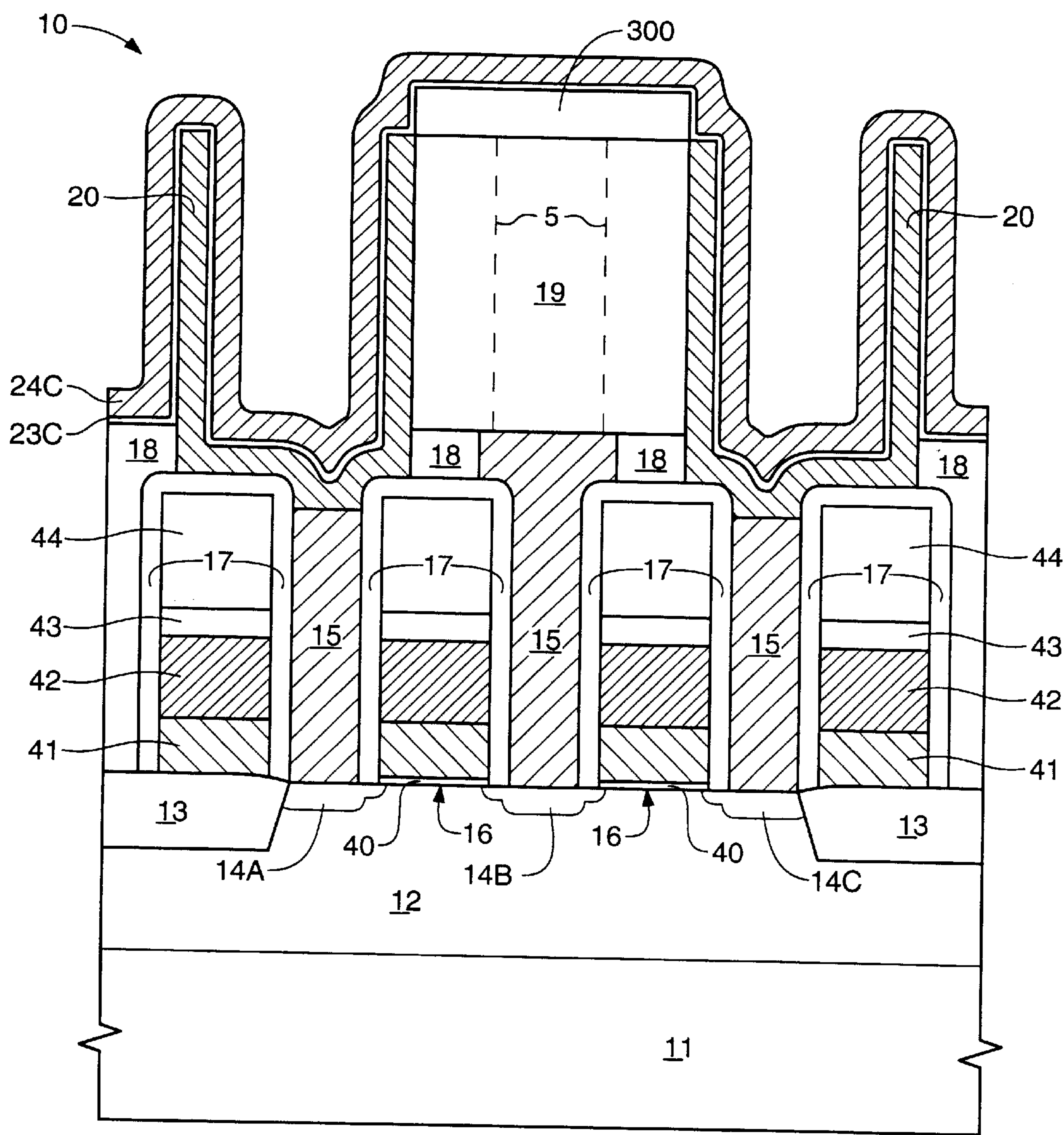
FIG. 14D
