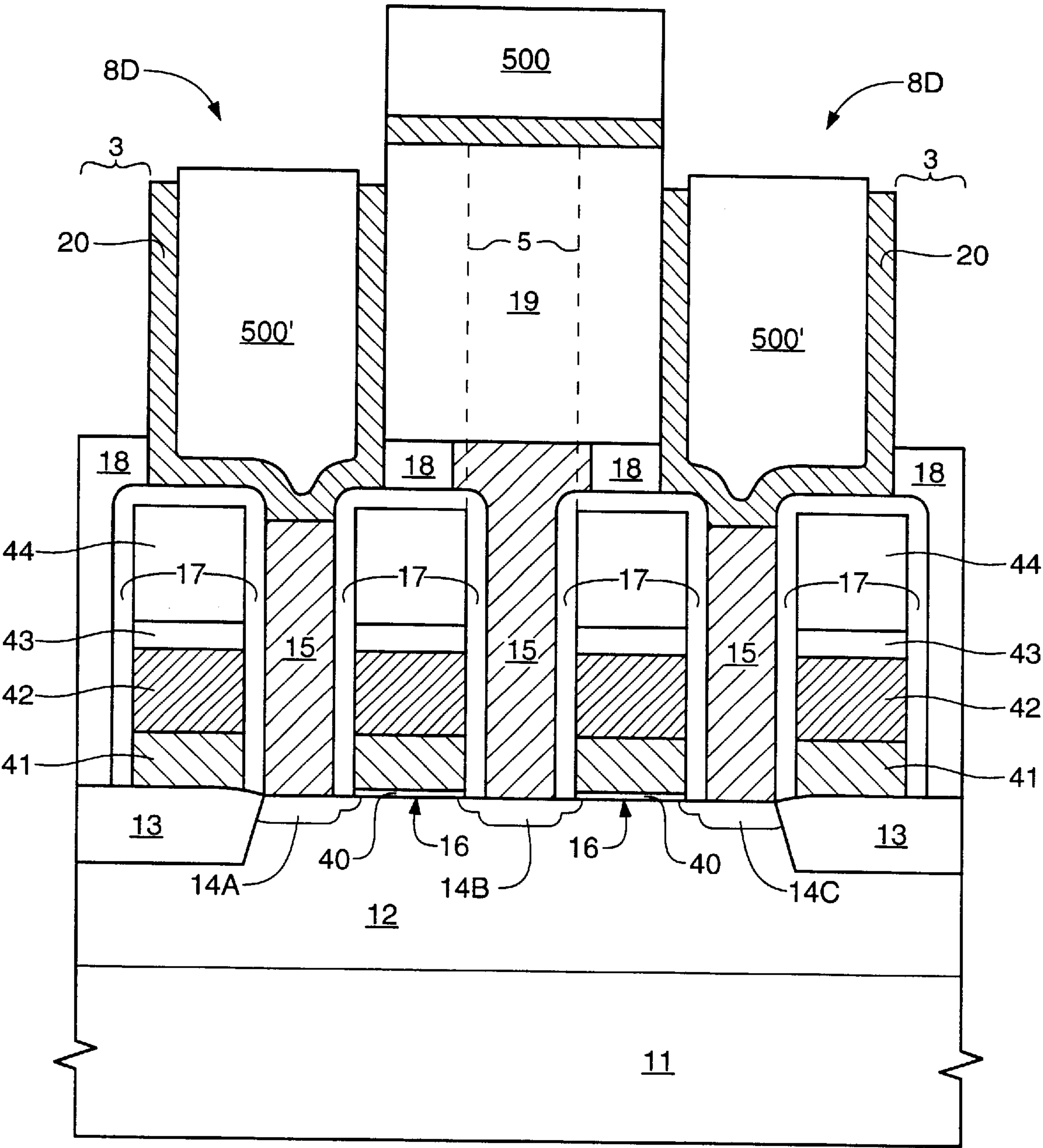
FIG. 17E
