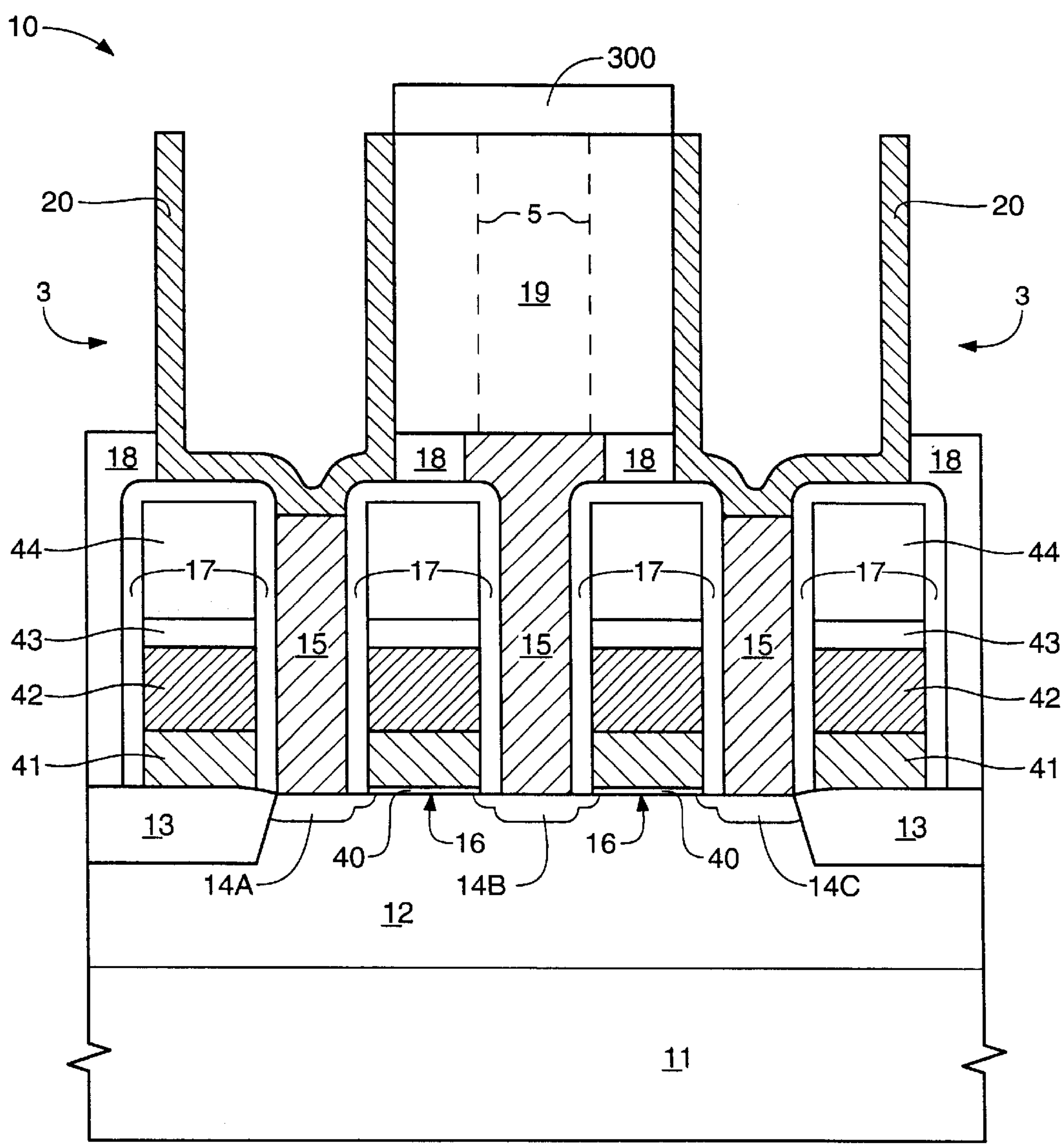
FIG. 14C
