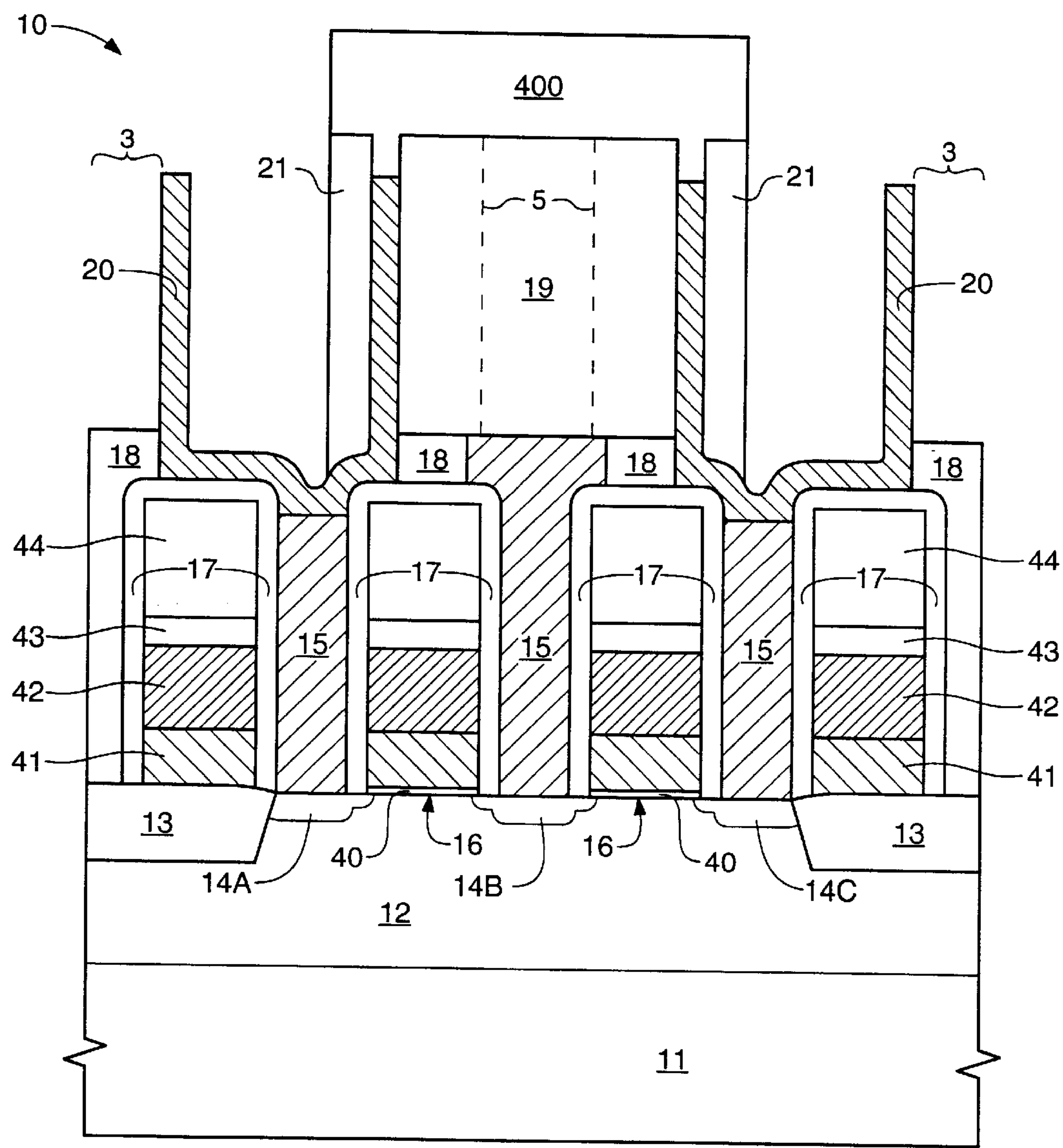
FIG. 15D
