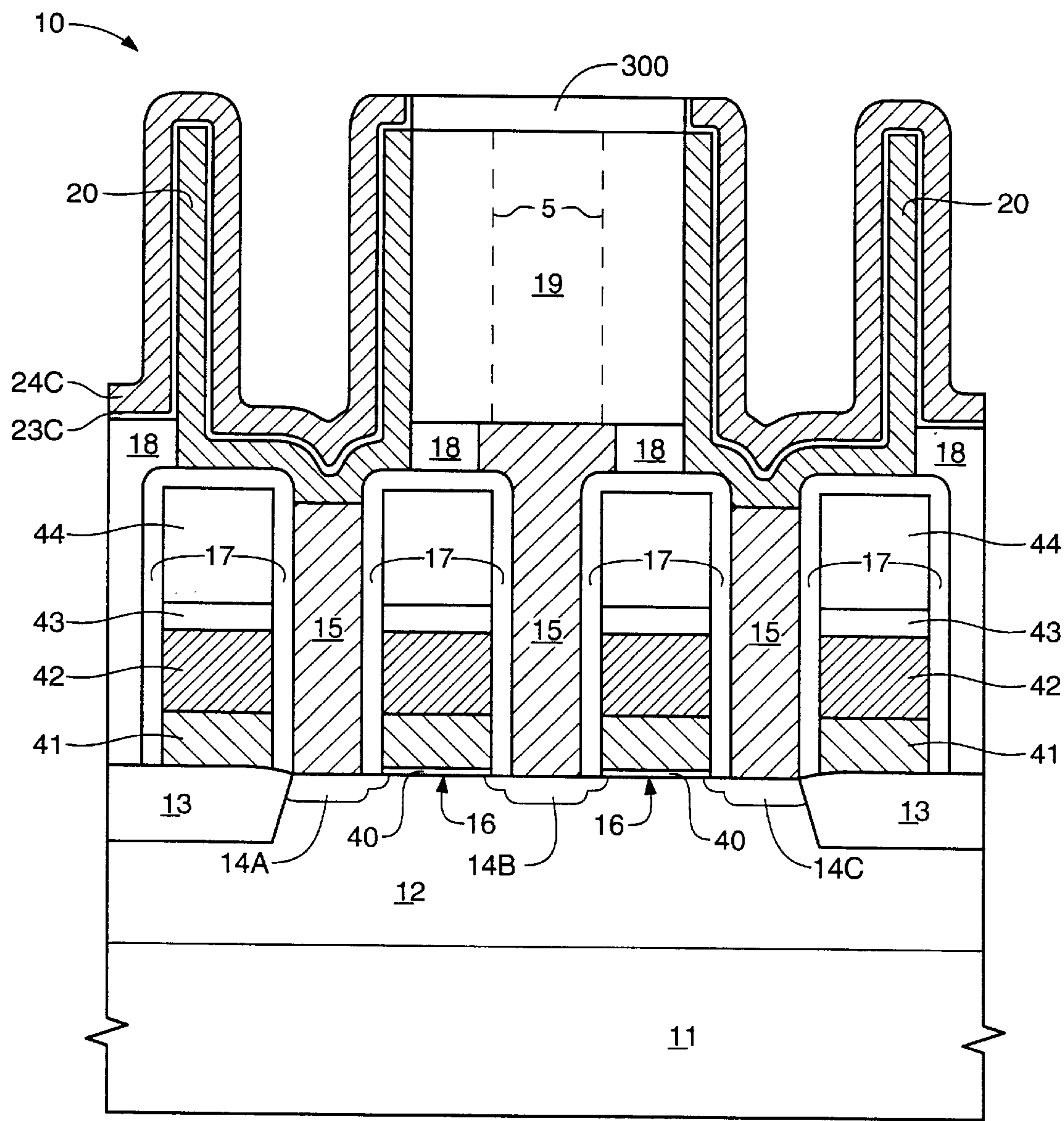
FIG. 14E
