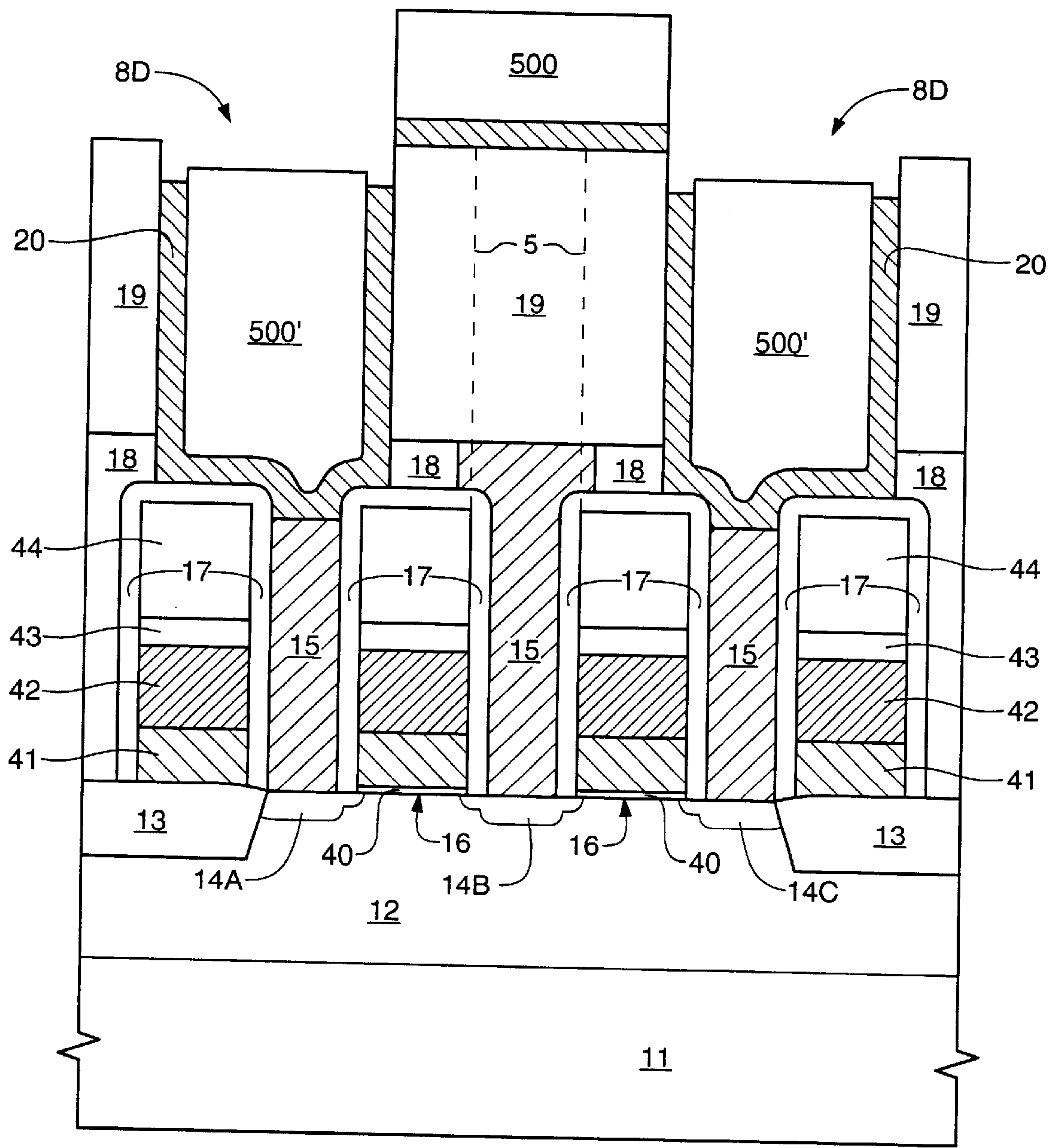
FIG. 17D
