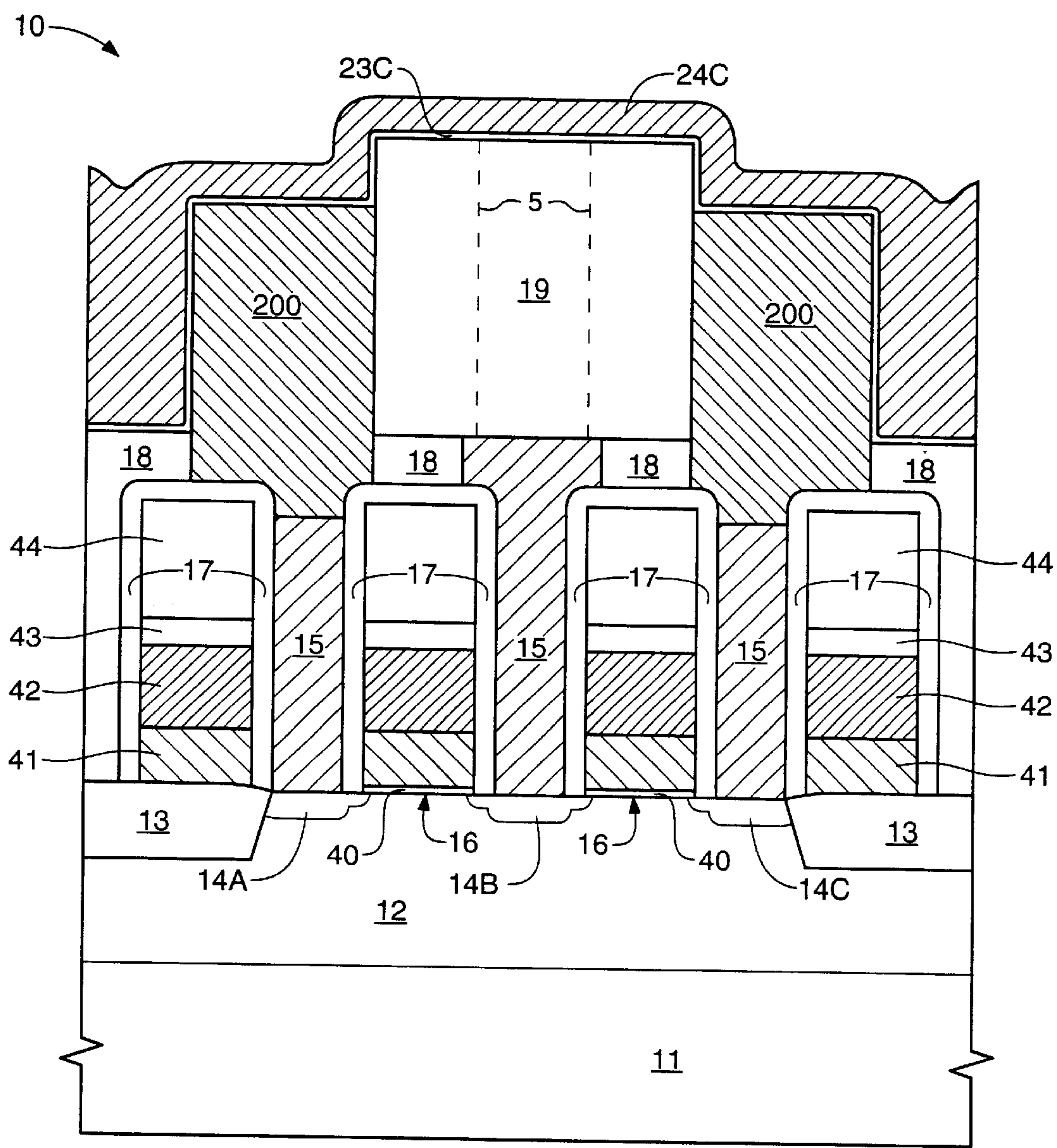
FIG. 16F
