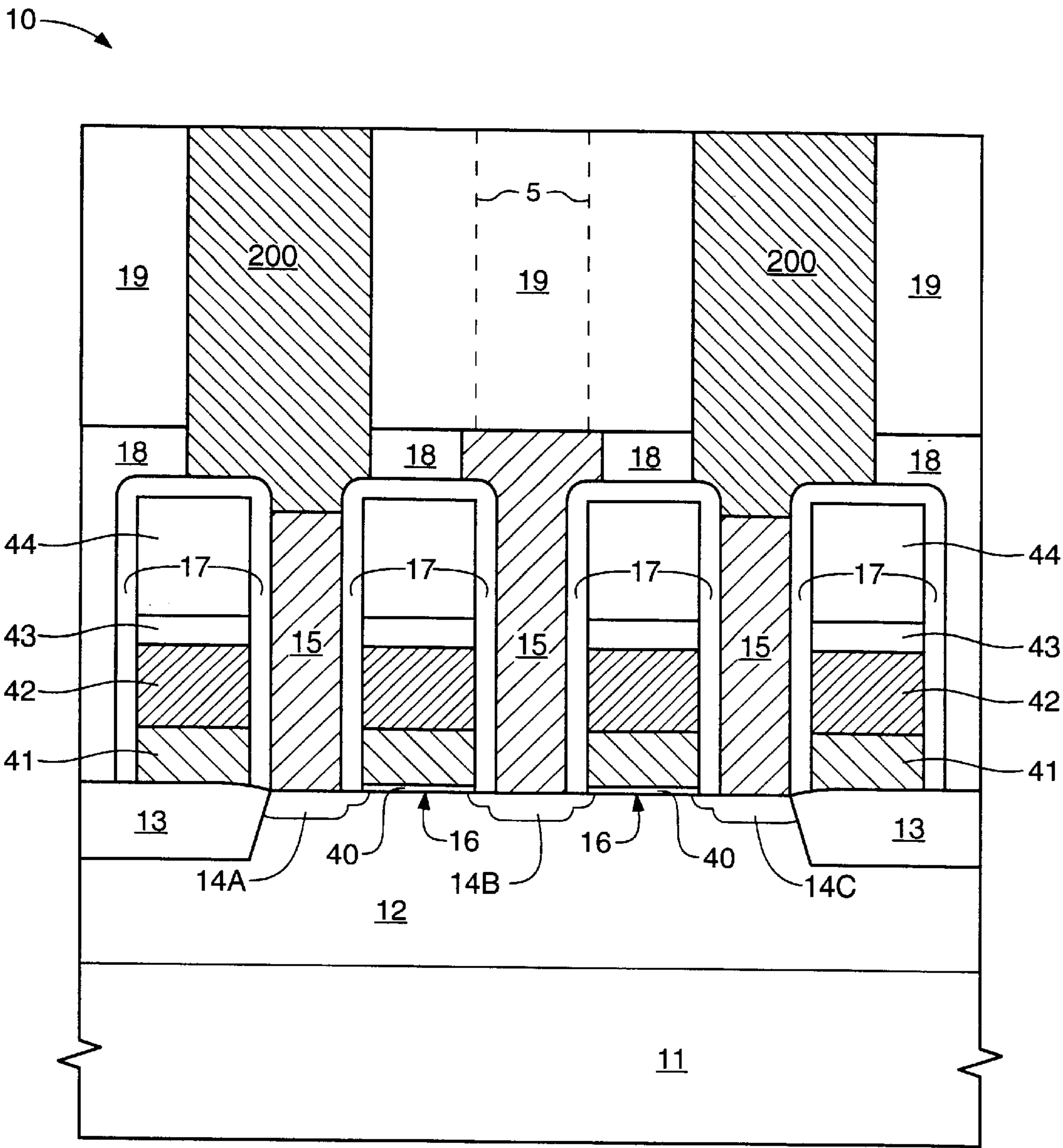
FIG. 16A
