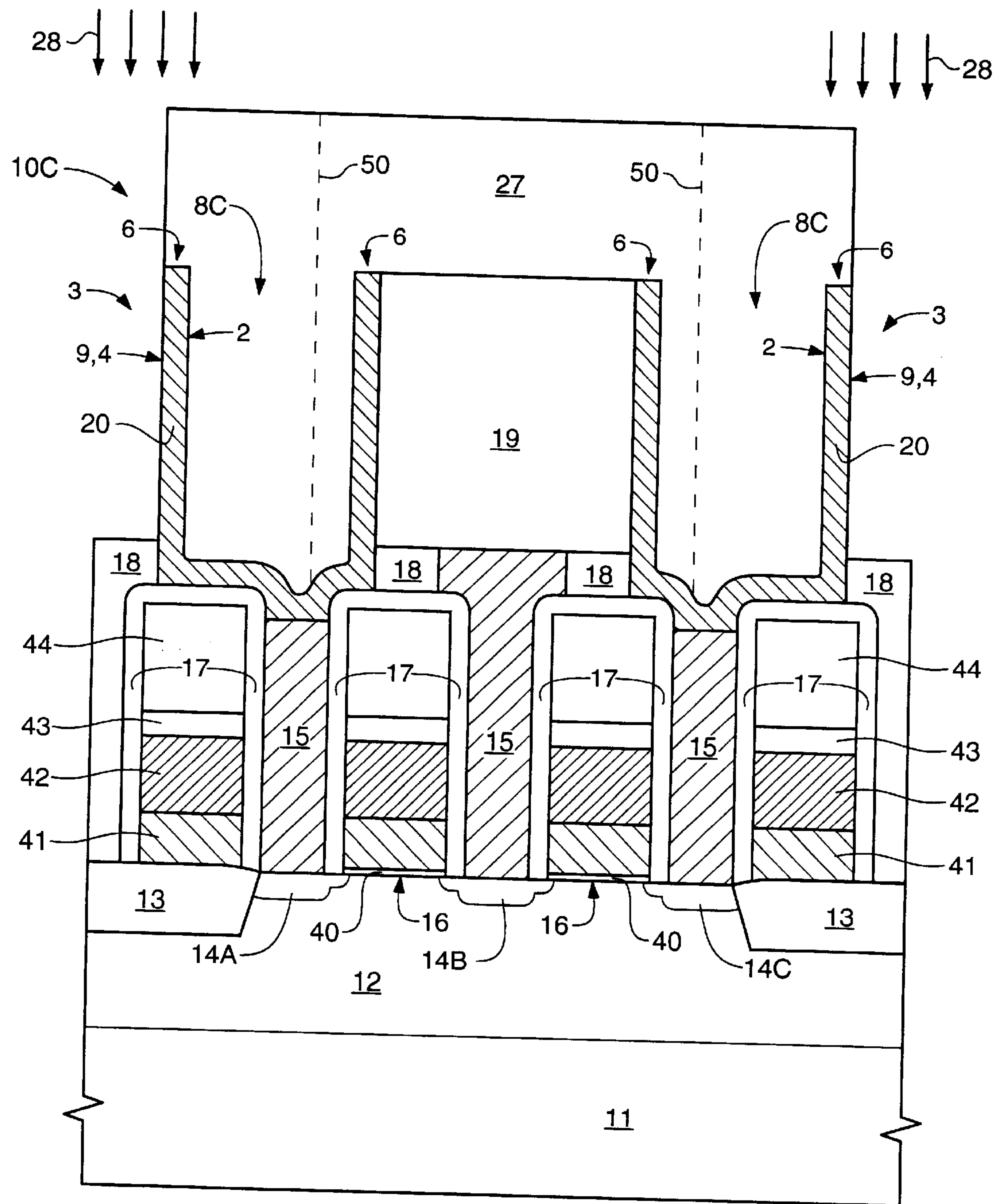
FIG. 7B
