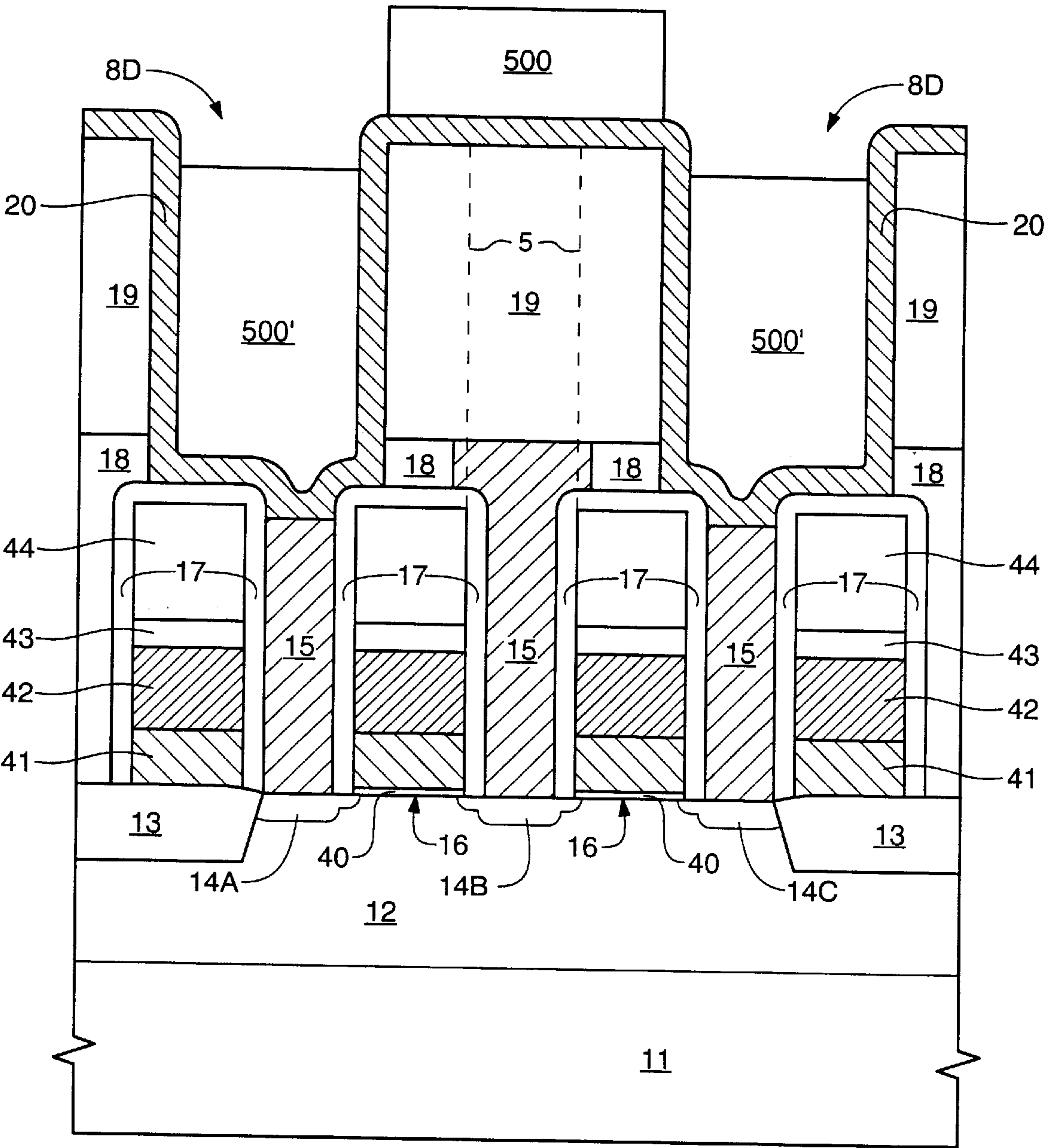
FIG. 17C
