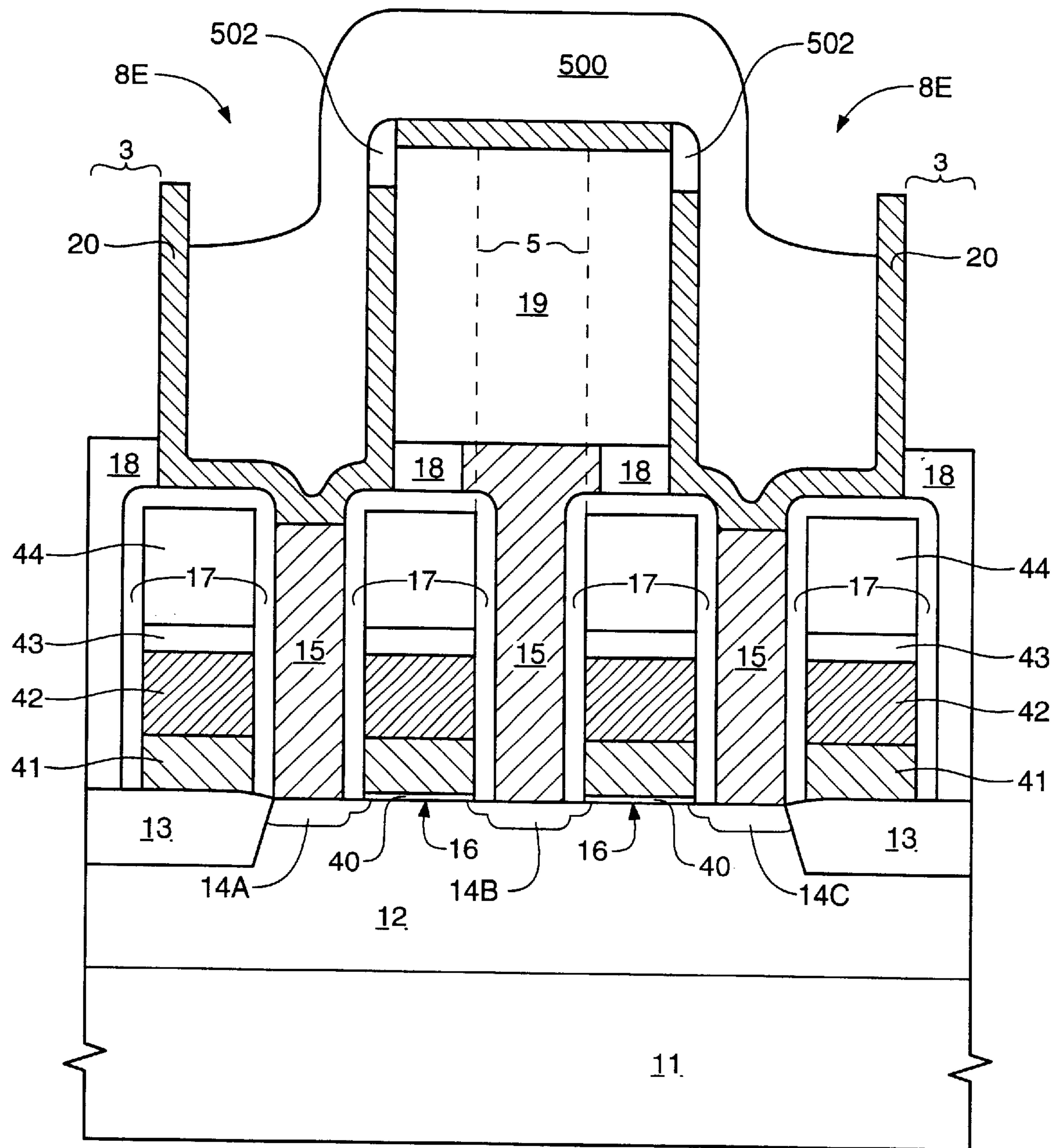
FIG. 18D
