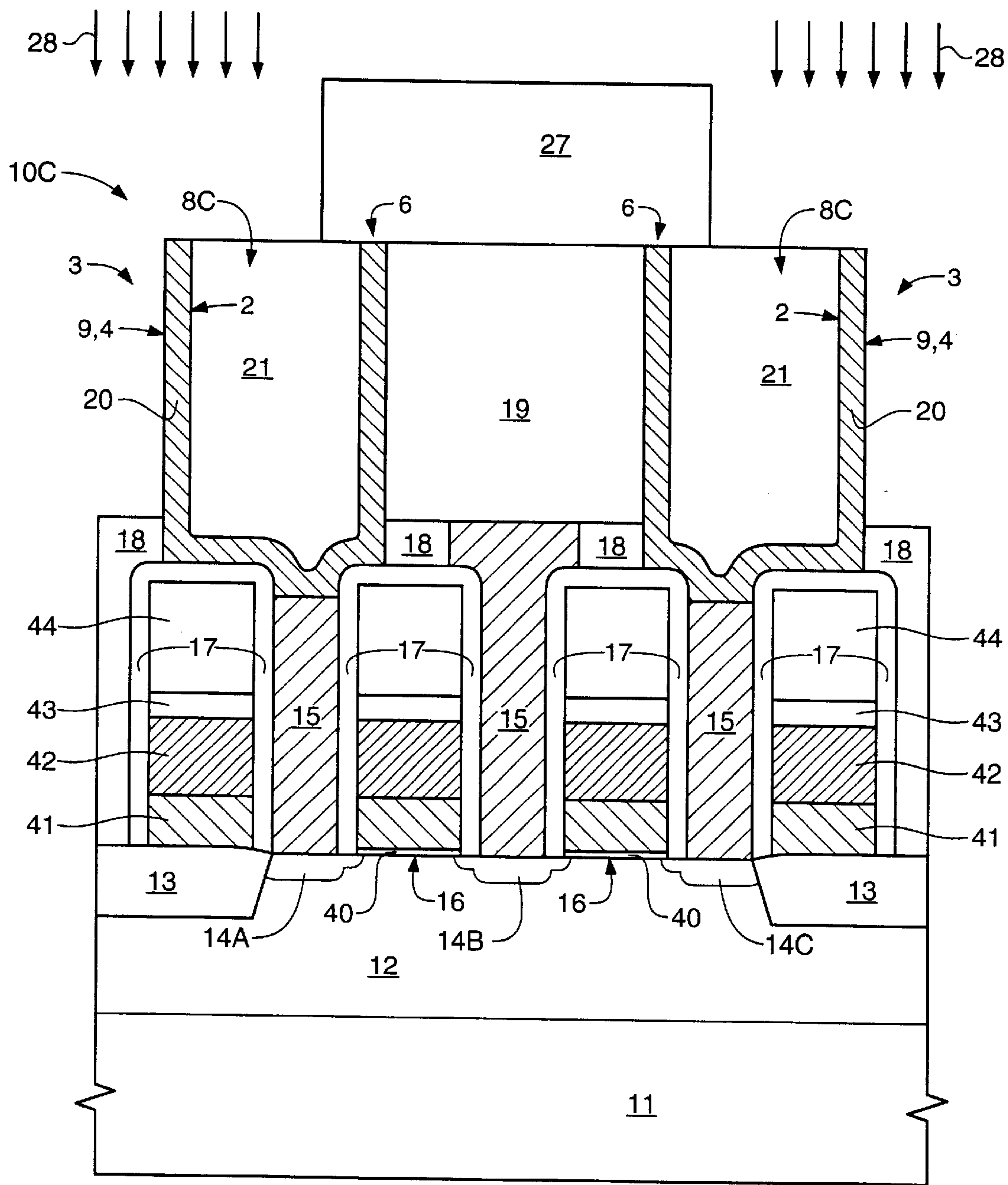
FIG. 7A
