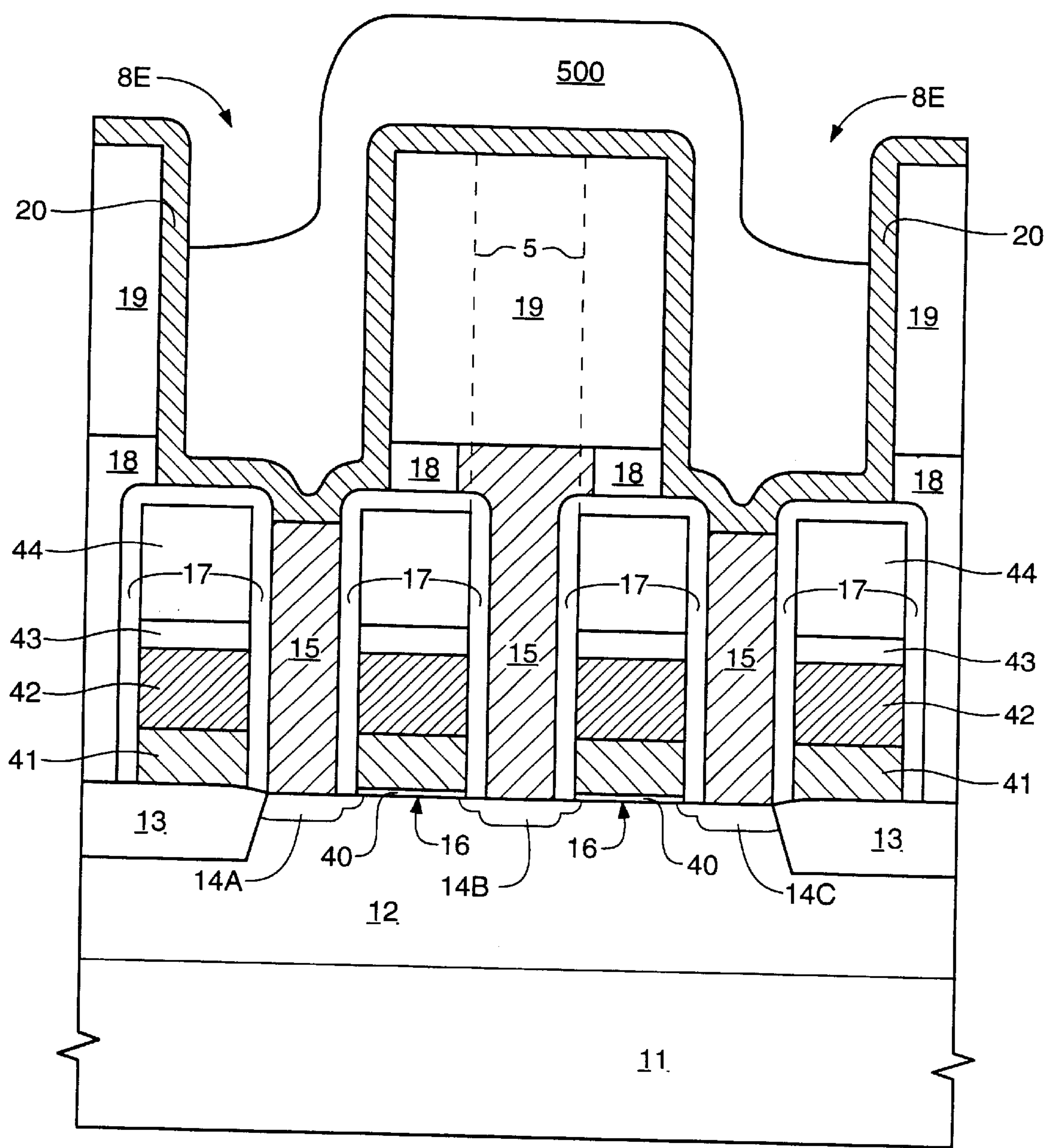
FIG. 18A
