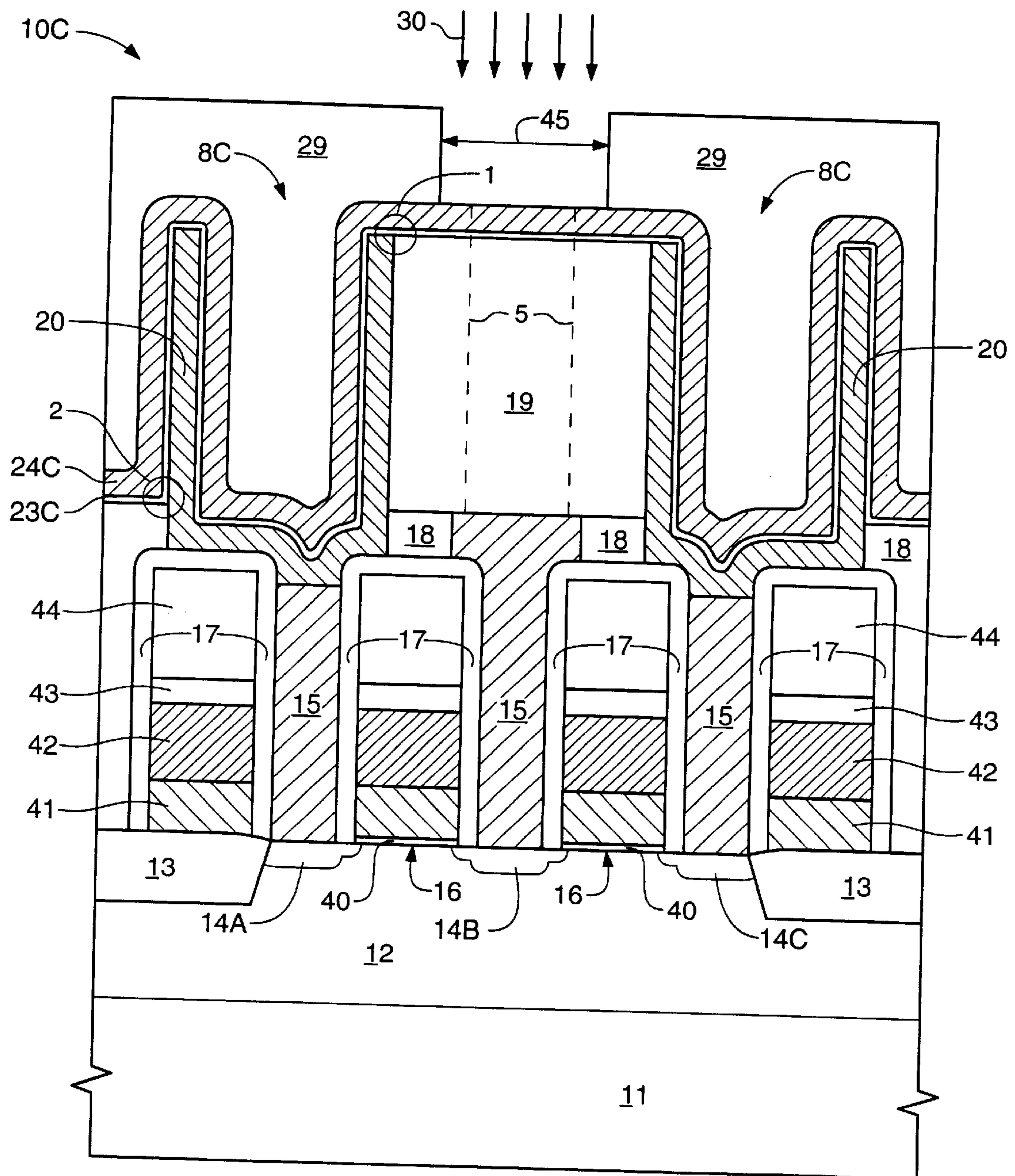
FIG. 8A
