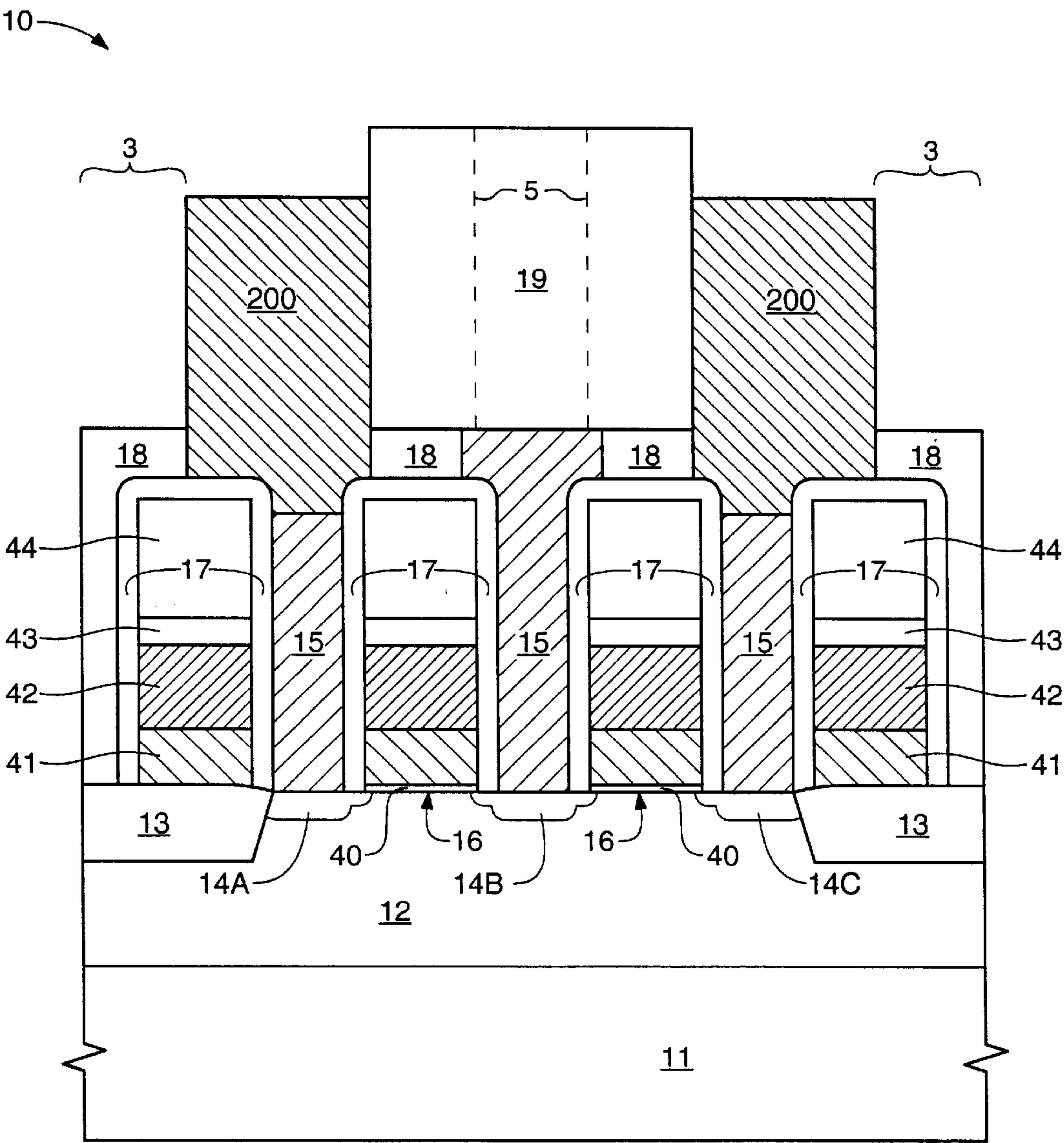
FIG. 16E
