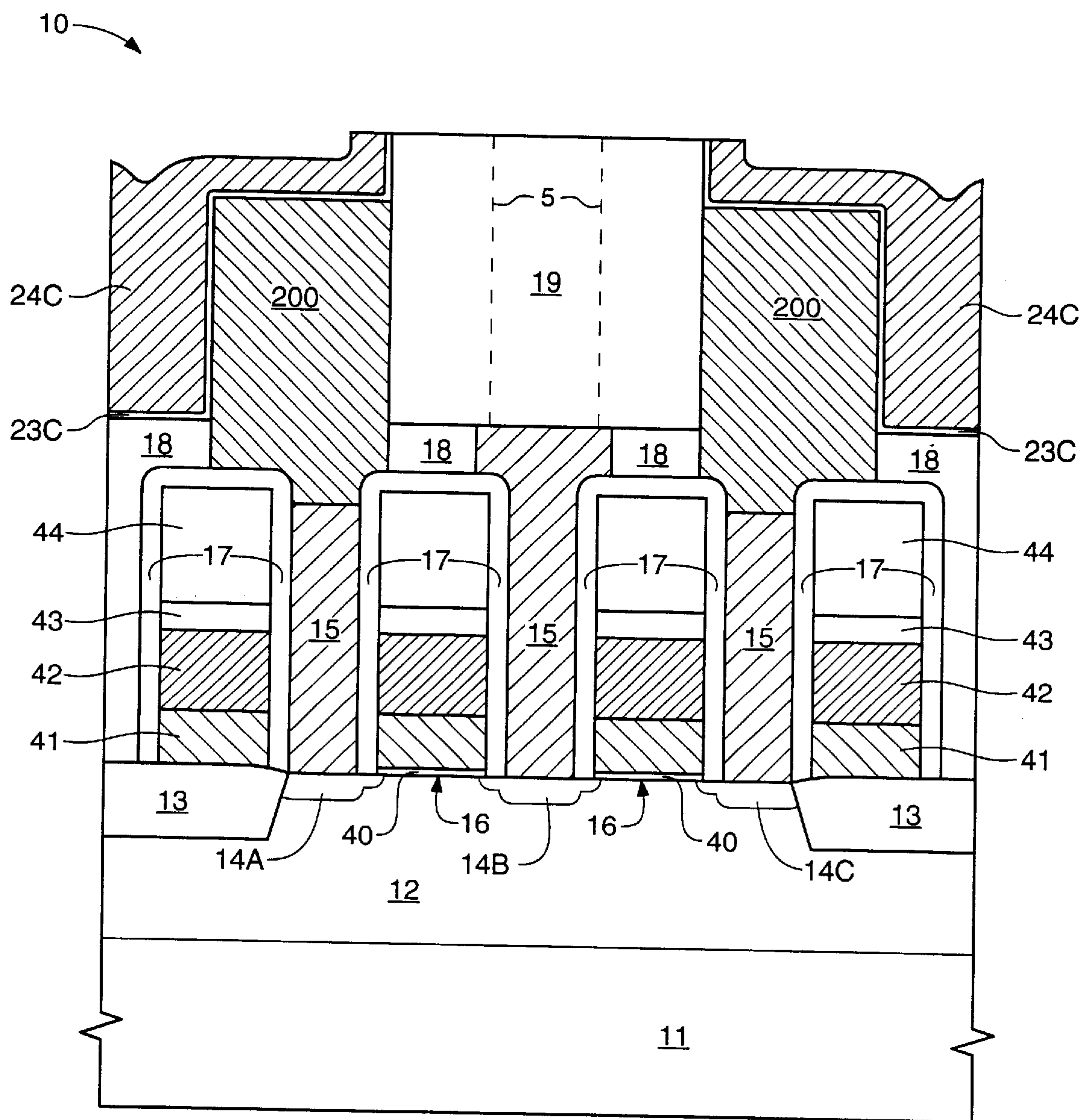
FIG. 16G
