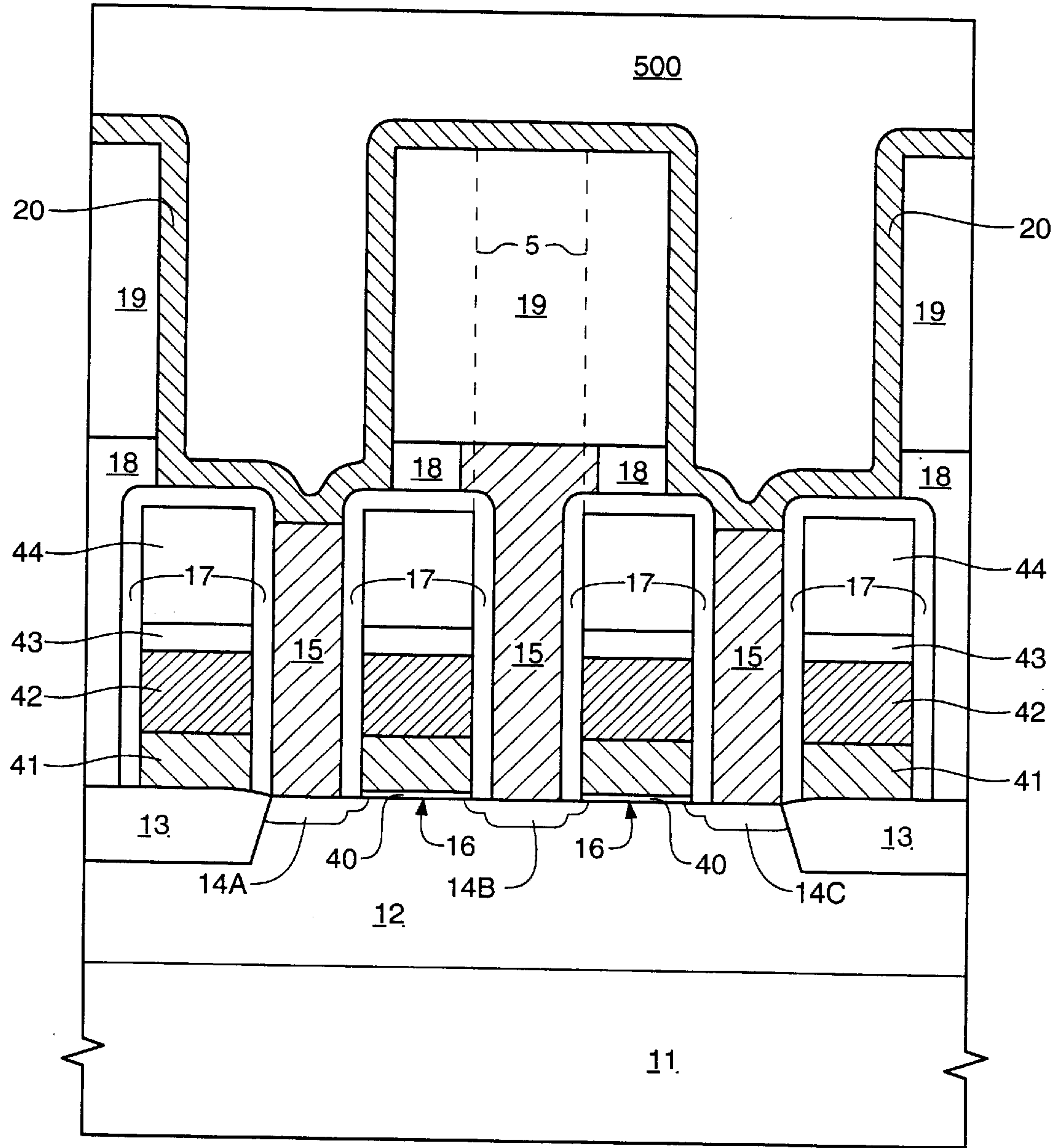
FIG. 17B
