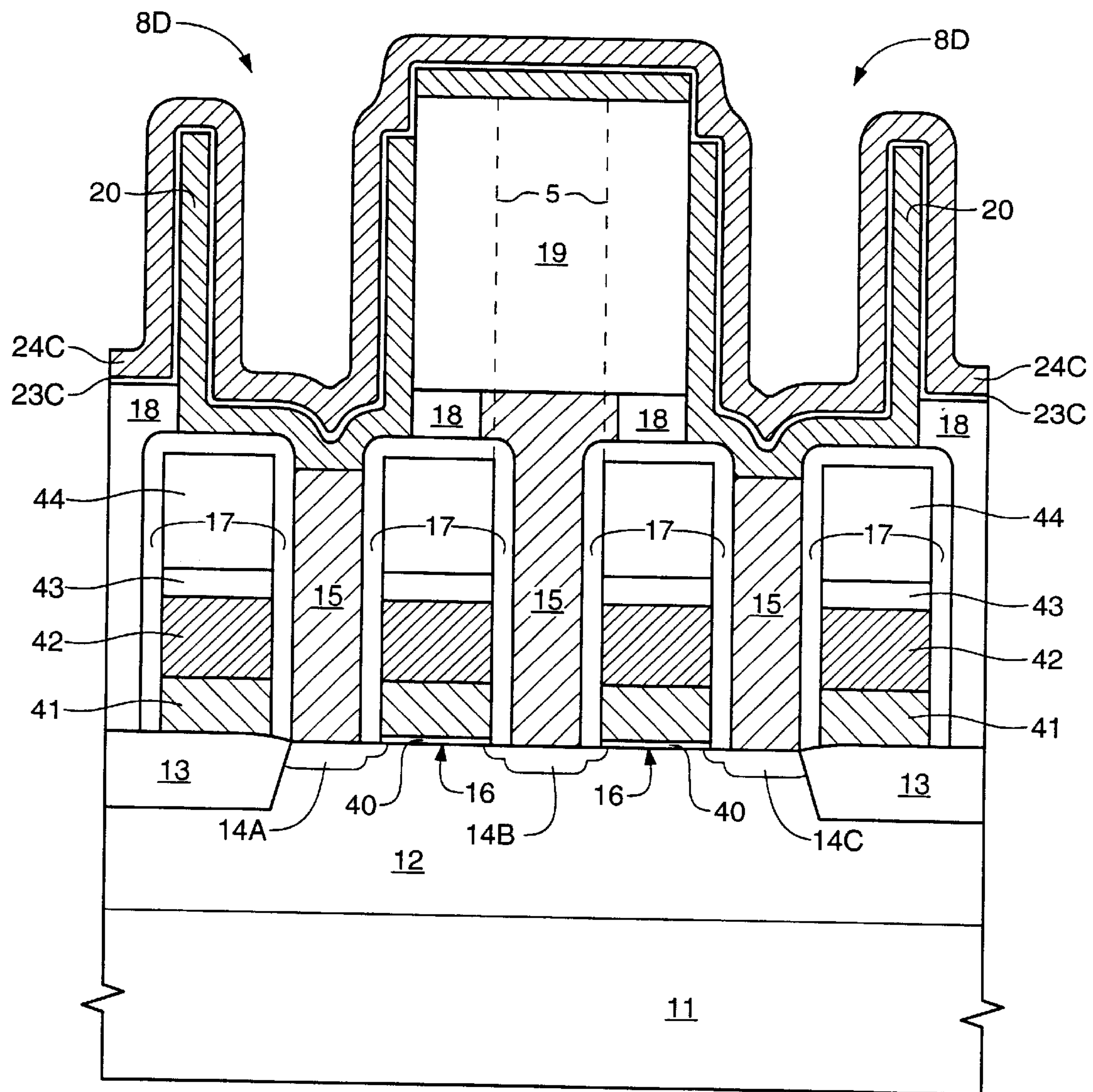
FIG. 17F
