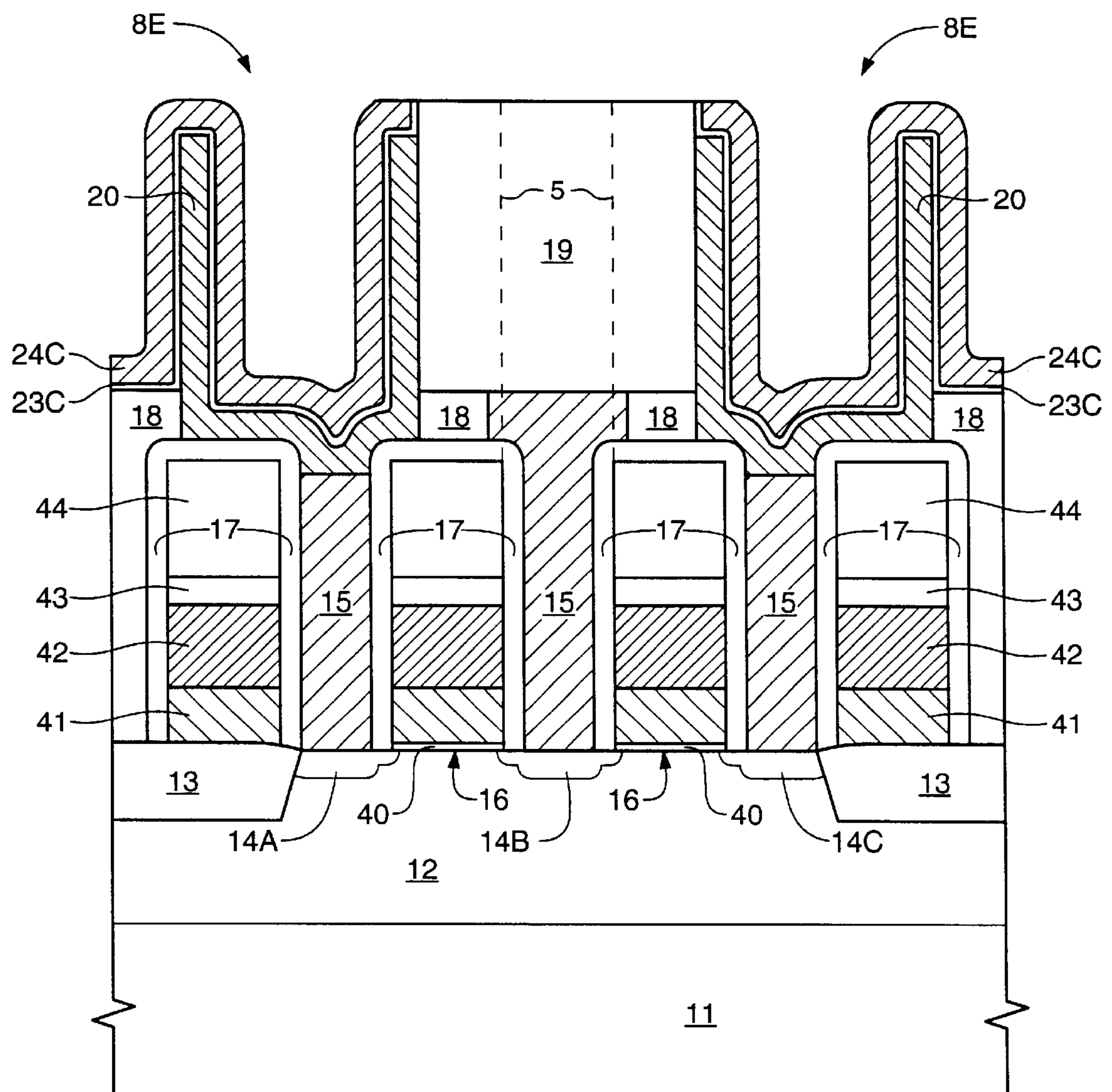
FIG. 18G
