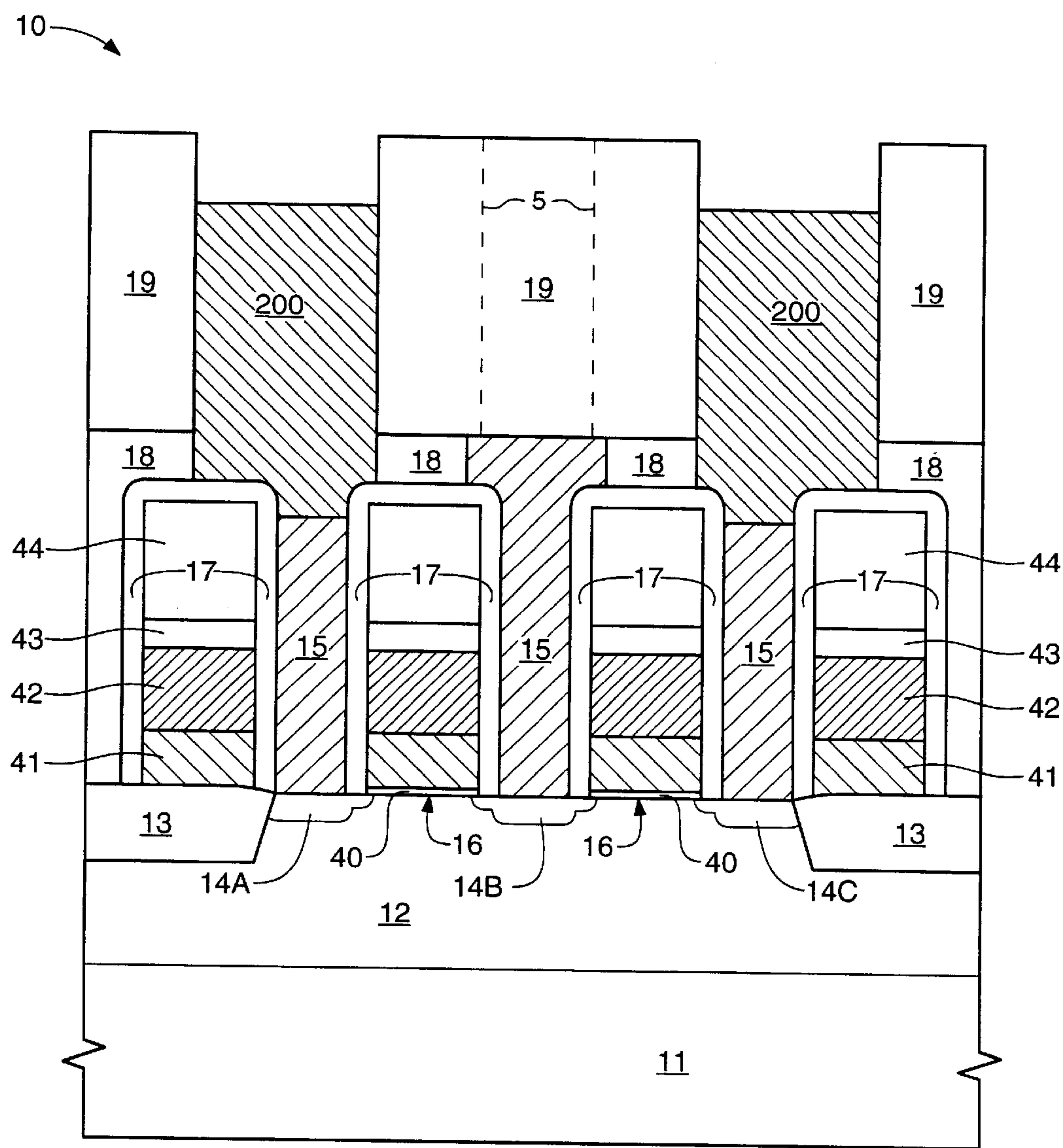
FIG. 16B
