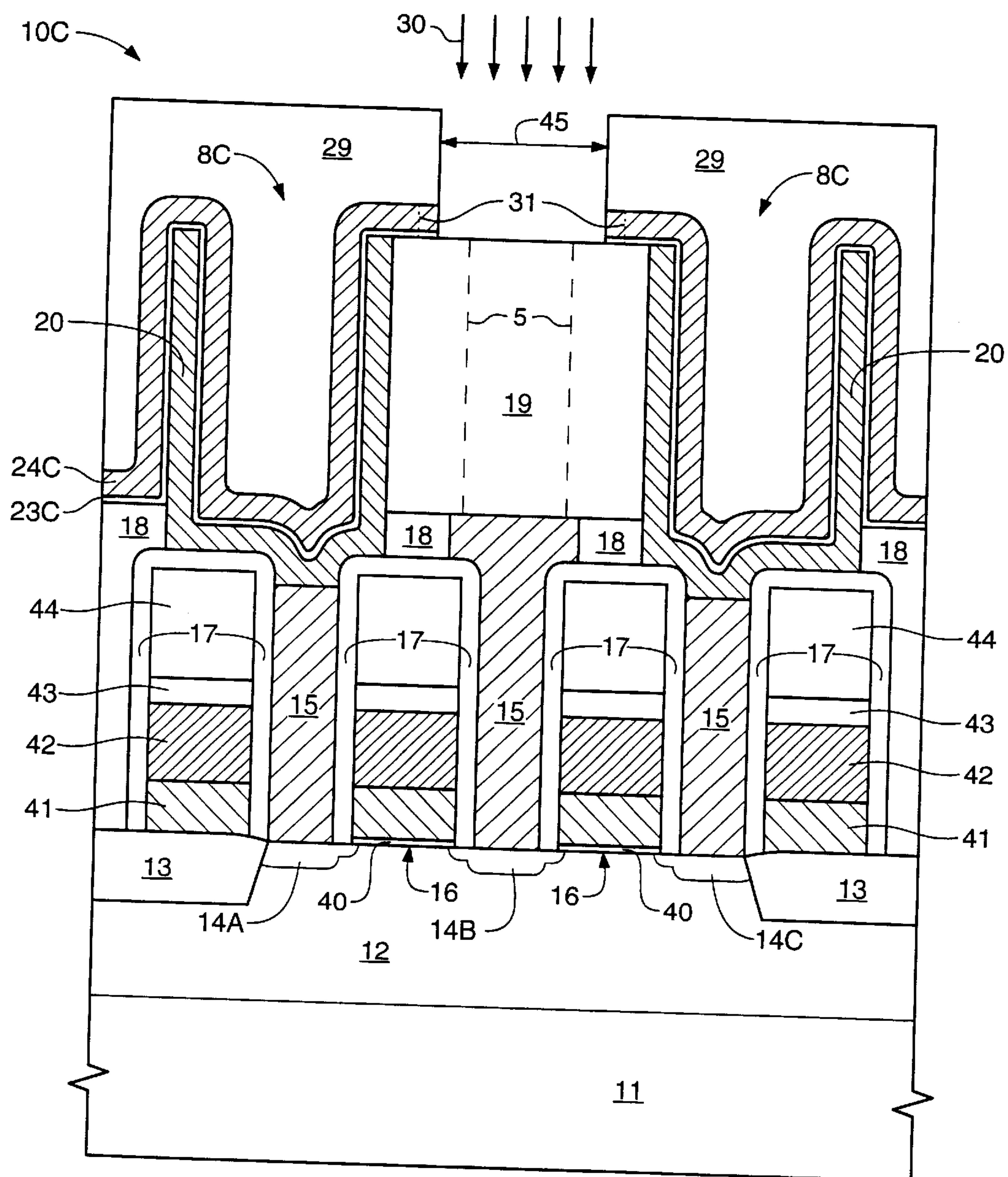
FIG. 9A
