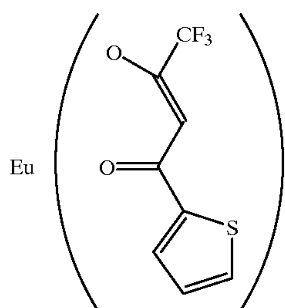
Eu(TTA) 3
