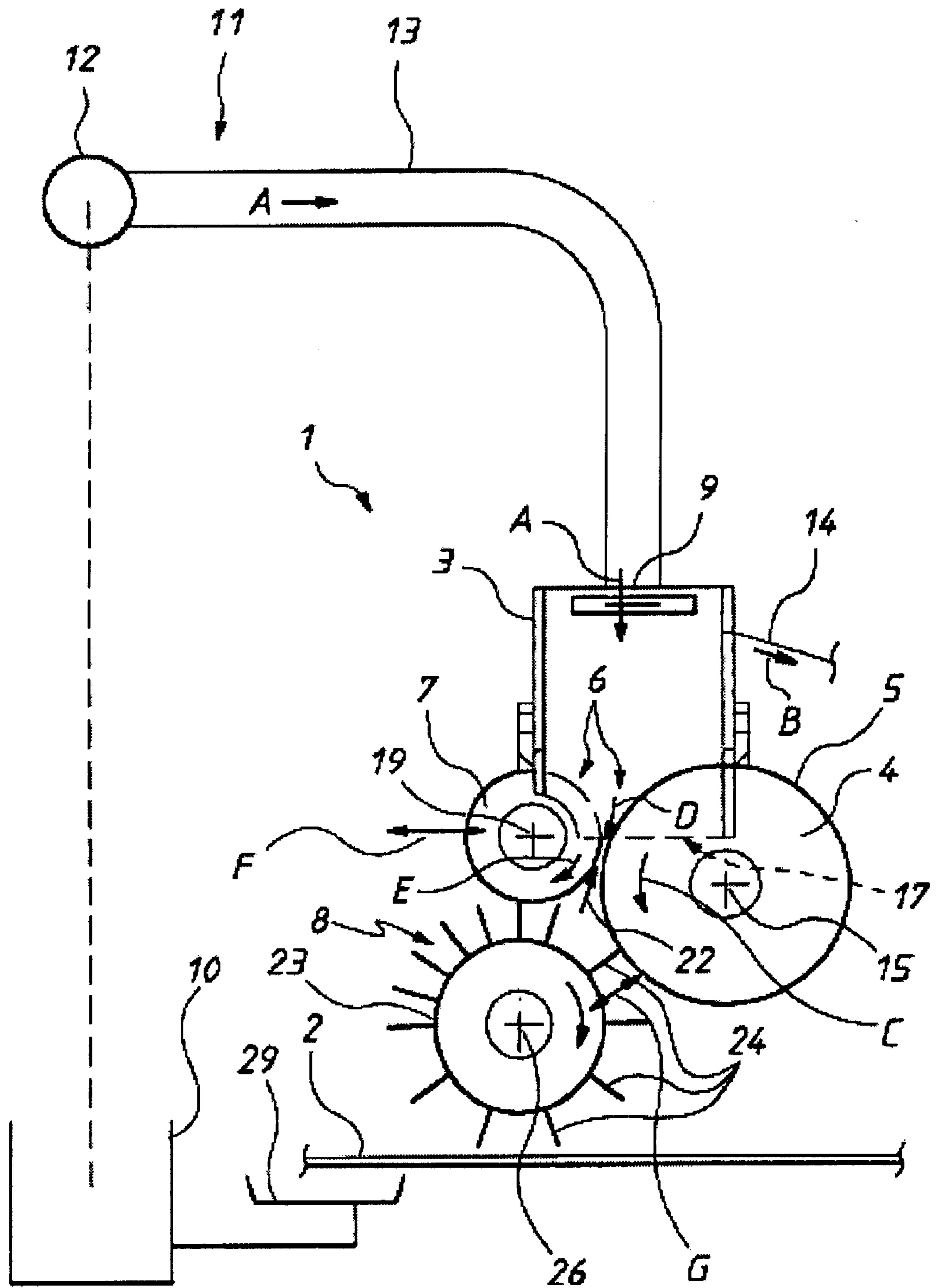
FIG. 3
