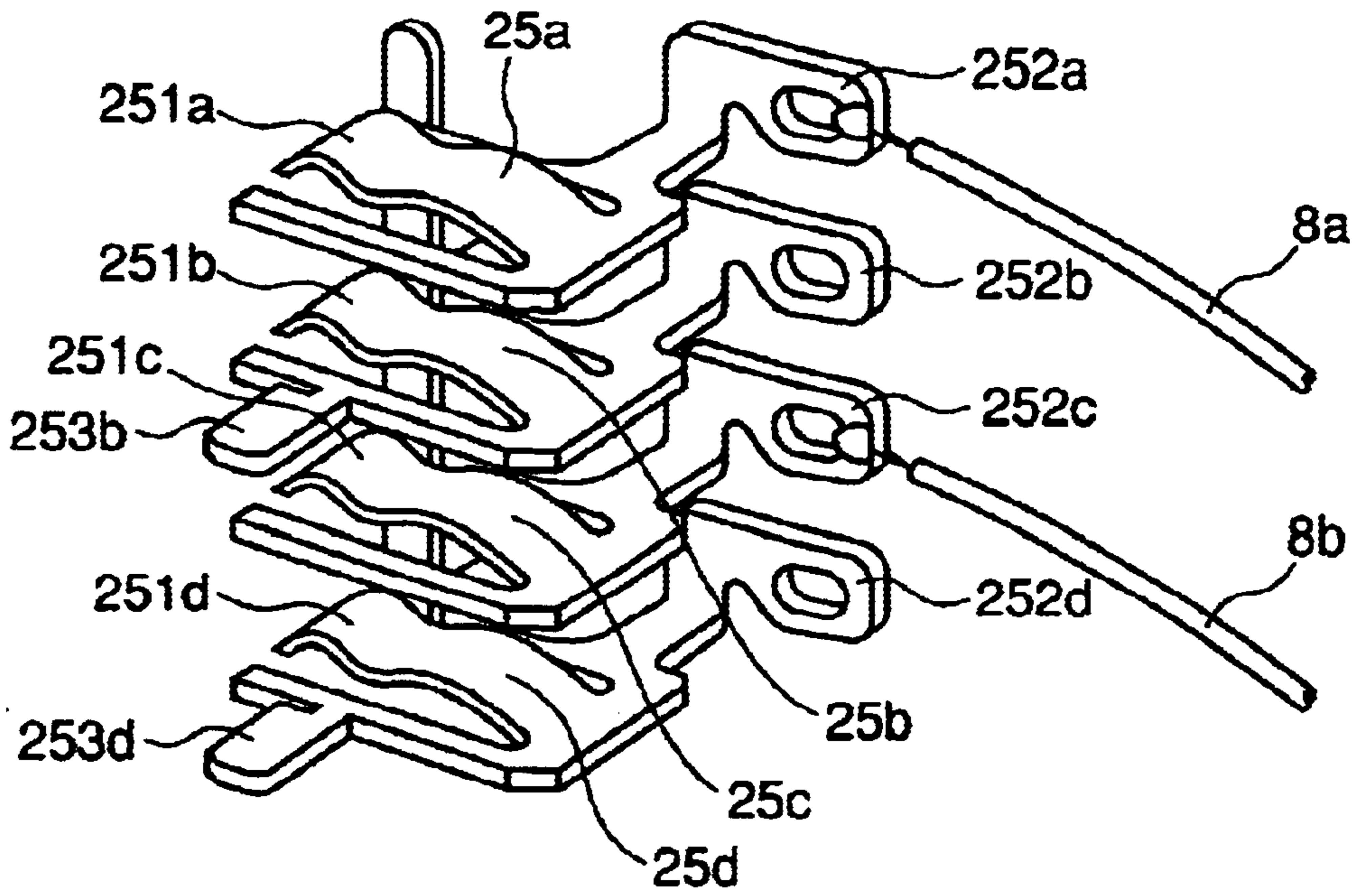
FIG. 9A
