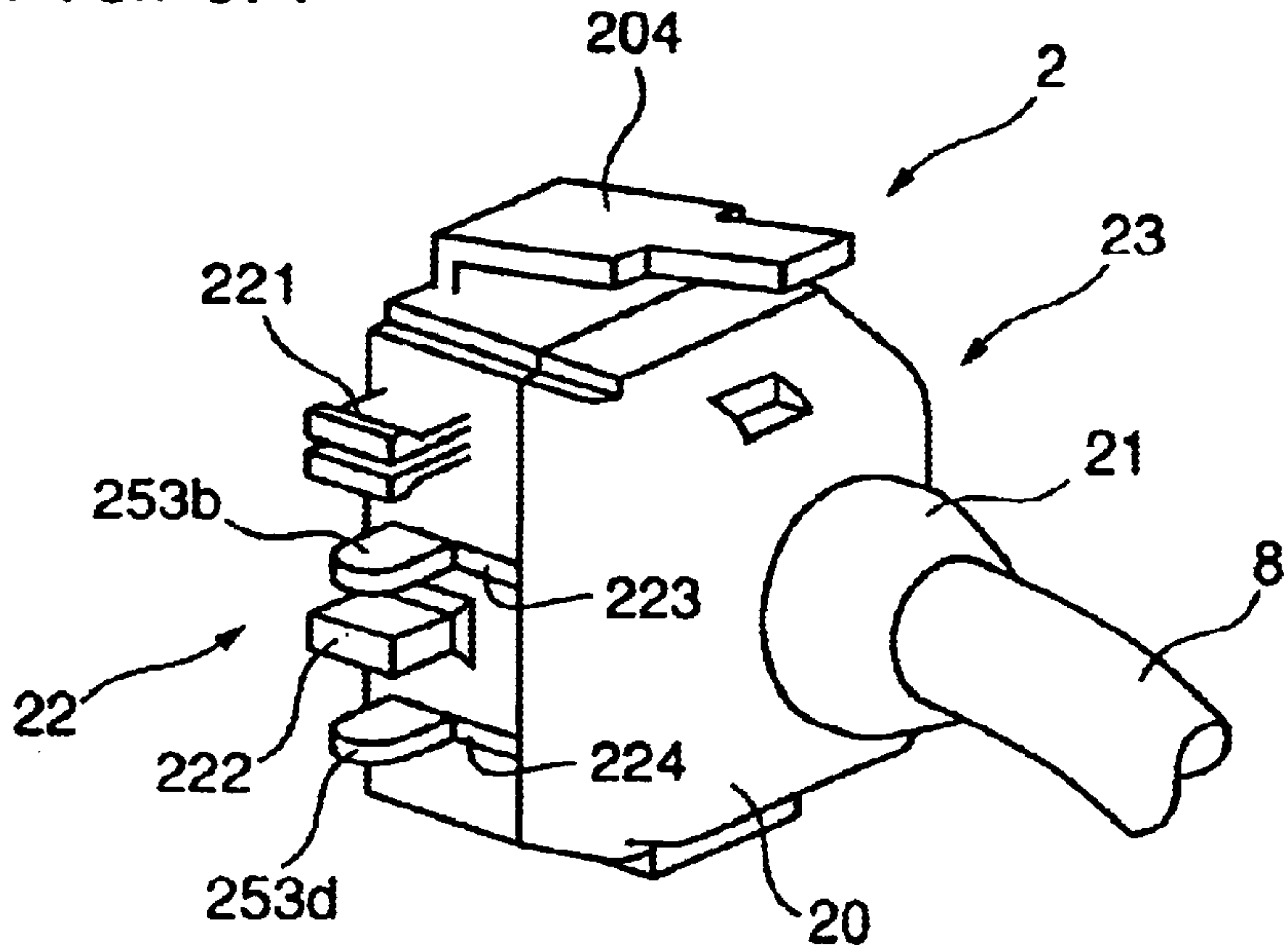
FIG. 5A
