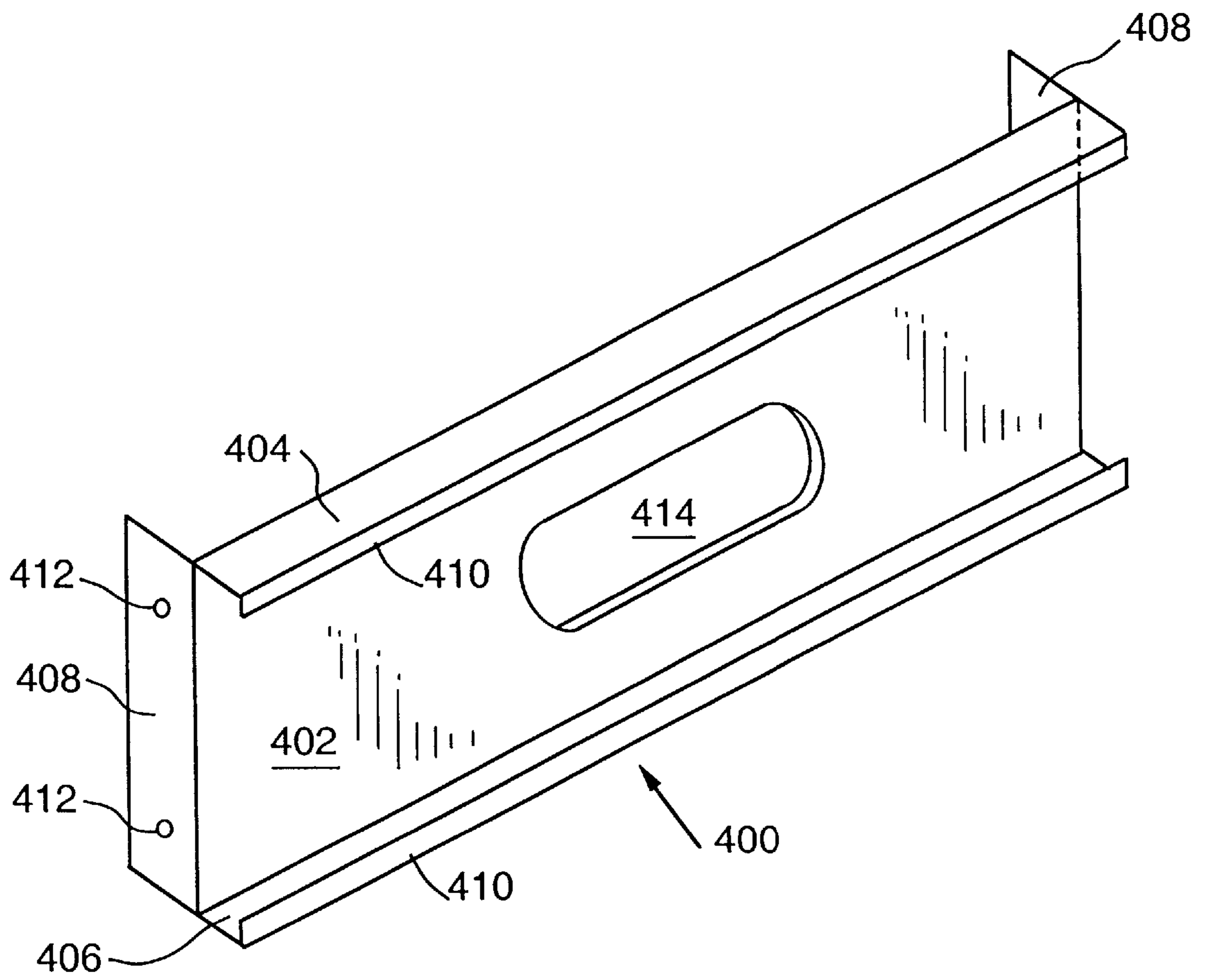
FIG. 12
