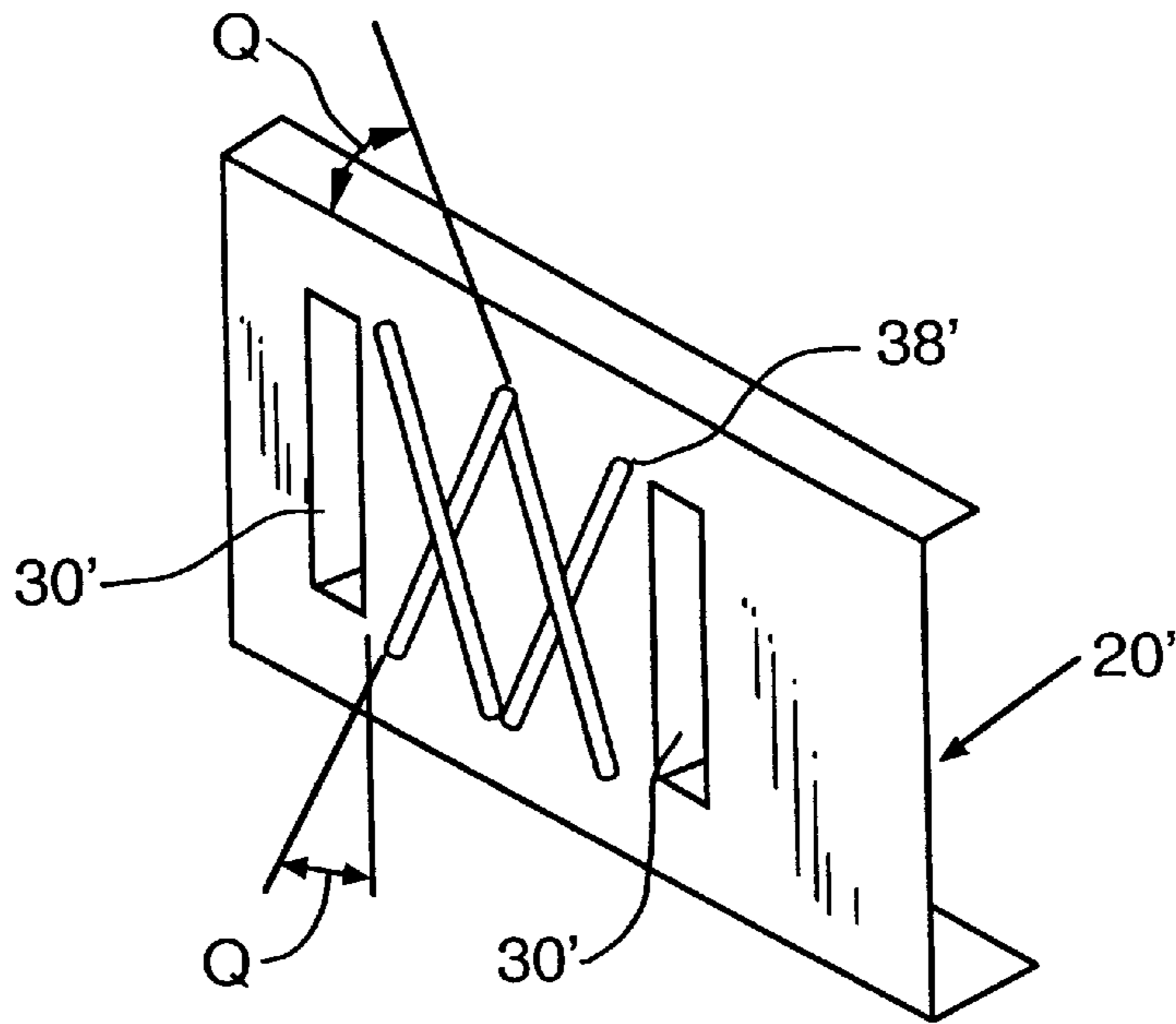
FIG. 4a
