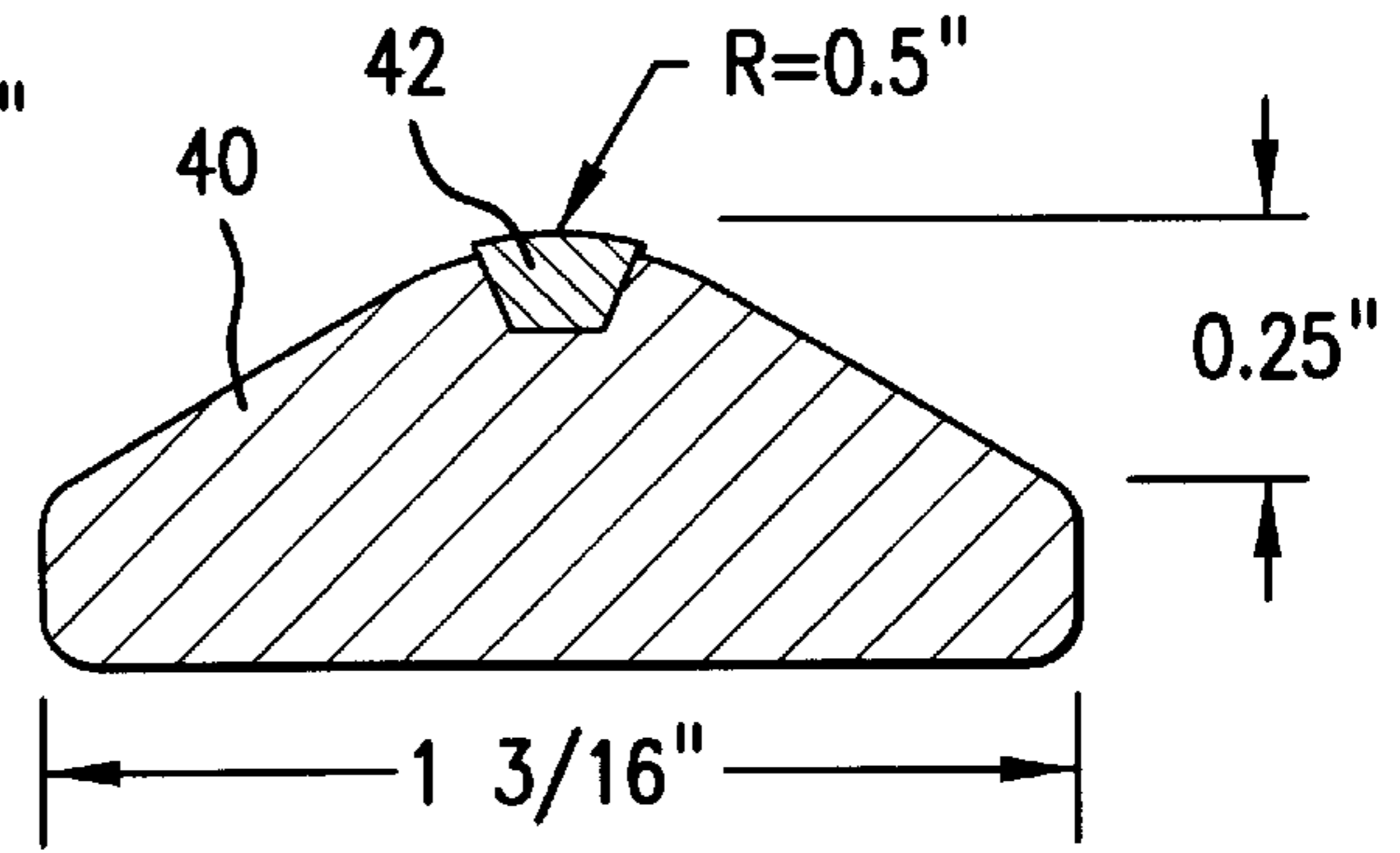
ANODE FIG. 7D
