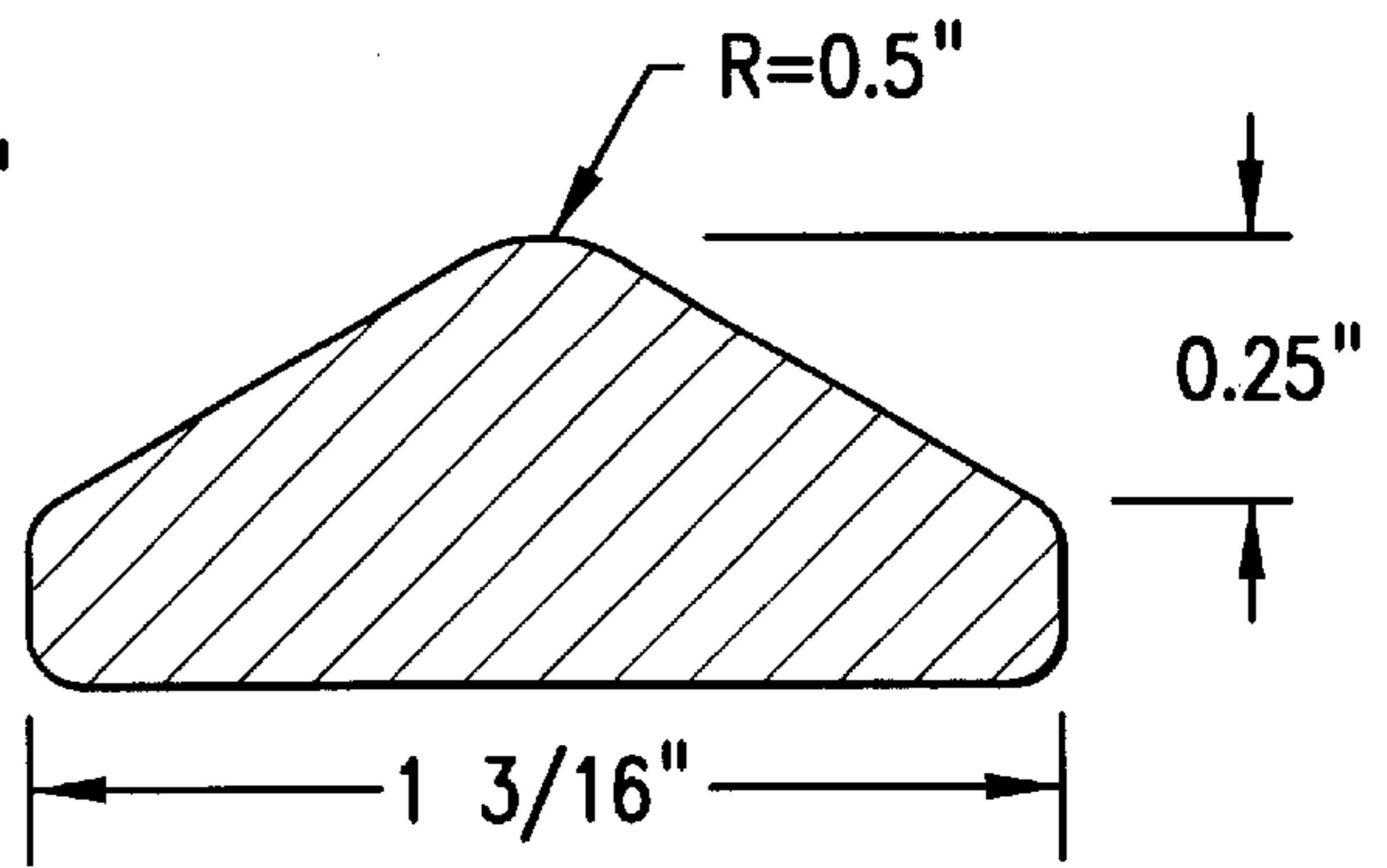
ANODE FIG. 7B
