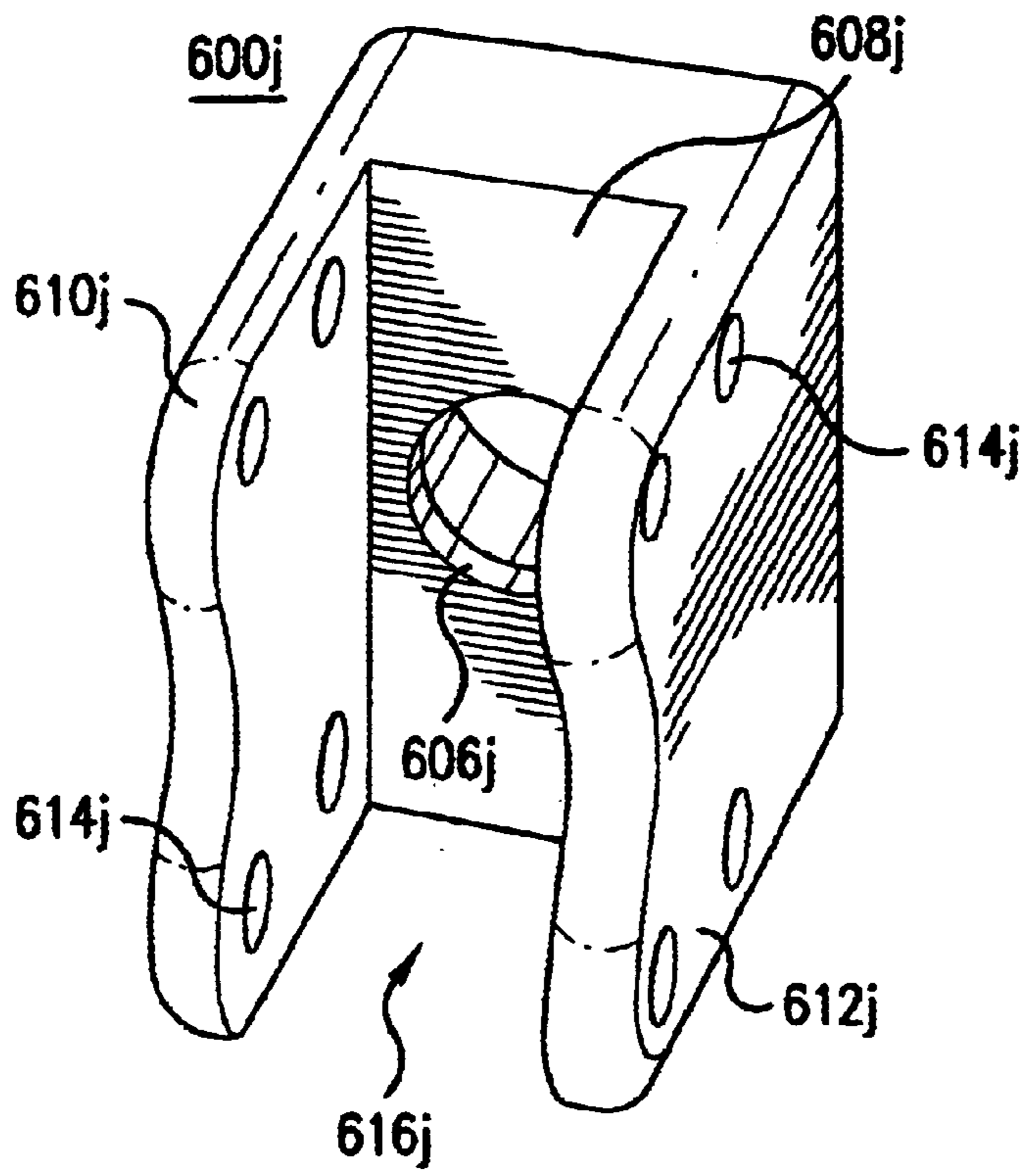
FIG. 51
