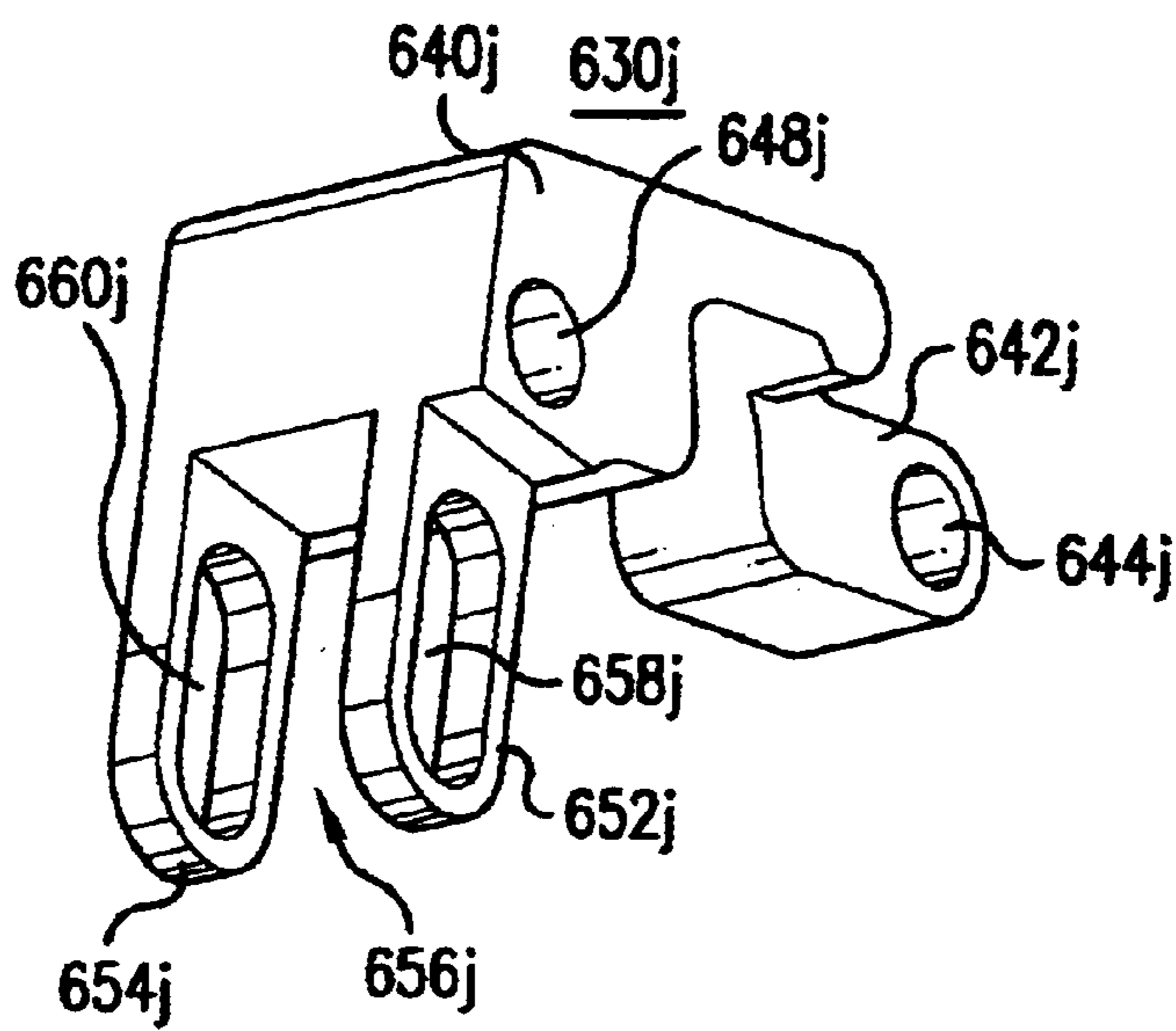
FIG. 52
