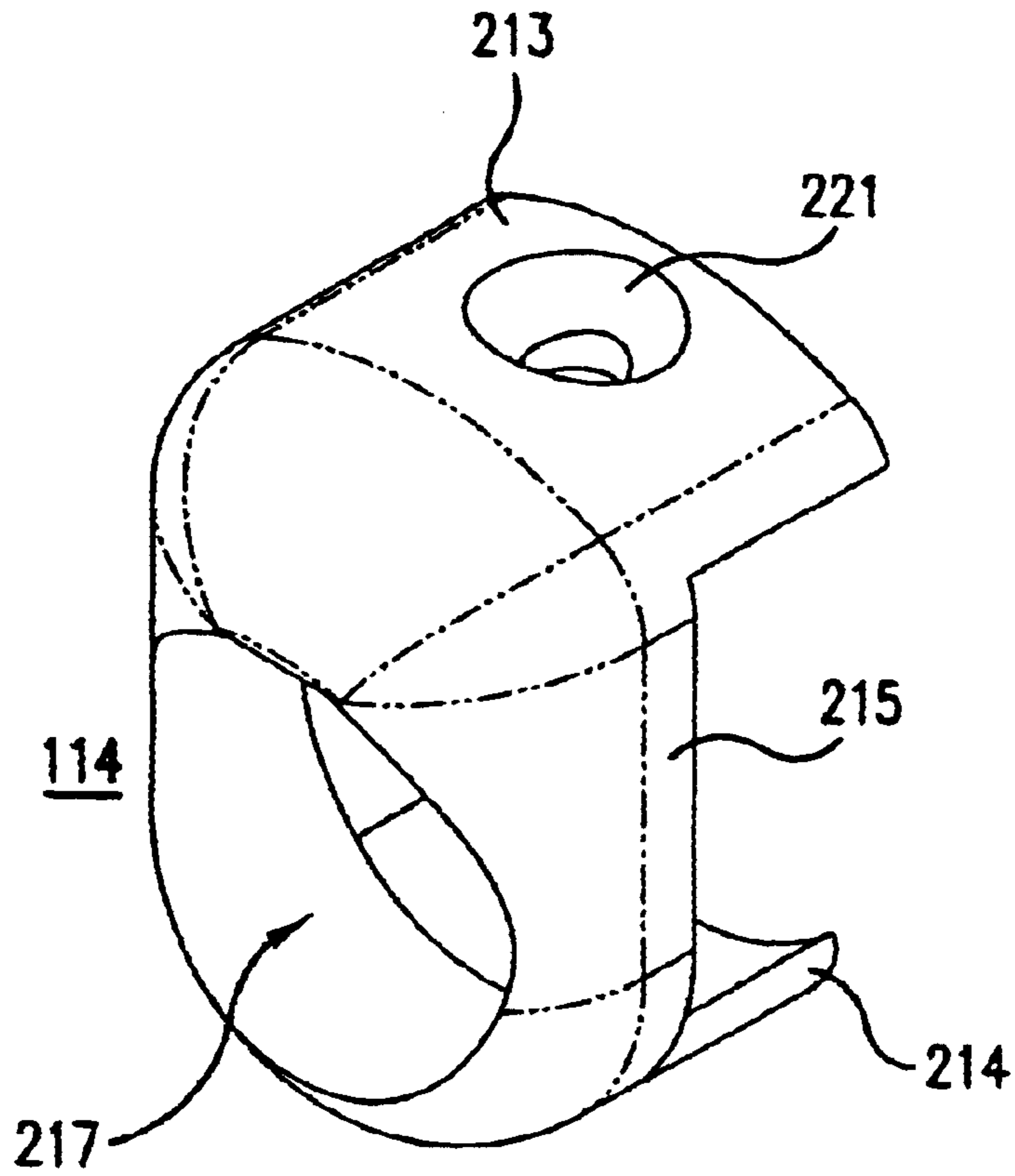
FIG. 23
