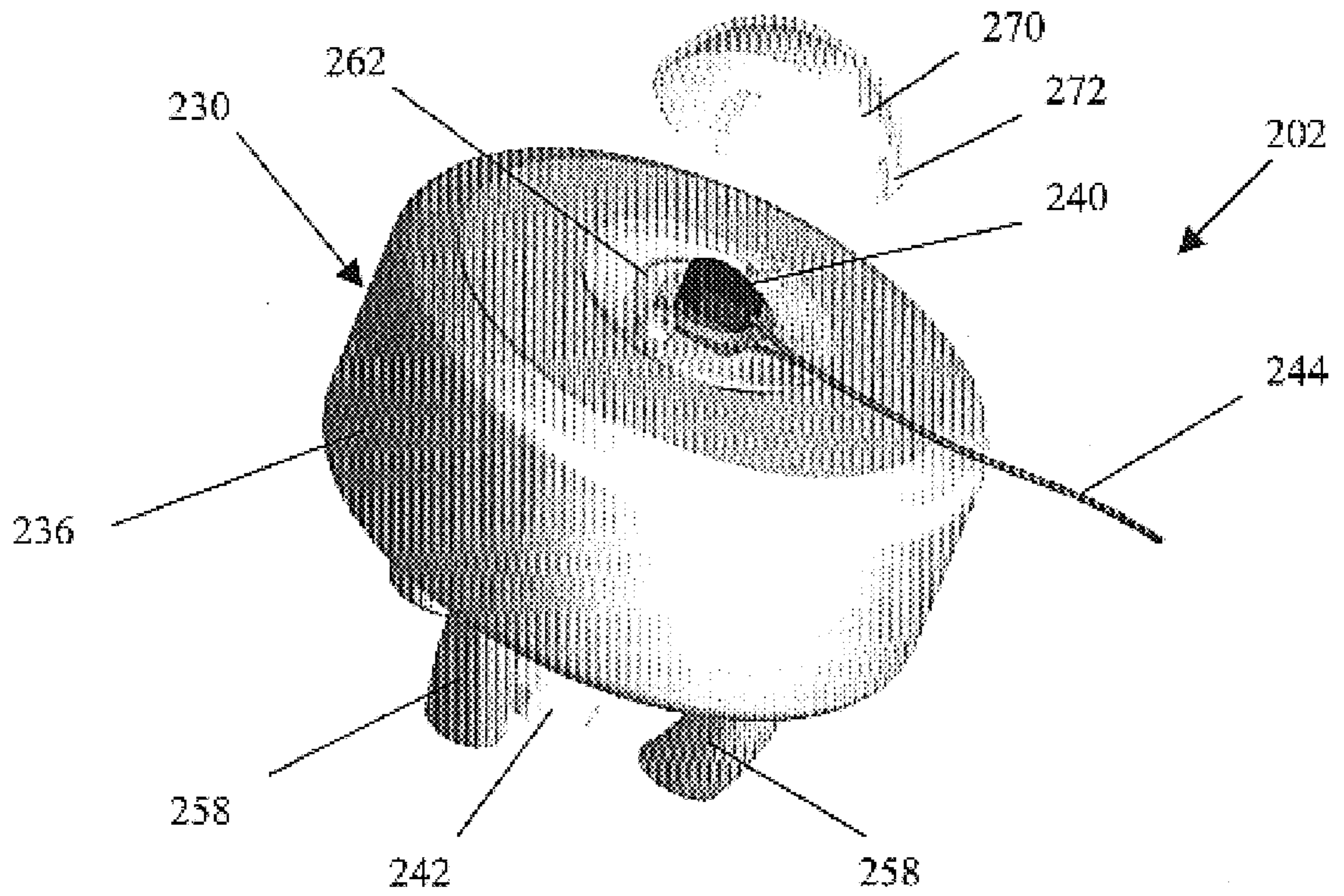
FIG. 4A
