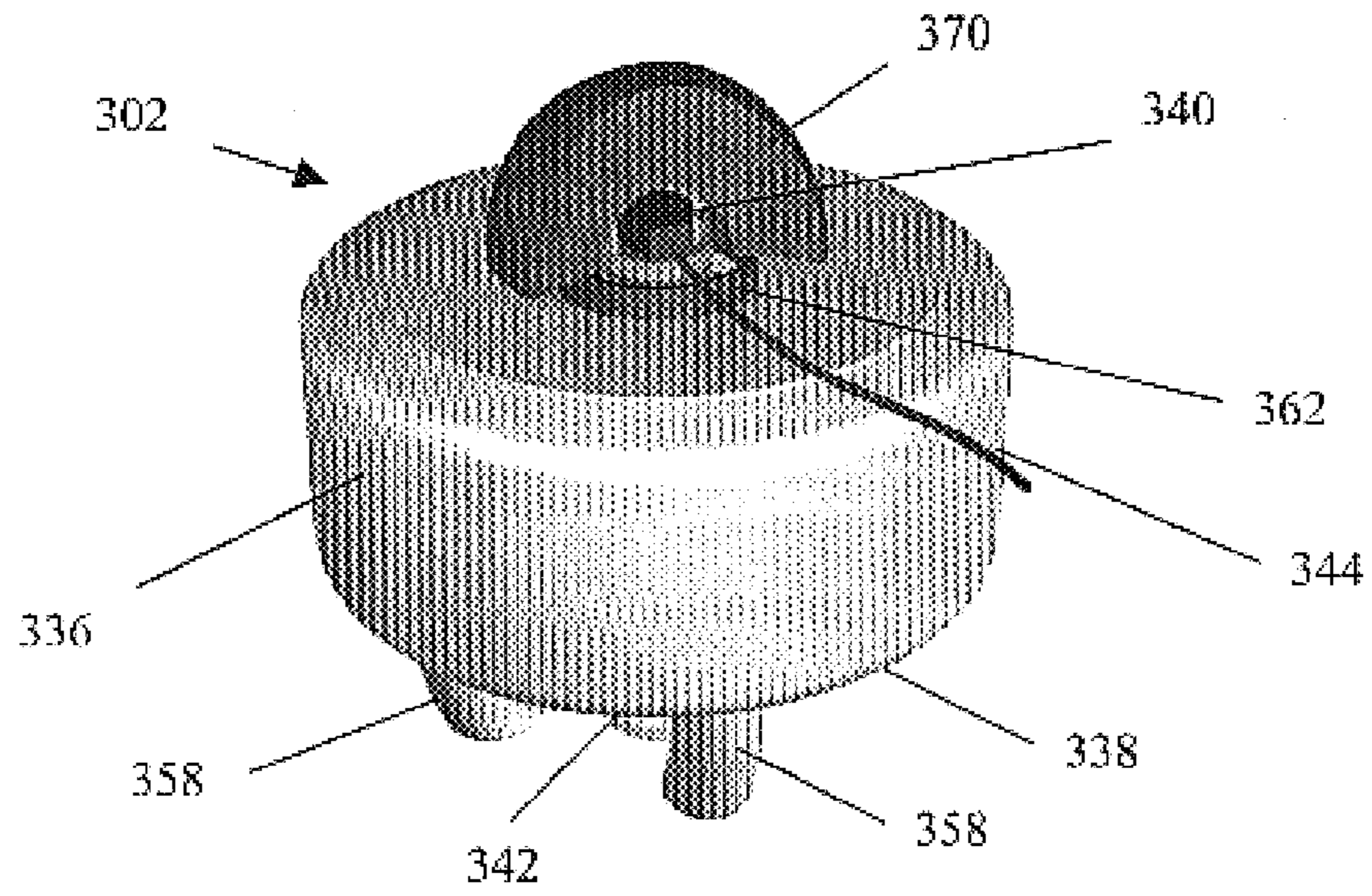
FIG. 5A
