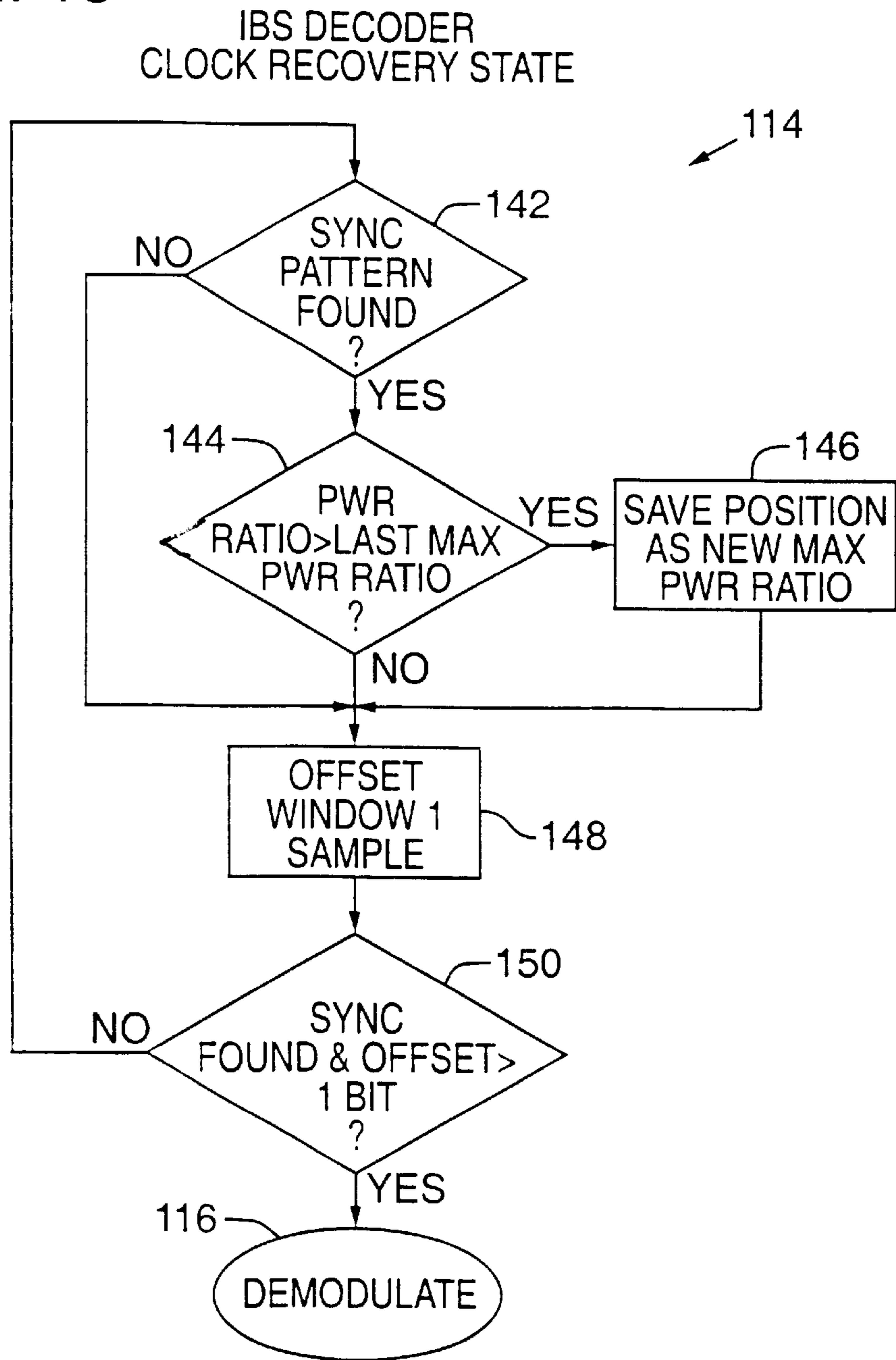
FIG. 13
