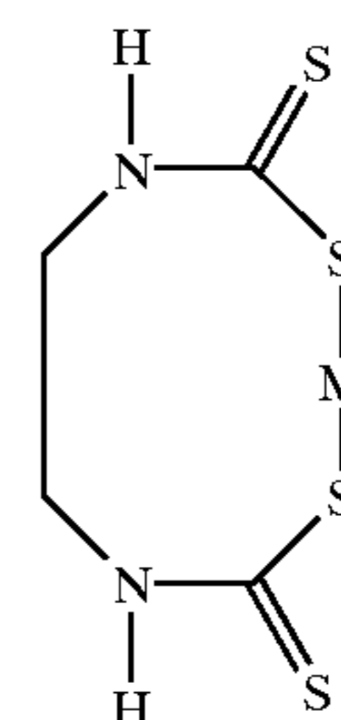
M = Zn (ZINEB)
