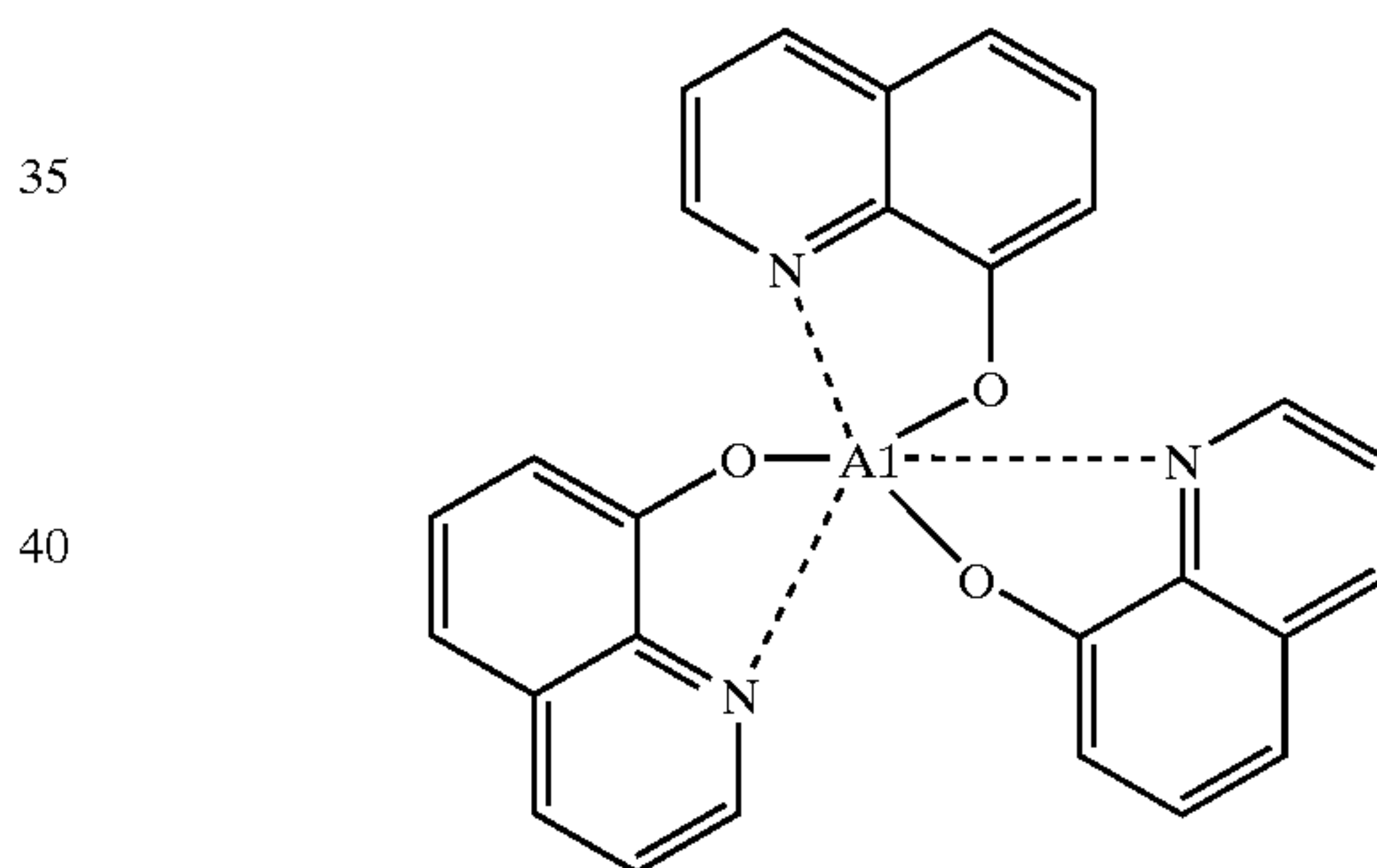
Alq 3 :
