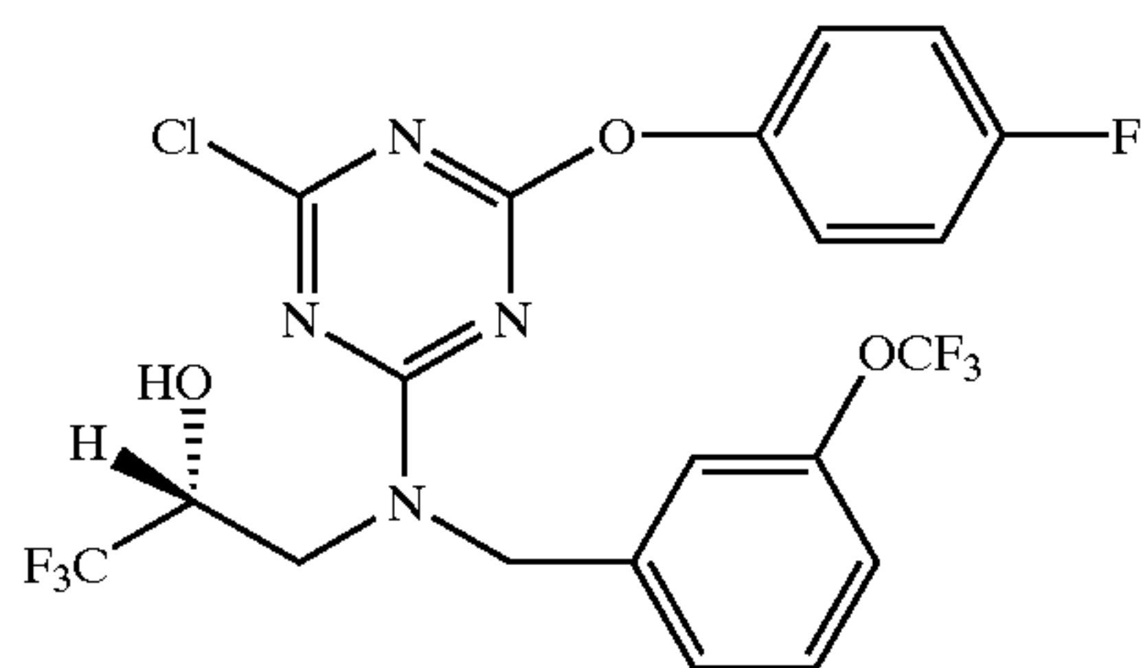
(2R)-N-[2-chloro-6-(p-fluorophenoxy)-1,3,5-triazin-4-yl]-3-[[[3-(trifluoromethoxy)phenyl]methyl]amino]-1,1,1-trifluoro-2-propanol
