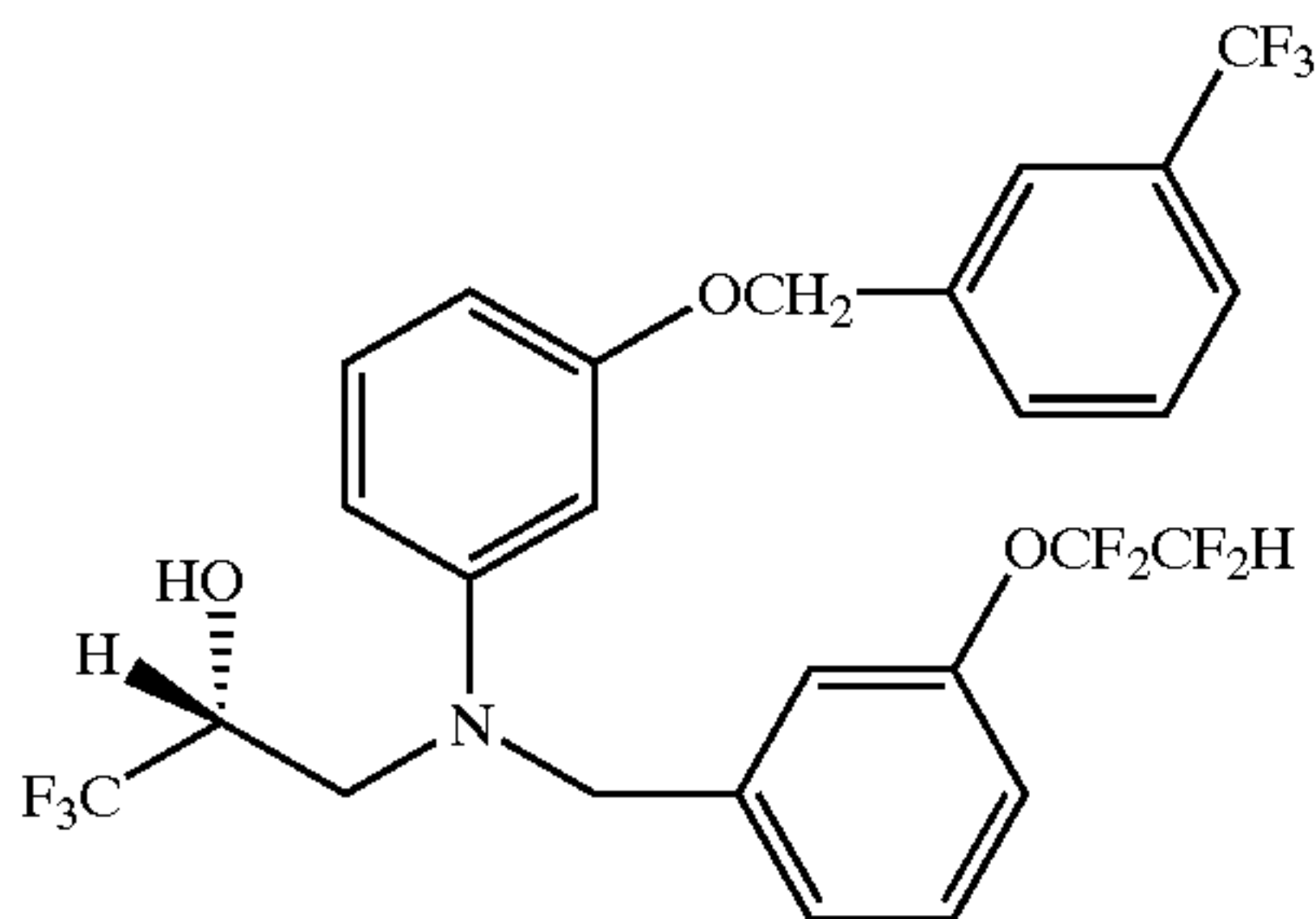
(2R)-3-[[[3-(1,1,2,2-tetrafluoroethoxy)phenyl]methyl][3-[[3-(trifluoromethyl)-phenyl]methoxy]phenyl]amino]-1,1,1-trifluoro-2-propanol
