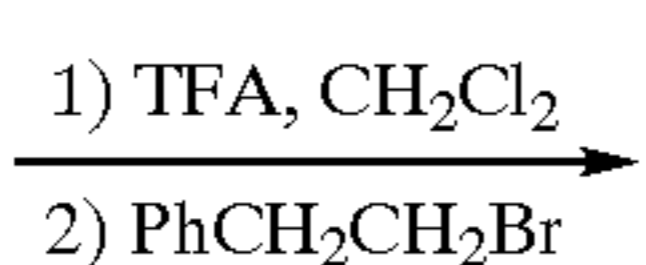
198 single enantiomer
