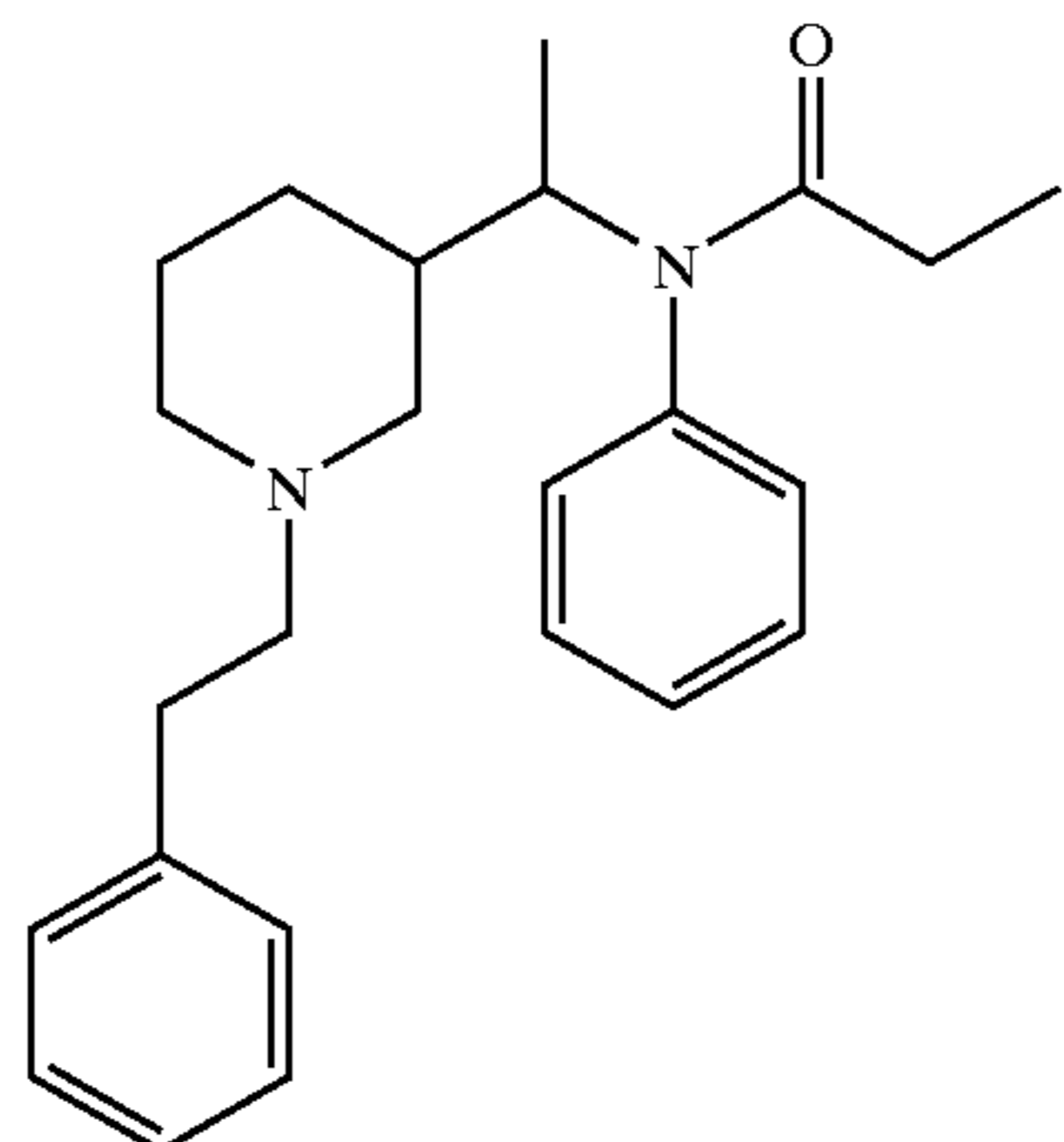
195 single enantiomer
