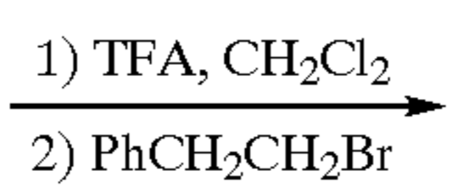
196 single enantiomer
