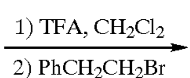
197 single enantiomer
