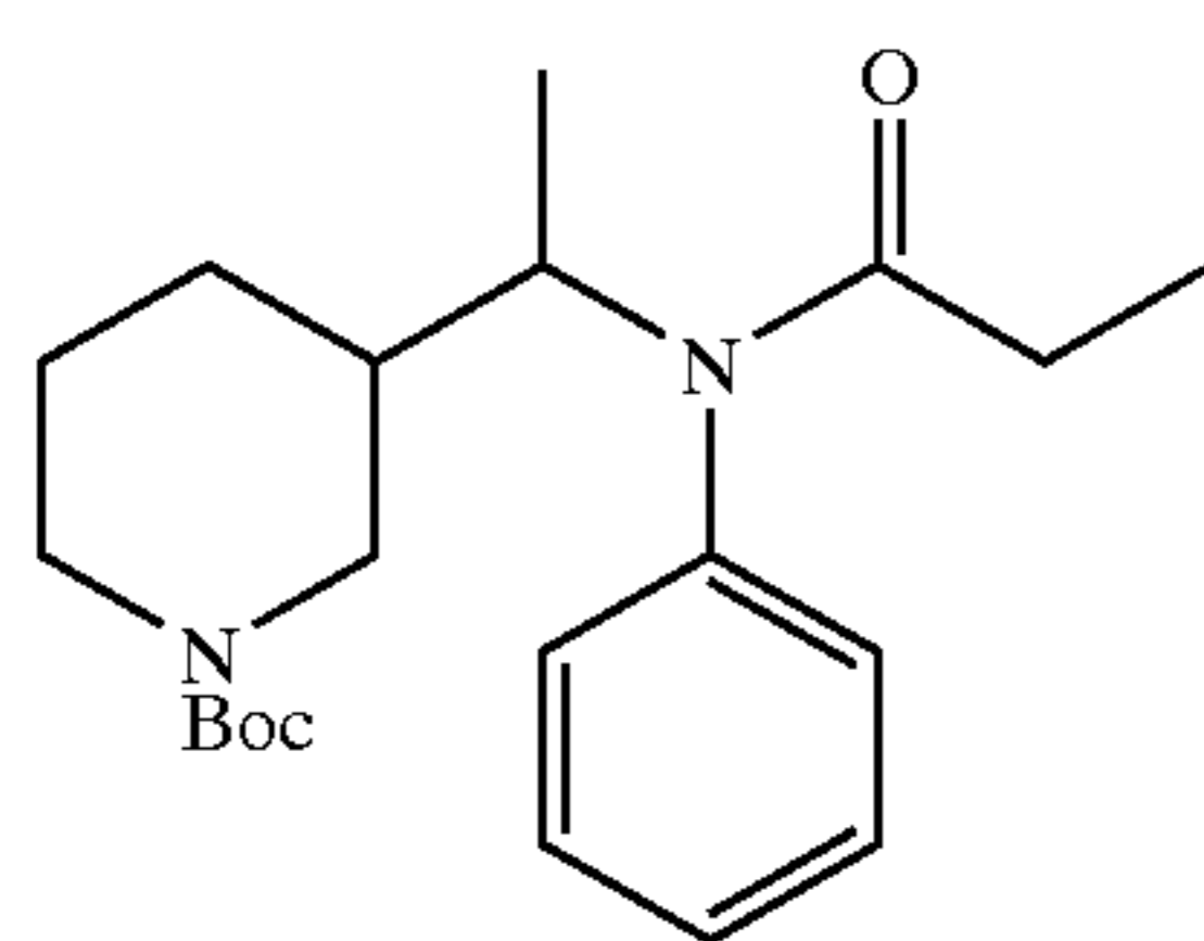
191 single enantiomer
