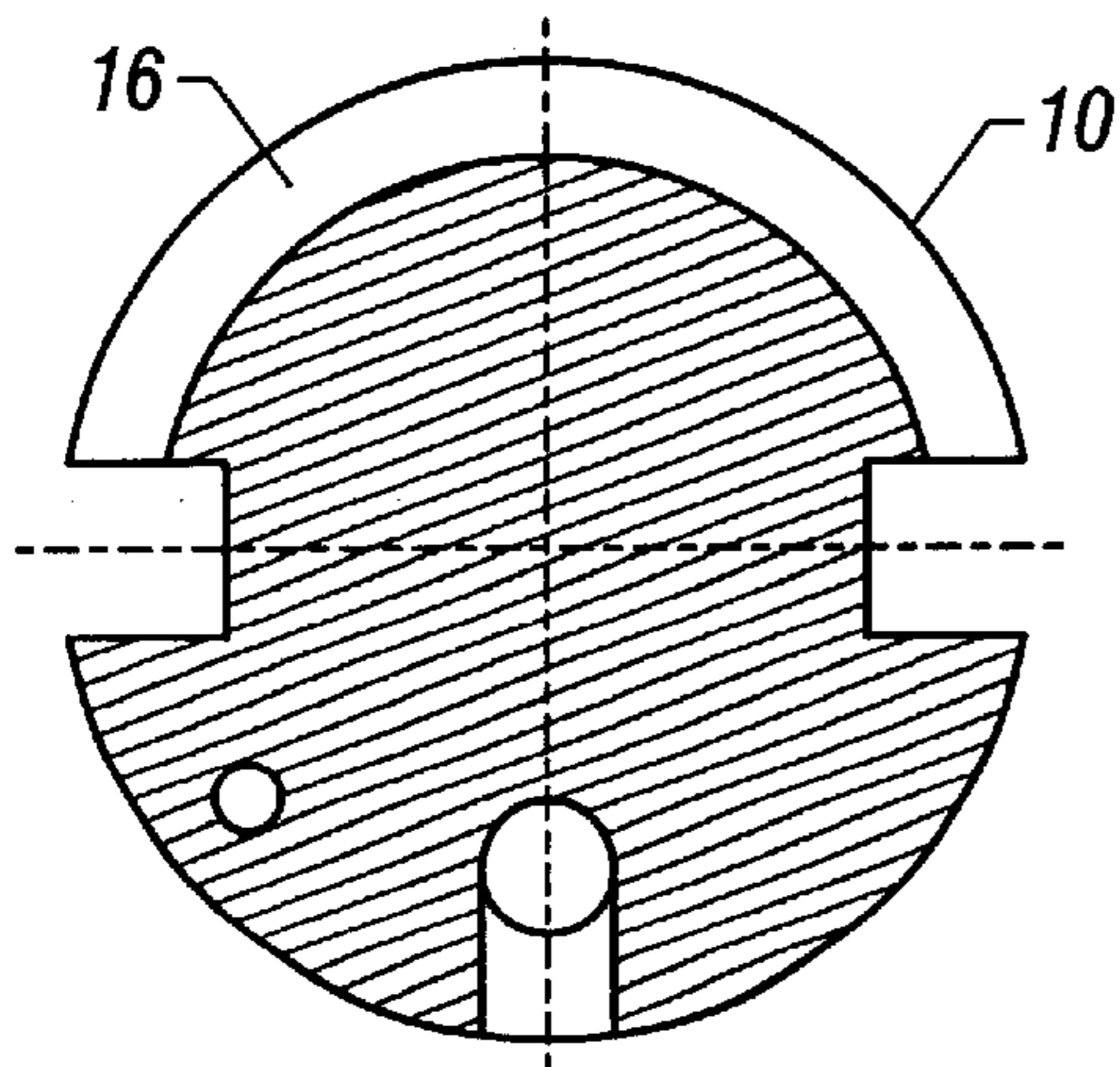
SECTION D-D
