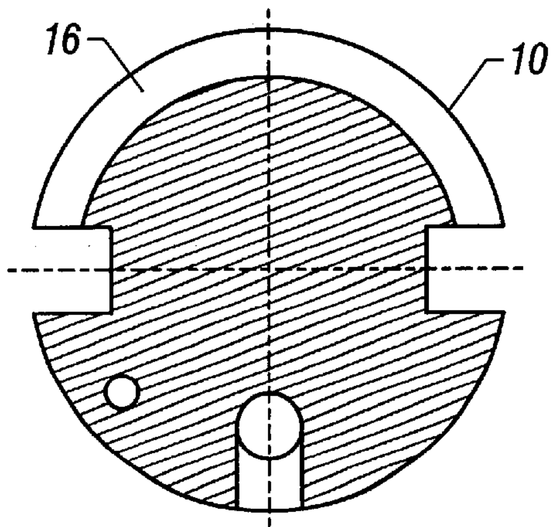
SECTION D-D
