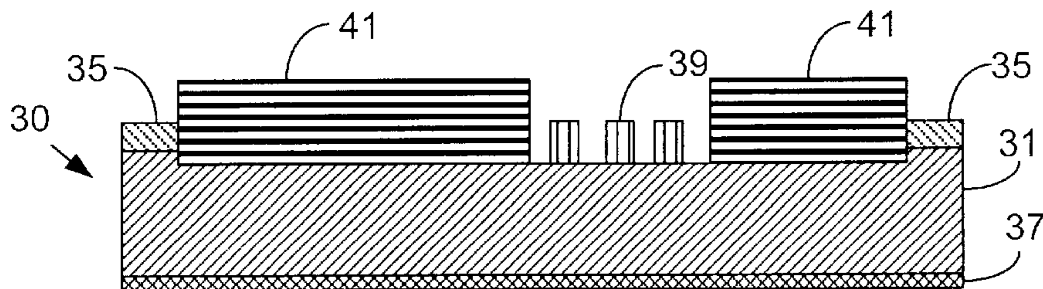
FIG. 2B
