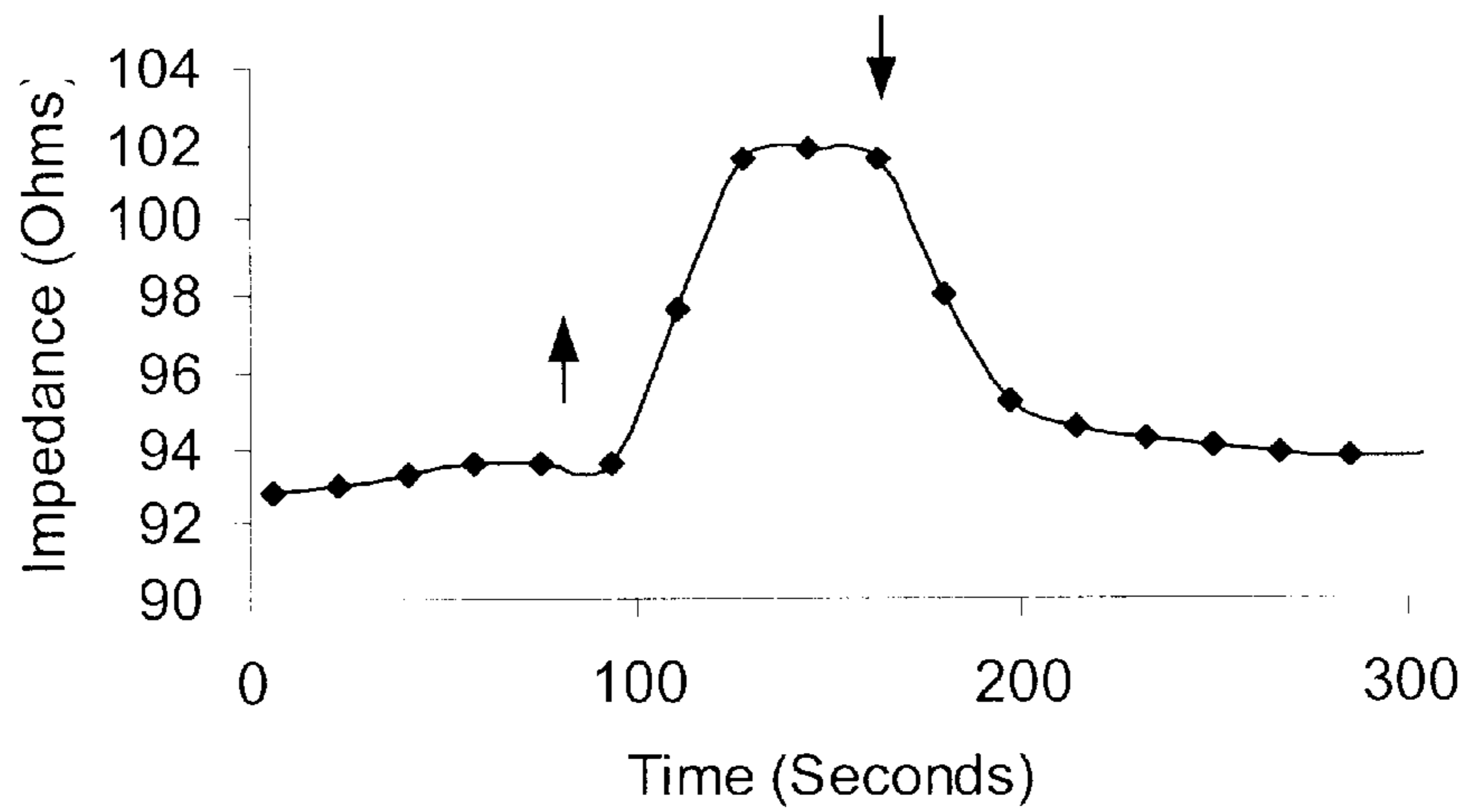
FIG. 4C
