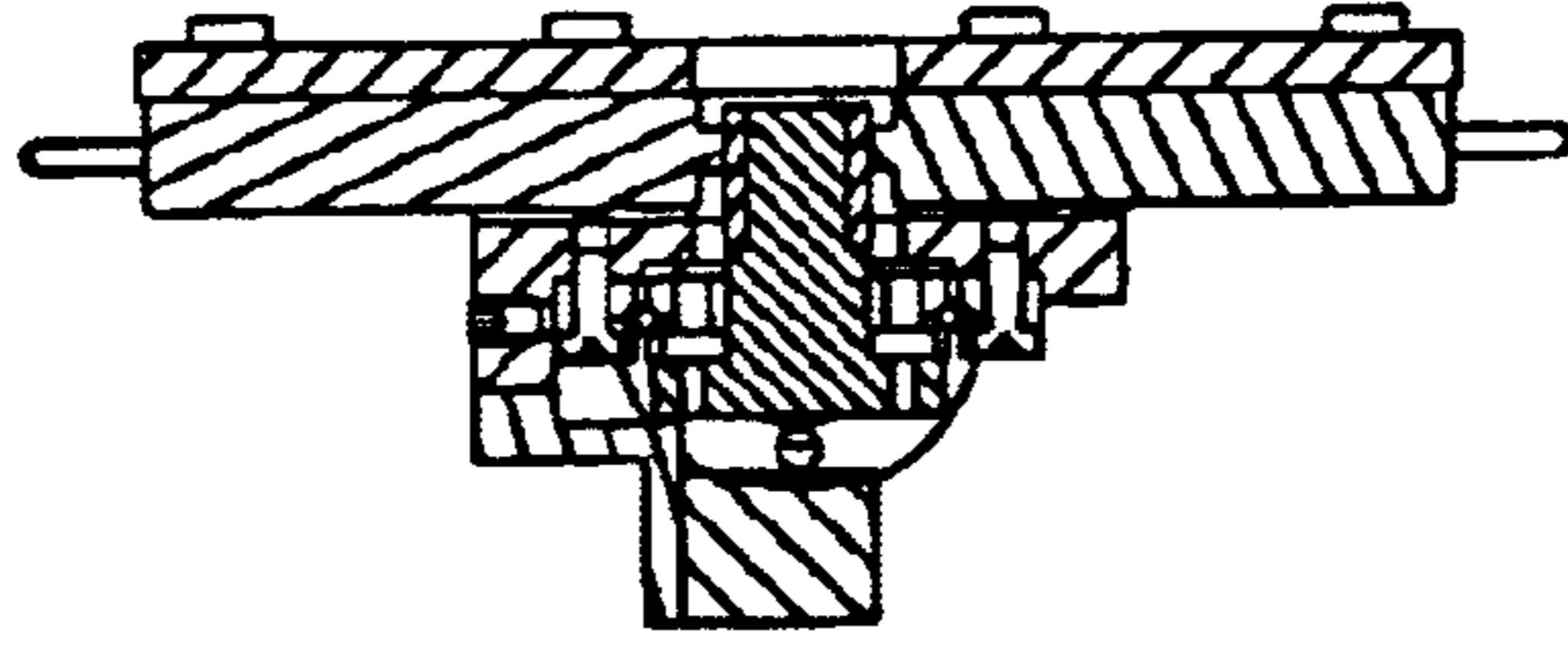
SECTION A-A
