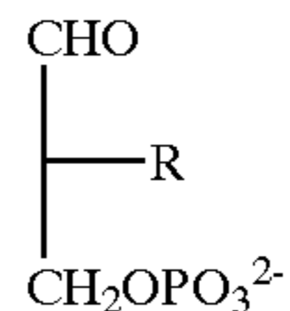
17 - R = I 18 - R = F 19 - R = SH 20 - R = OMe
