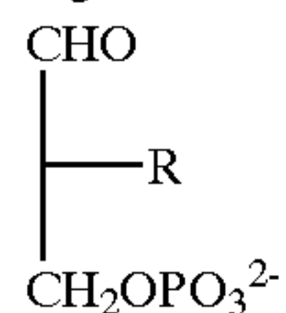
14 - R = F
