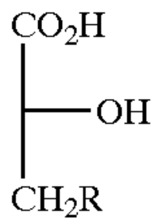
21 - R = I
