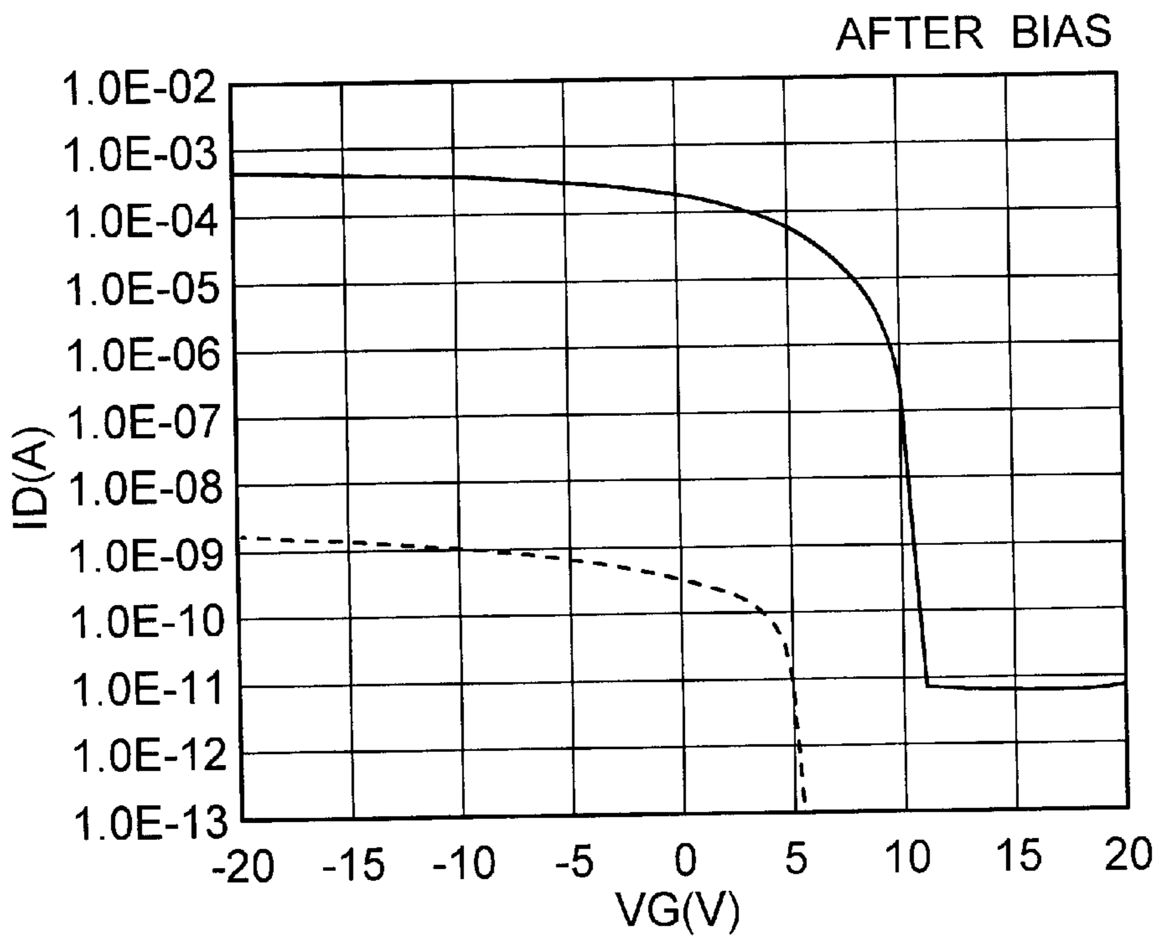
I D vs V G . 20B
