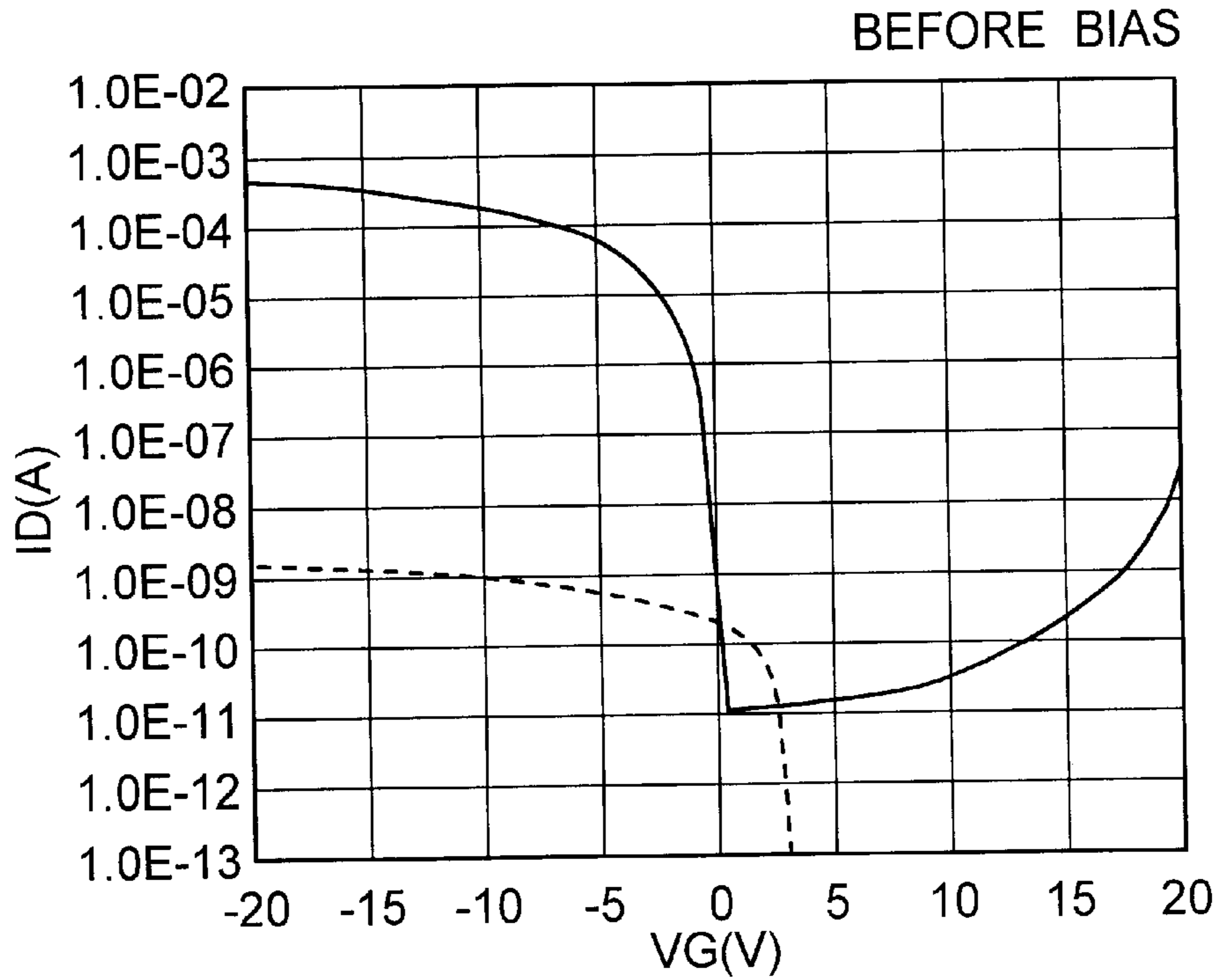
I D vs V G . 20A
