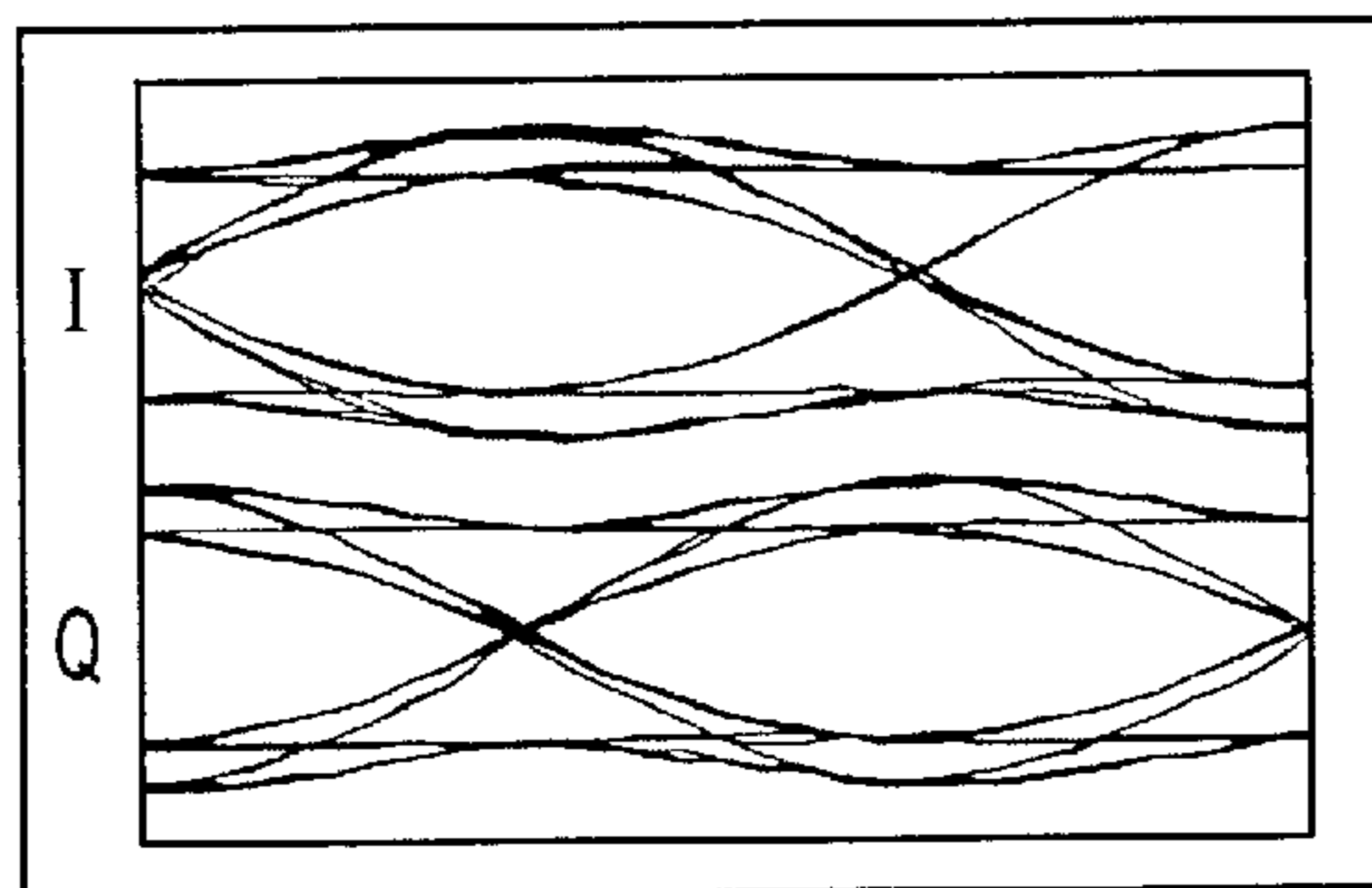
FQPSK-B MEAS.
