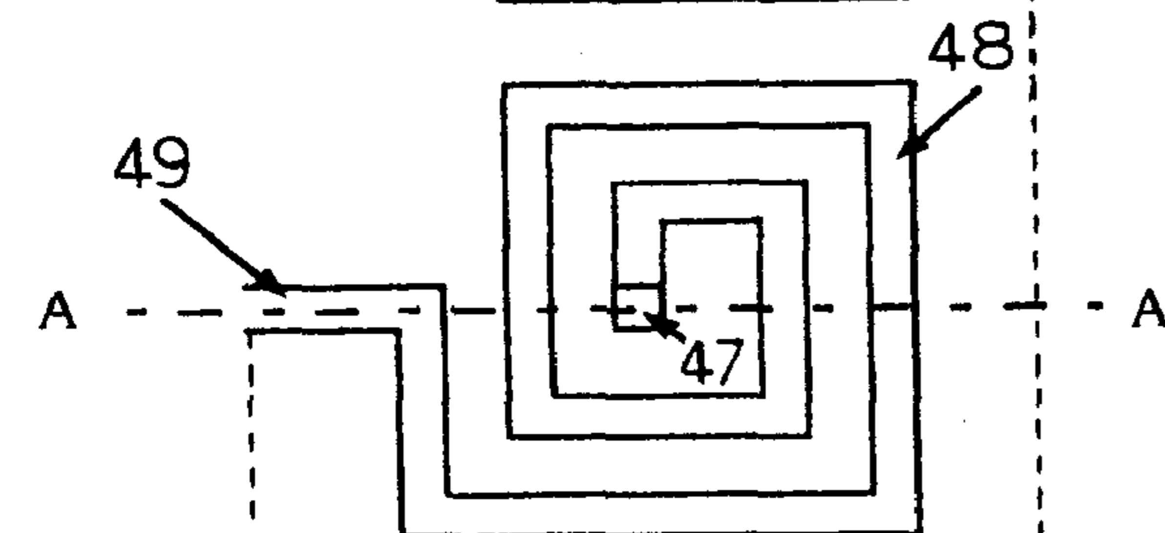
Fig. 4 (d) Top view of the fourth layer
