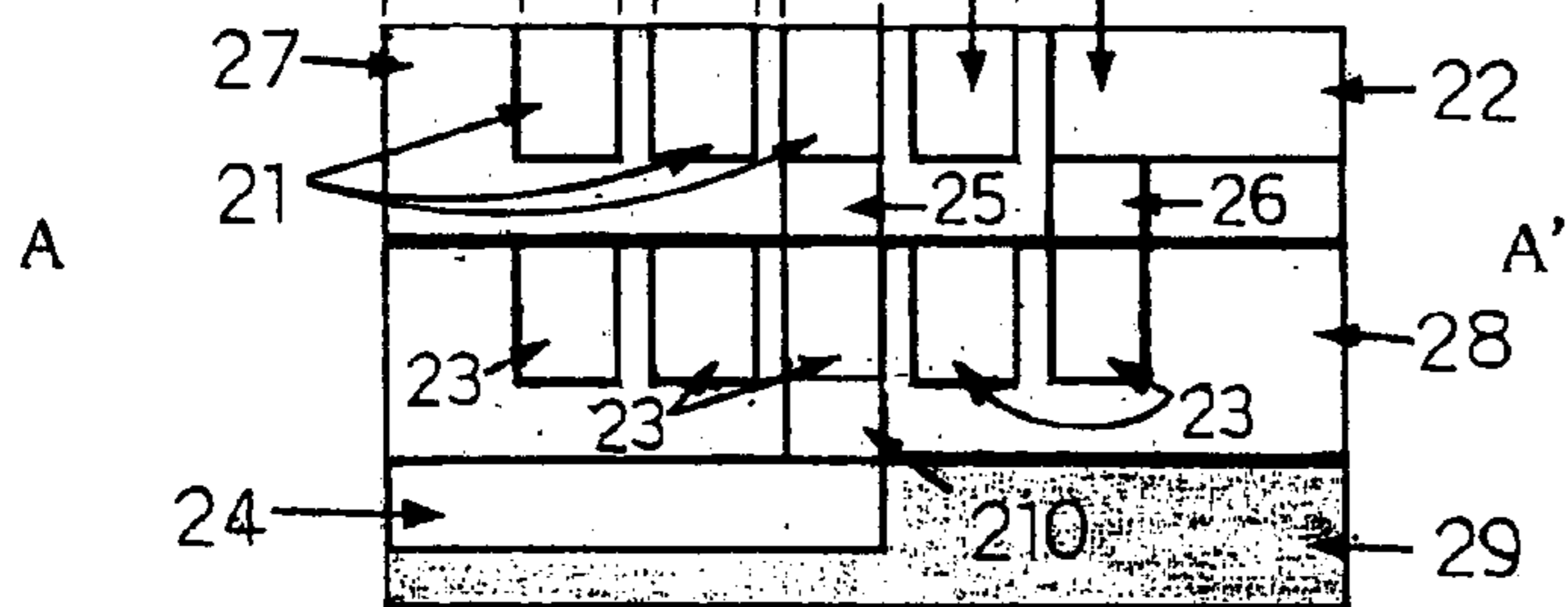
Fig. 2 (d) A-A' cross section
