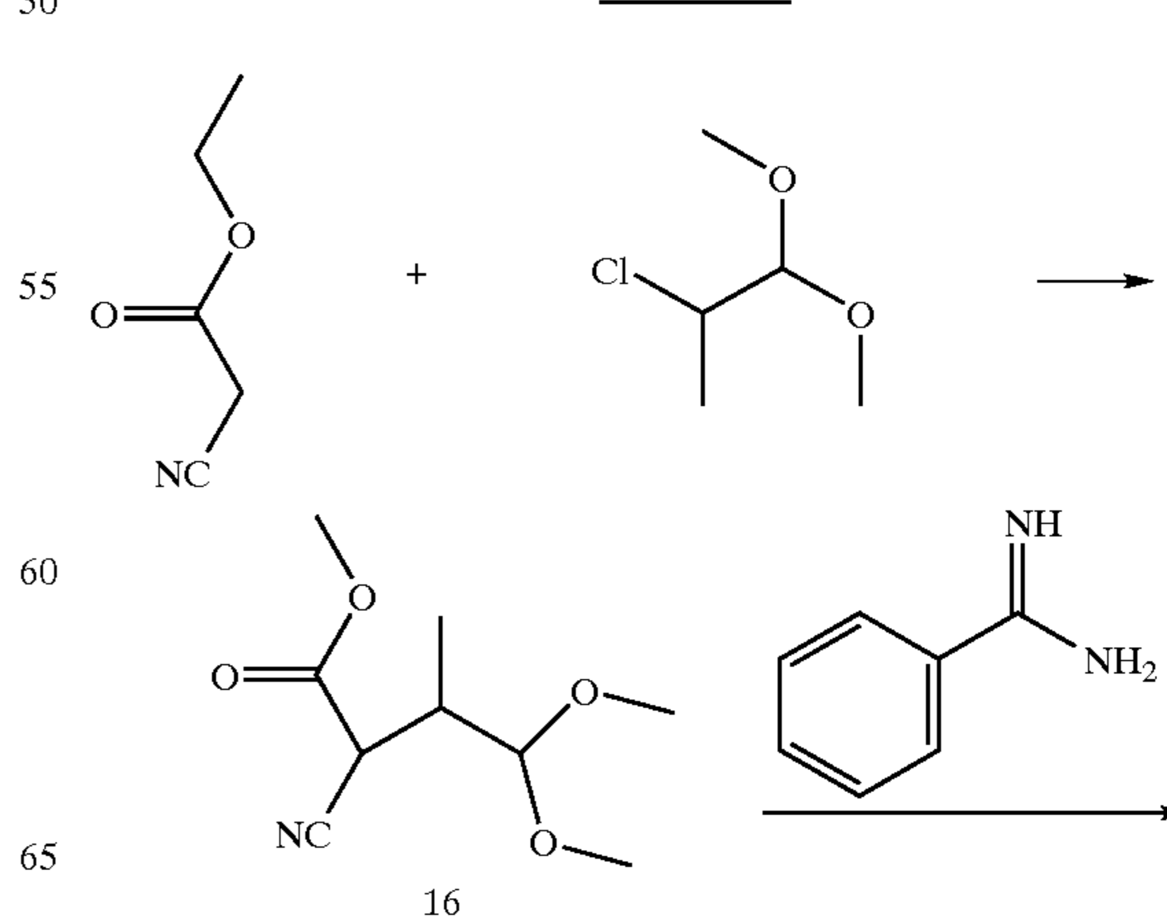
Scheme VI
