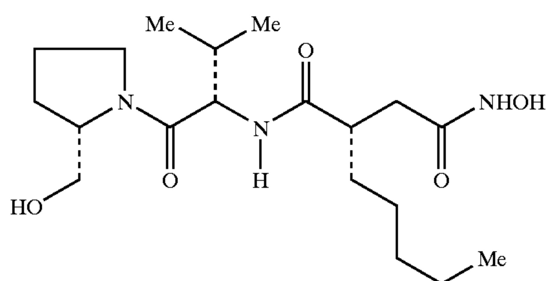
Epiactinonin
