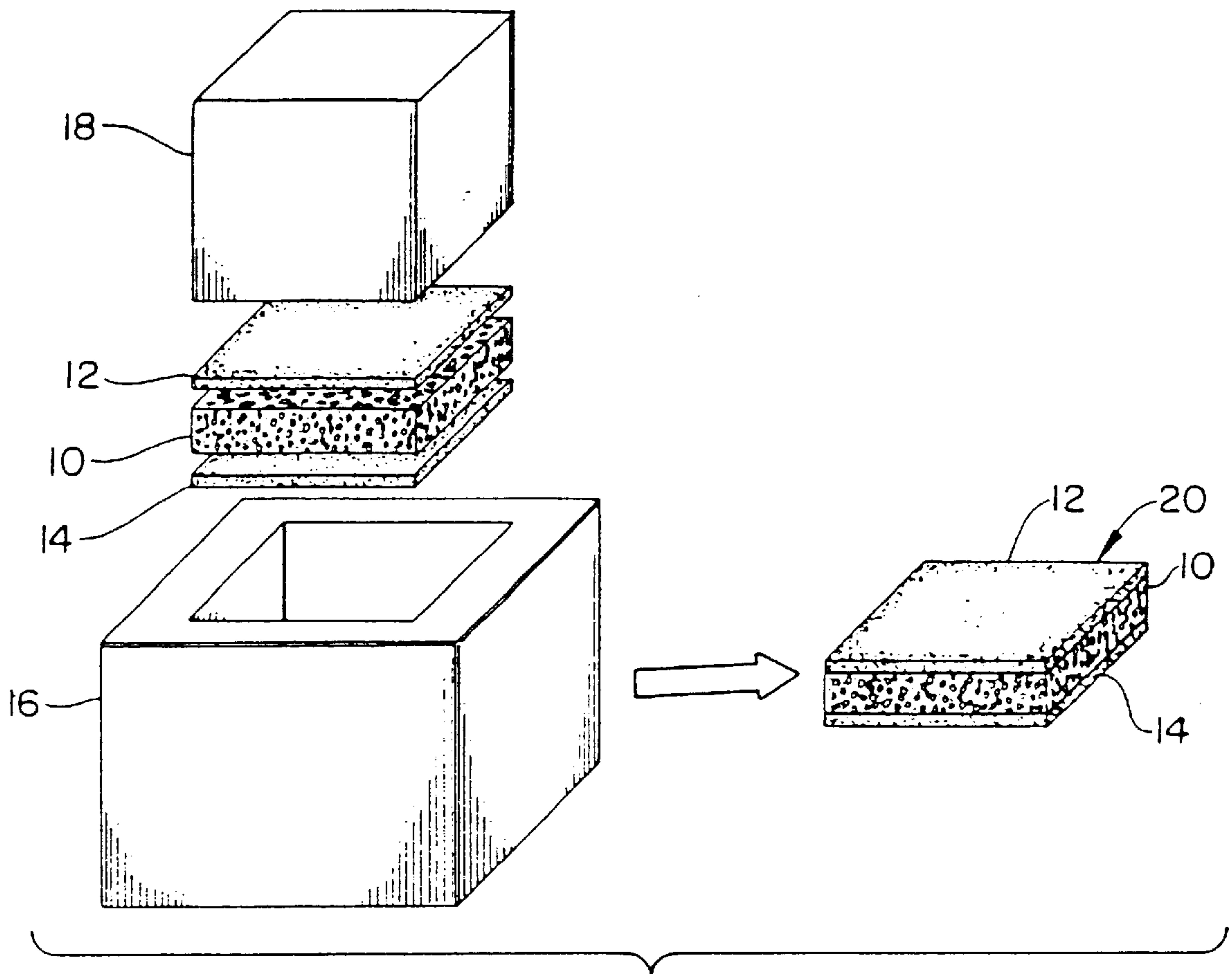
FIG. 13A
