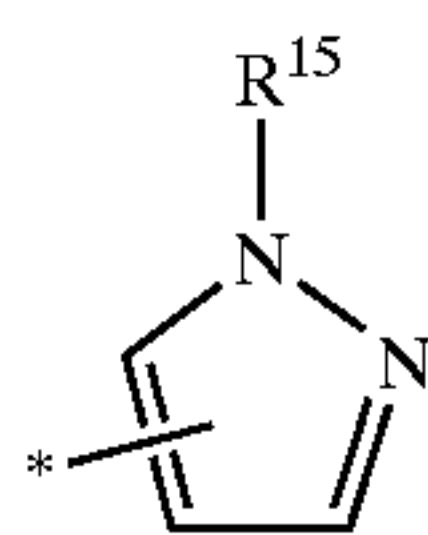
pyrazolyl
