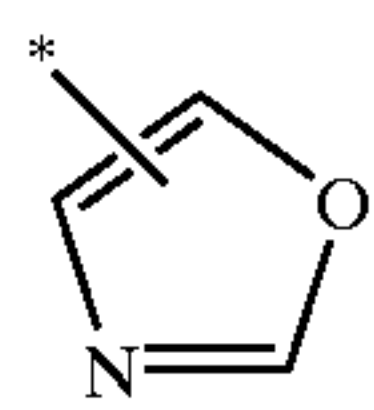
oxazolyl
