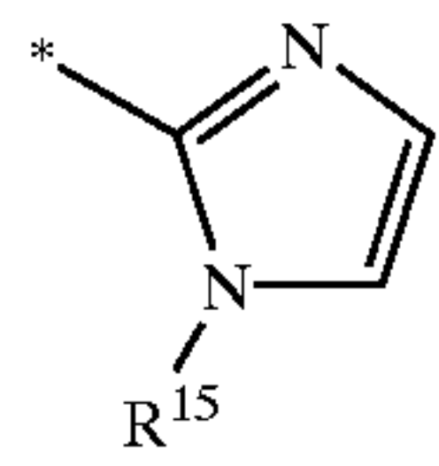
imidazol-2-yl
