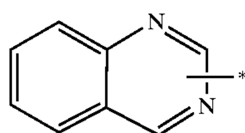
quinazoliny
