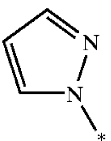
pyrazol-1-yl
