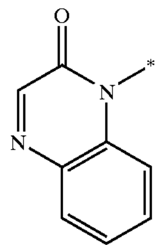
1H-quinoxalin-2-on-1-yl
