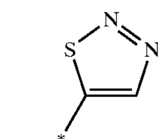
1,2,3-thiadiazol-5-yl
