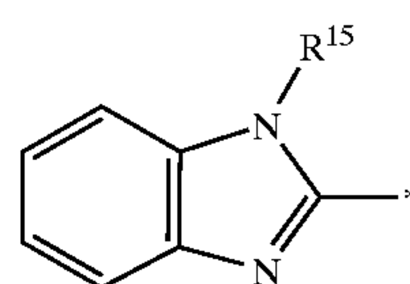
benzimidazolyl
