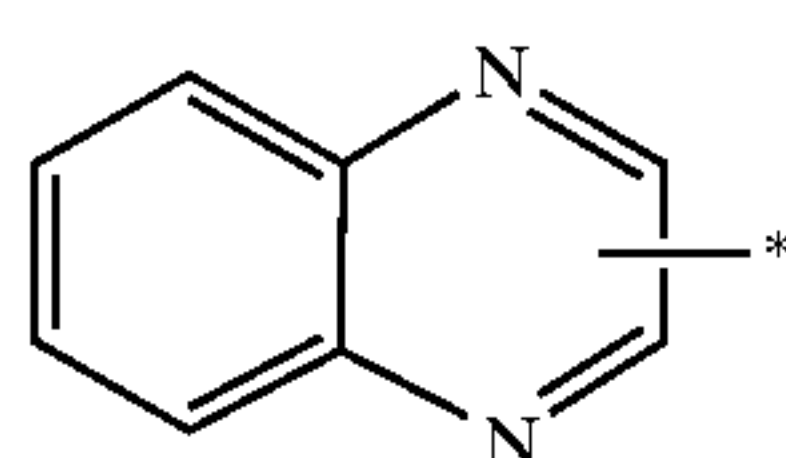
quinoxaliny
