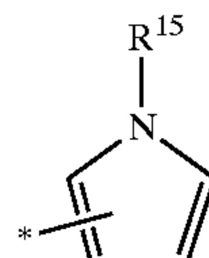
pyrrolyl
