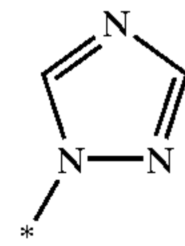
1H-1,2,4-triazol-1-yl
