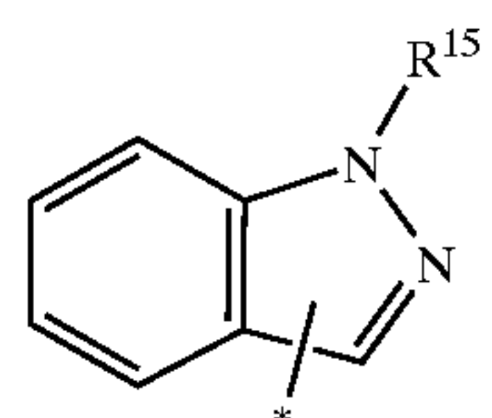
1H-indazolyl
