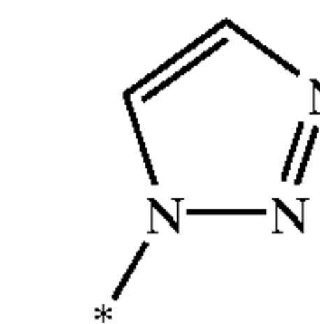
1H-1,2,3-triazol-1-yl
