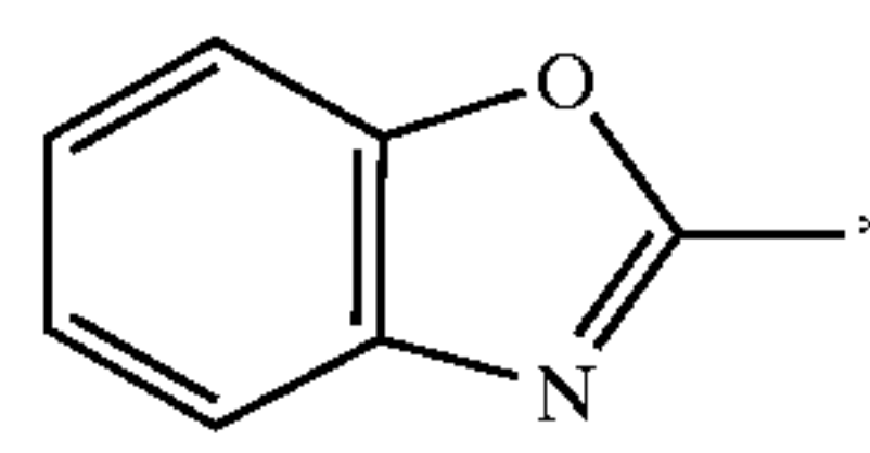
benzoxazolyl
