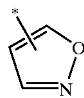
isoxazolyl
