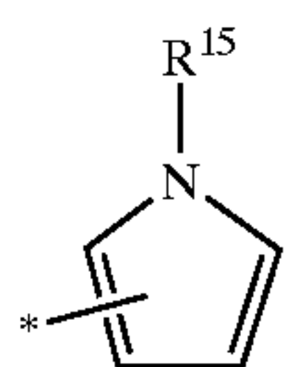
pyrrolyl
