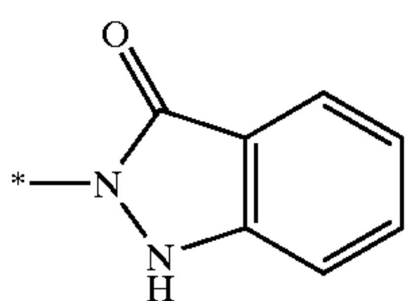
1H-indazol-3-on-2-yl
