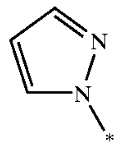
pyrazol-1-yl
