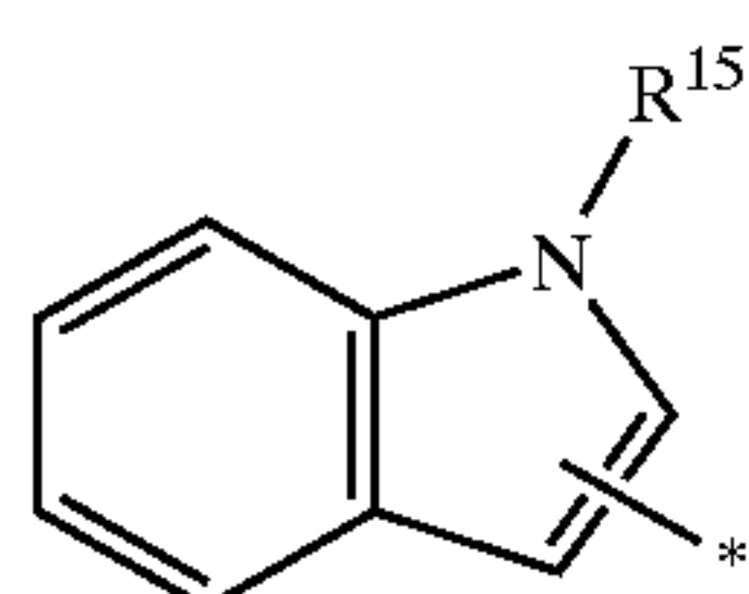
indolyl
