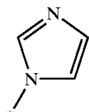
imidazol-1-yl
