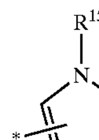
pyrazolyl
