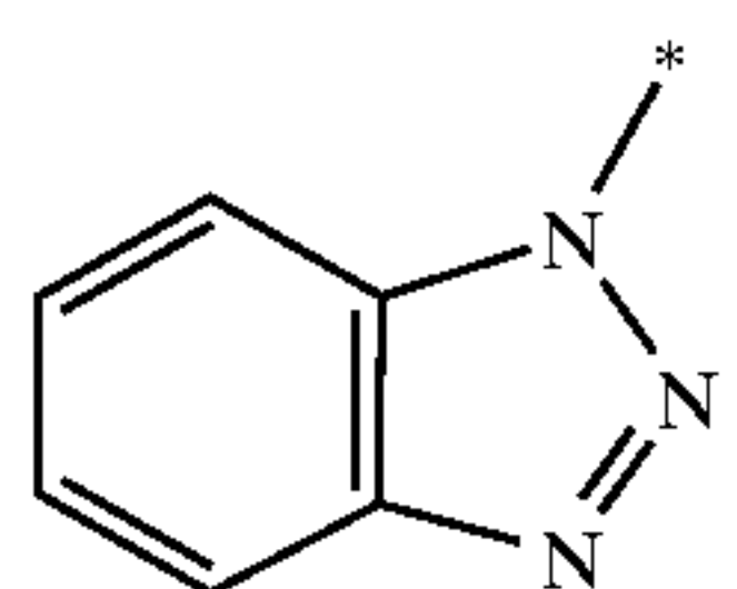
benzotriazolyl
