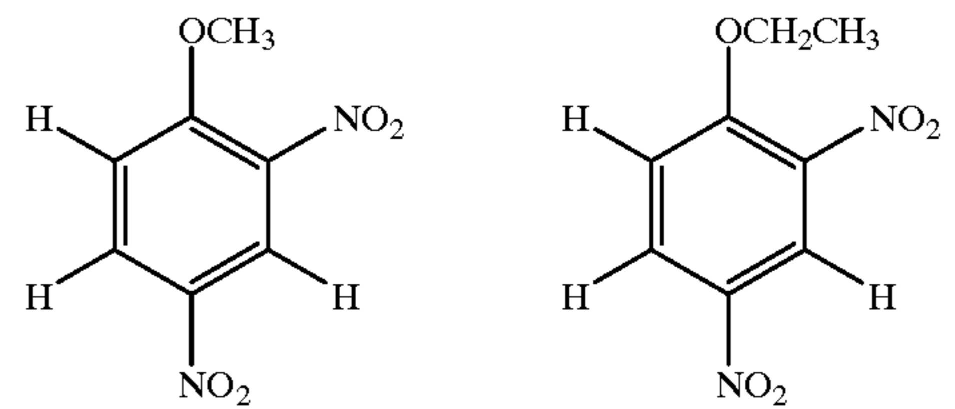
2,4-dinitroanisole (DNAN)
