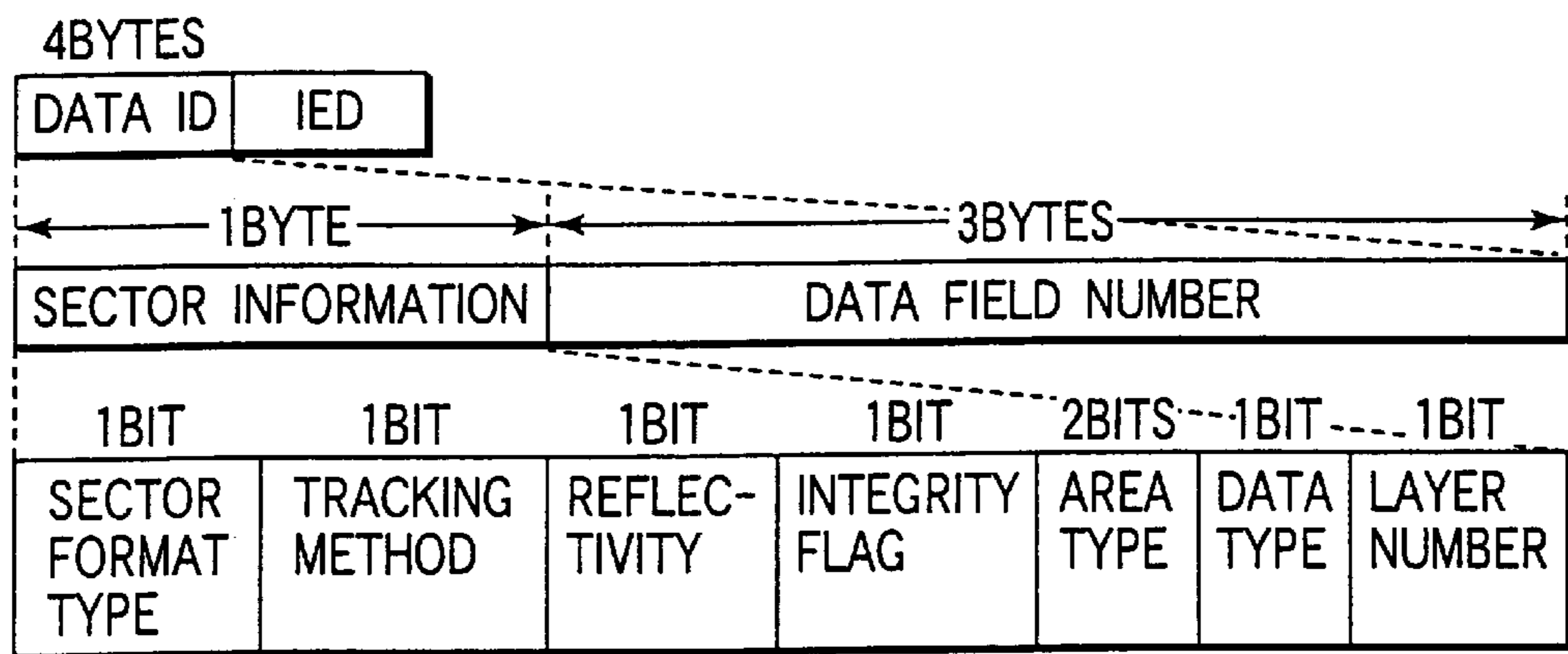
FIG. 5A
