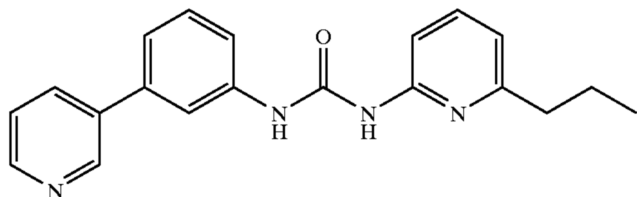
N-[3-(3-Pyridinyl)phenyl]-N'-2-(6-propylpyridinyl)urea
