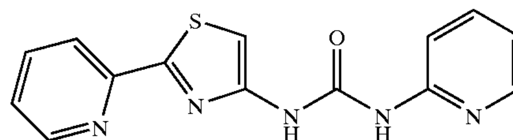
N-[2-(2-Pyridinyl)-4-thiazolyl]-N'-2-pyridinylurea
