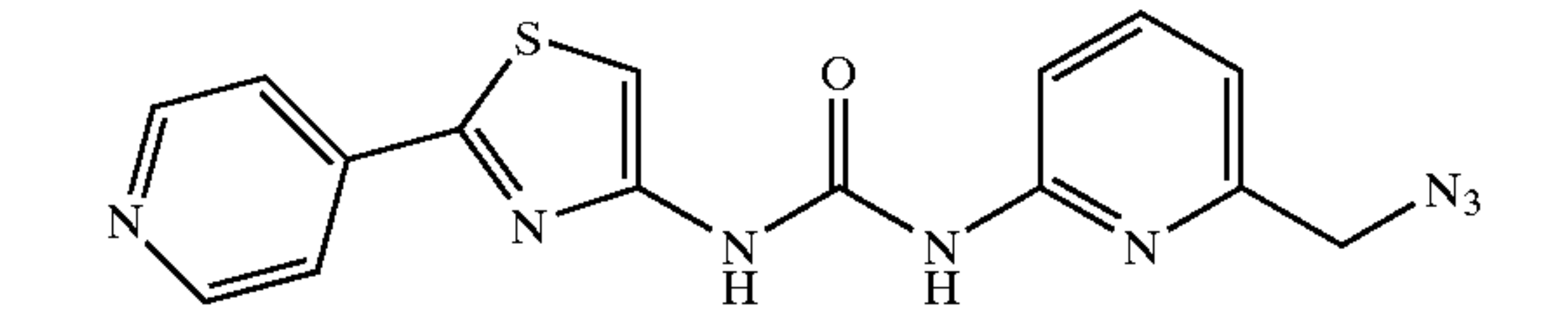
N-(6-azidomethyl-2-pyridyl)-N'-[2-(4-pyridinyl)-4-thiazolyl]urea
