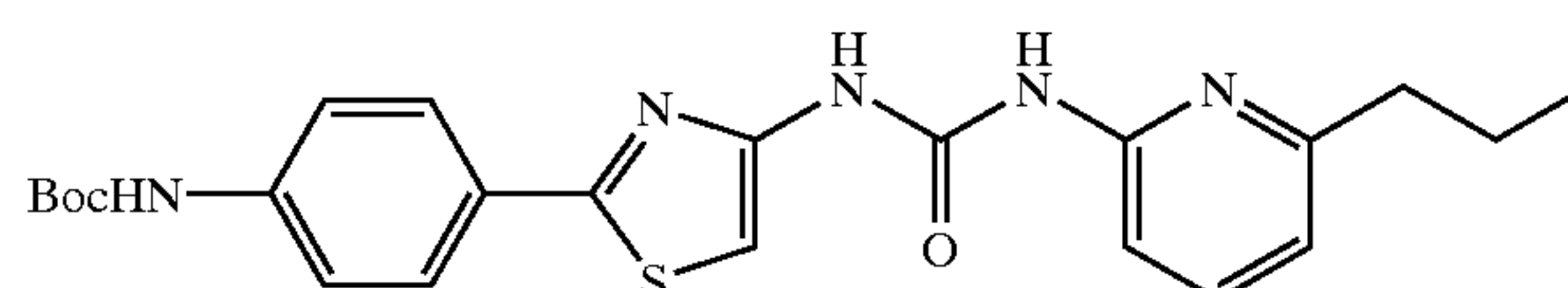
Tert-Butyl (4-{4-[3-(6-propylpyridin-2-yl)ureido]-thiazol-2-yl}phenyl)carbamate
