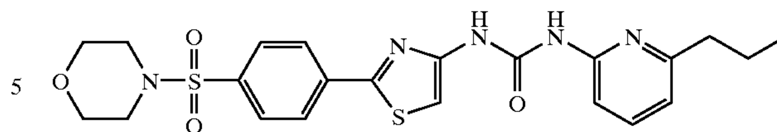
1-{2-[4-(4-Morpholinylsulfonyl)phenyl]thiazol-4-yl}-3-(6-propylpyridin-2-yl)urea
