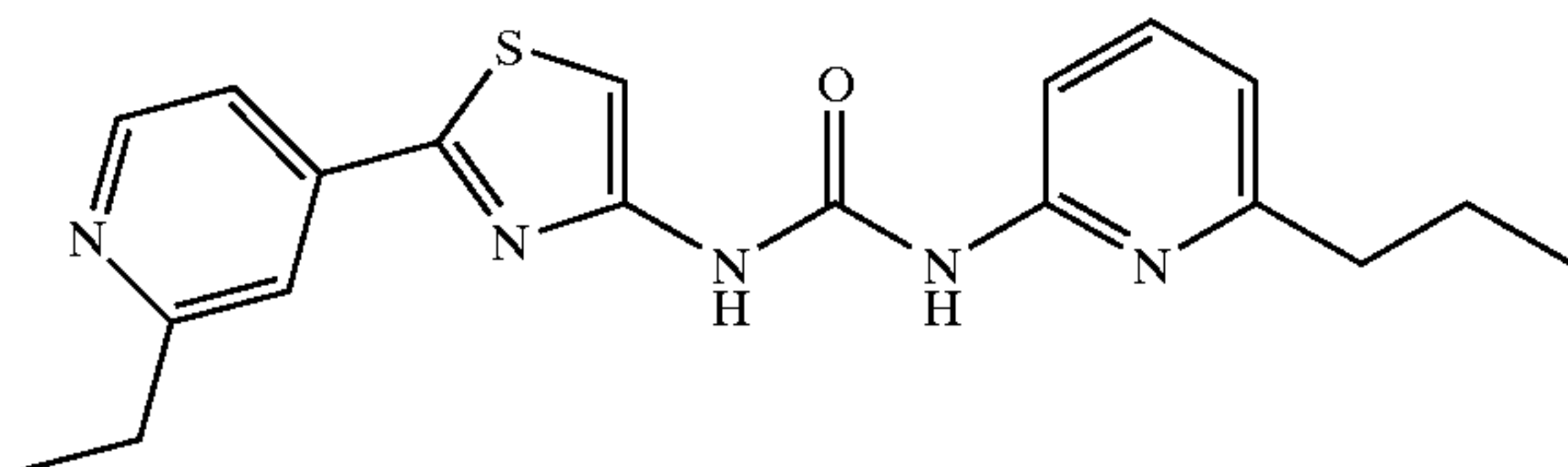
N-[2-(2-Ethyl-4-pyridinyl)-4-thiazolyl]-N'-2-(6-propylpyridinyl)urea
