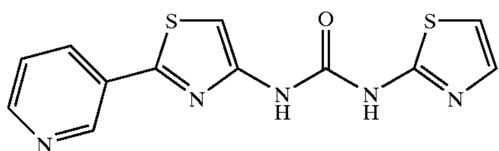
N-[2-(3-Pyridinyl)-4-thiazolyl]-N'-2-thiazolylurea
