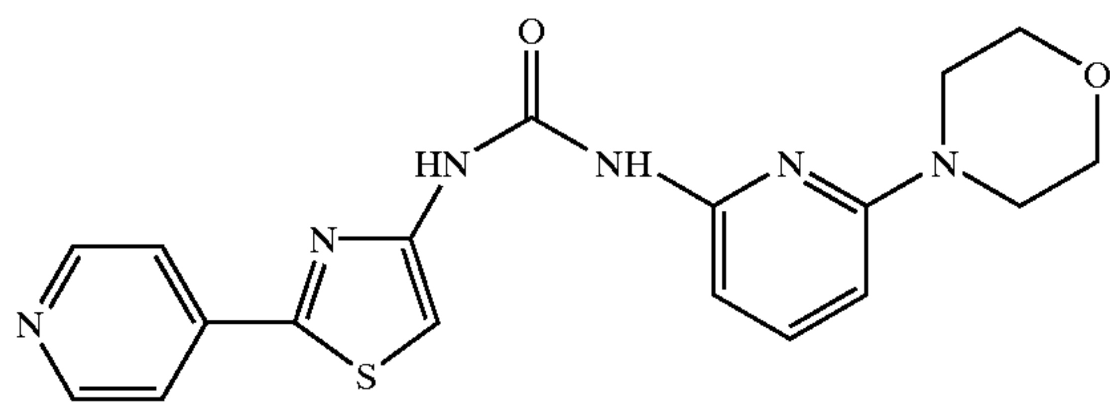
N-[2-(4-Pyridinyl)-4-thiazolyl]-N'-2-[6-(4-morpholinyl)pyridinyl]urea
