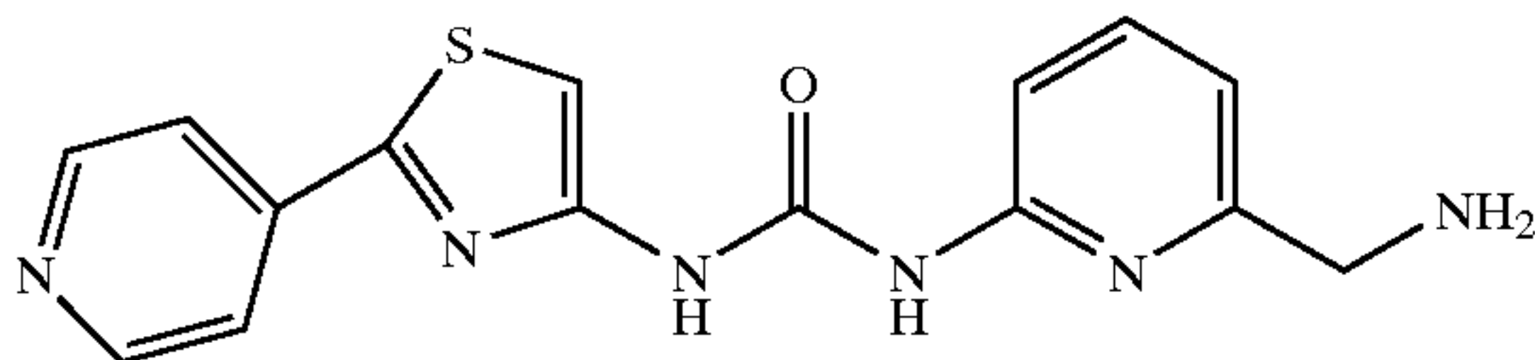
N-(6-Aminomethyl-2-pyridyl)-N'-[2-(4-pyridinyl)-4-thiazolyl]urea
