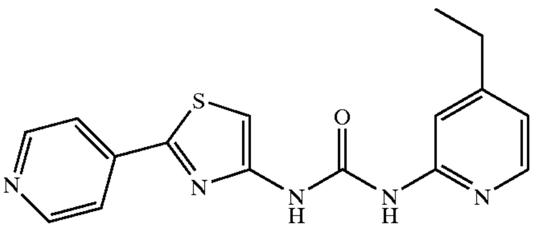
N-[2-(4-Pyridinyl)-4-thiazolyl]-N'-2-(4-ethylpyridinyl)urea
