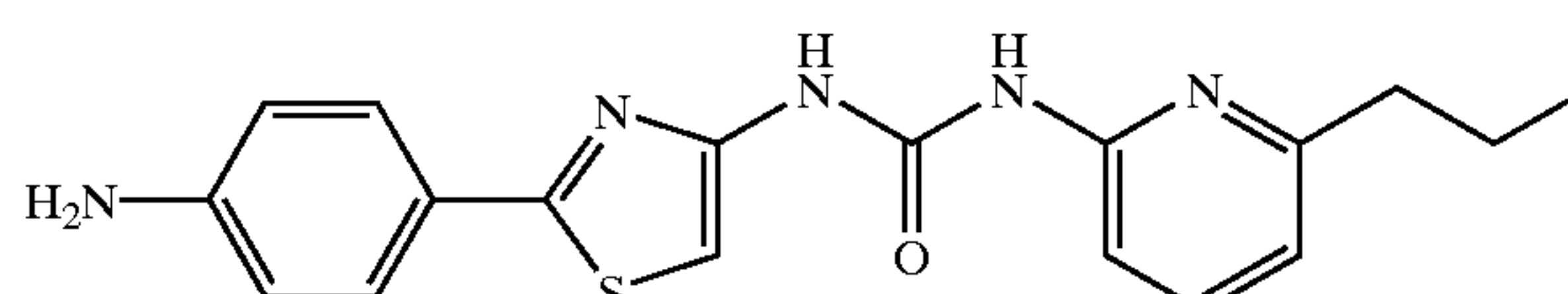
1-[2-(4-Aminophenyl)thiazol-4-yl]-3-(6-propylpyridin-2-yl)urea
