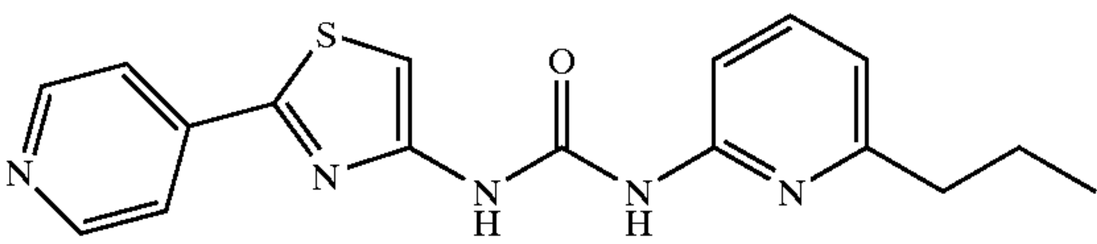
N-[2-(4-Pyridinyl)-4-thiazolyl]-N'-2-(6-propylpyridinyl)urea
