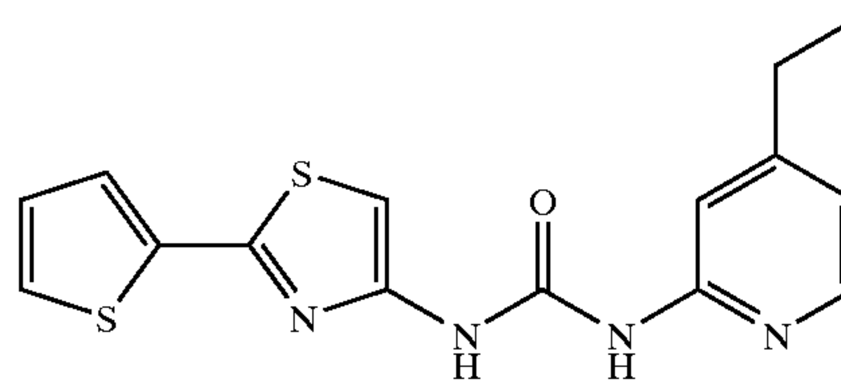
N-[2-(2-Thienyl)-4-thiazolyl]-N'-2-(4-ethylpyridinyl)urea
