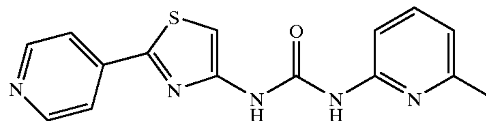
N-[2-(4-Pyridinyl)-4-thiazolyl]-N'-2-(6-methylpyridinyl)urea
