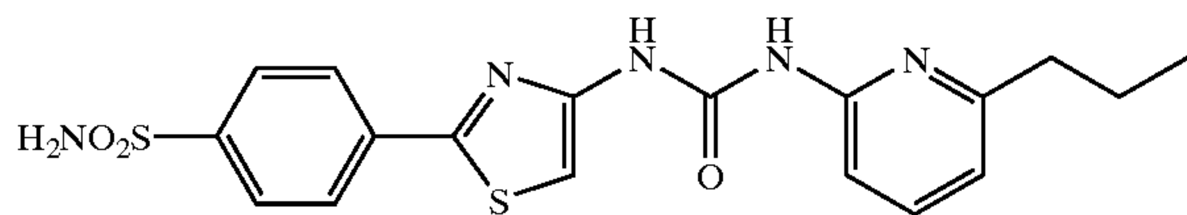
4-{4-[3-(6-Propyl-pyridin-2-yl)-ureido]-thiazol-2-yl}-benzenesulfonamide
