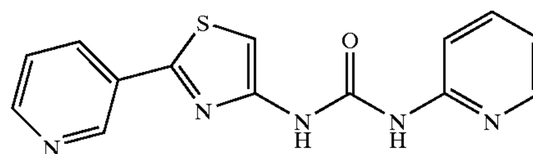
N-[2-(3-Pyridinyl)-4-thiazolyl]-N'-2-pyridinylurea
