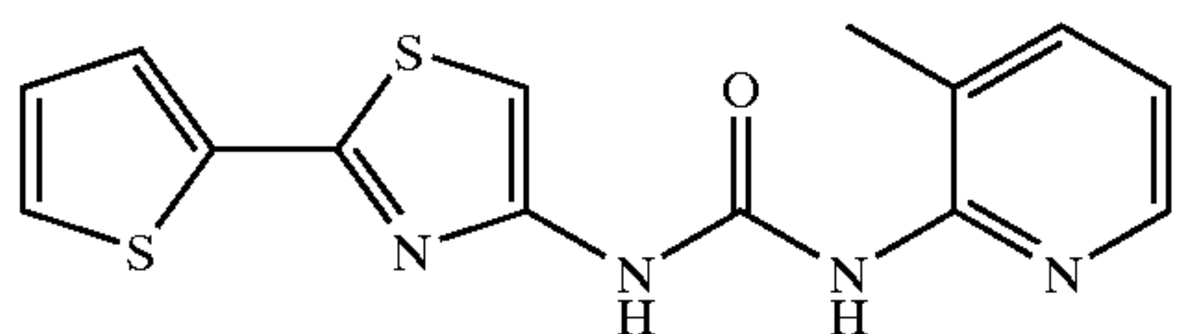
N-[2-(2-Thienyl)-4-thiazolyl]-N'-2-(3-methylpyridinyl)urea
