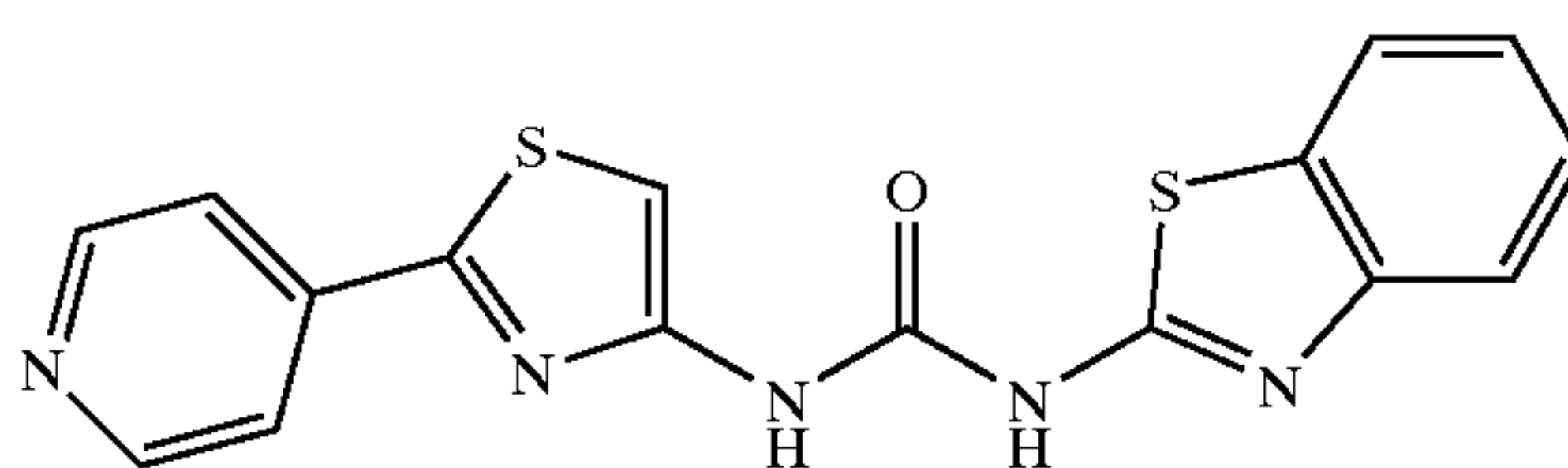
N-[2-(4-Pyridinyl)-4-thiazolyl]-N'-2-benzthiazolylurea
