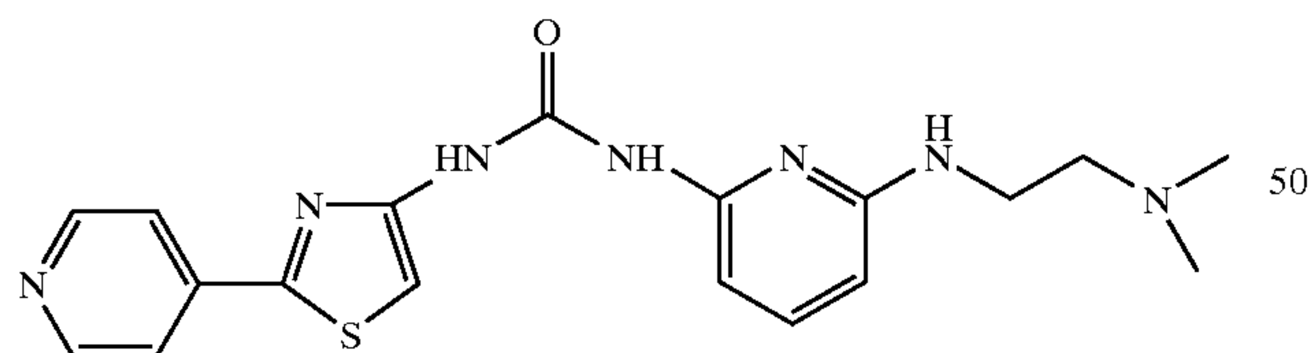
N-[2-(4-Pyridinyl)-4-thiazolyl]-N'-2-[6-(N'',N''-aminoethylamino)pyridinyl]urea
