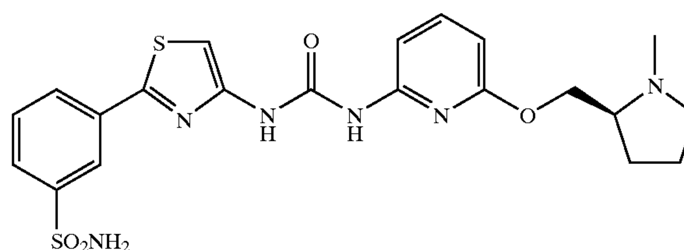
3-(4-{3-[6-(1-Methyl-pyrrolidin-2-ylmethoxy)-pyridin-2-yl]-ureido}-thiazol-2-yl)-benzenesulfonamide
