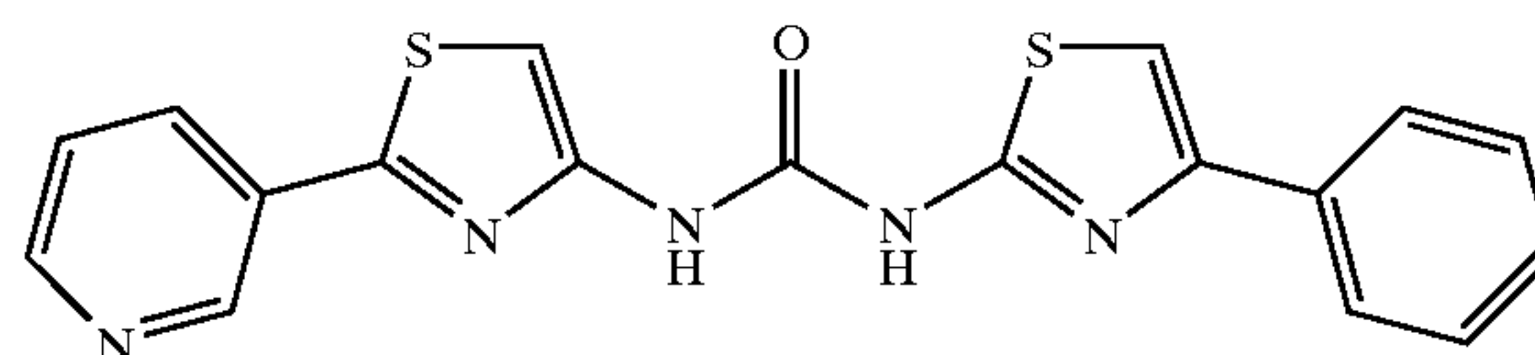
N-[2-(3-Pyridinyl)-4-thiazolyl]-N'-[4-phenyl-2-thiazolyl]urea
