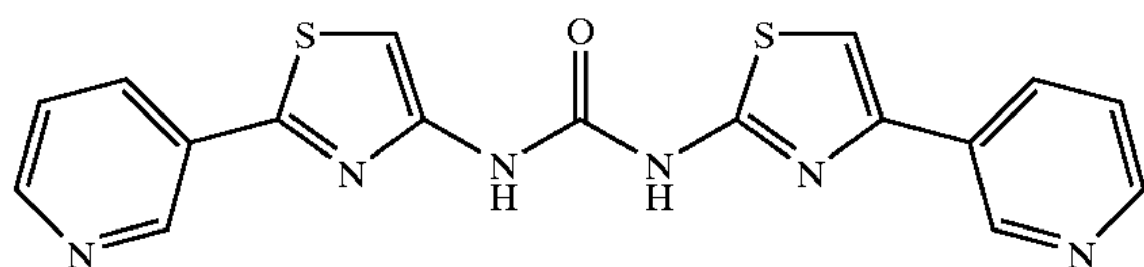
N-[2-(3-Pyridinyl)-4-thiazolyl]-N'-[4-(3-pyridinyl)-2-thiazolyl] urea
