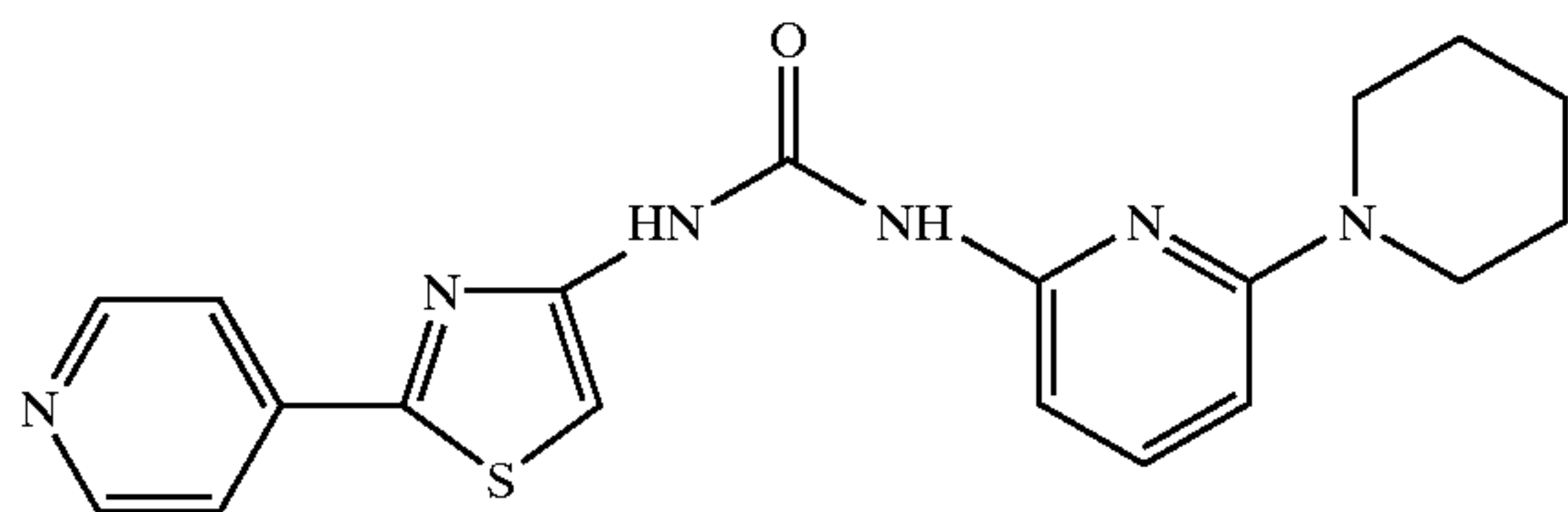
N-[2-(4-Pyridinyl)-4-thiazolyl]-N'-2-[6-(1-piperidinyl)pyridinyl]urea
