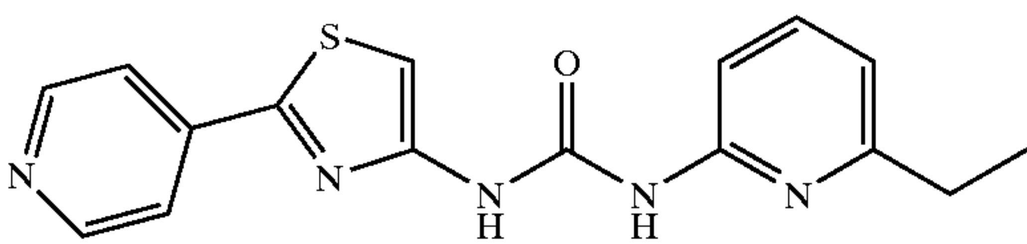
N-[2-(4-Pyridinyl)-4-thiazolyl]-N'-2-(6-ethylpyridinyl)urea
