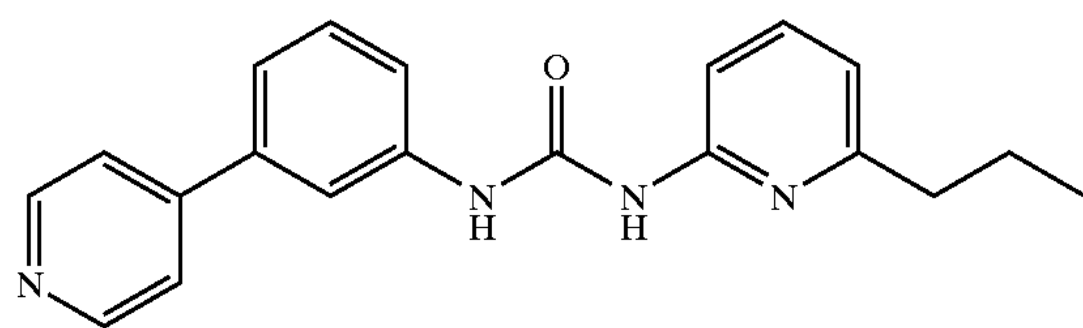
N-[3-(4-Pyridinyl)phenyl]-N'-2-(6-propylpyridinyl)urea
