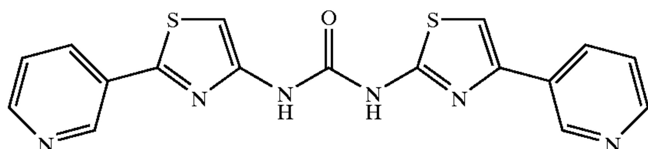
N-[2-(3-Pyridinyl)-4-thiazolyl]-N'-[4-(3-pyridinyl)-2-thiazolyl] urea
