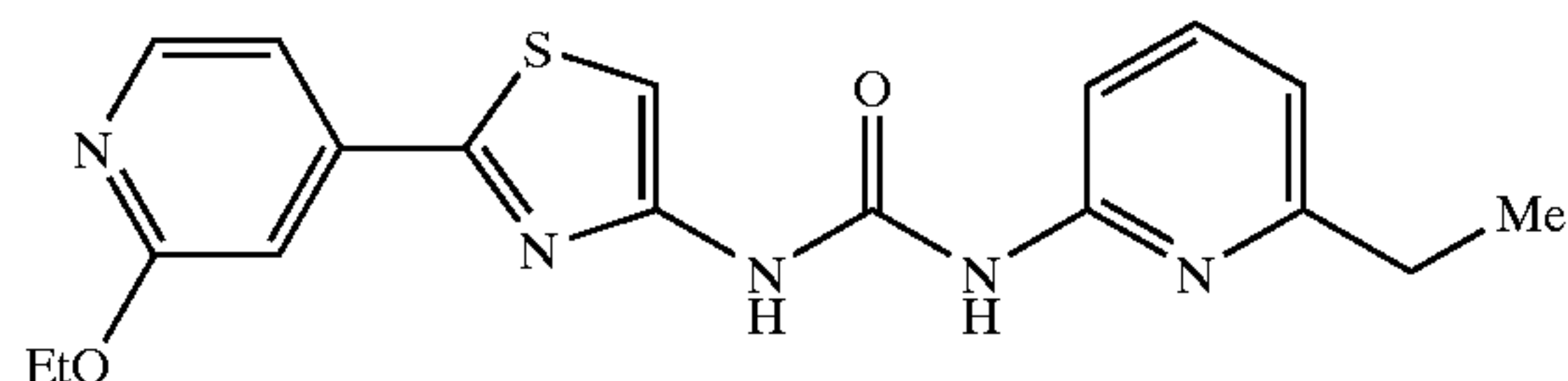
1-[2-(2-Ethoxypyridin-4-yl)thiazol-4-yl]-3-(6-ethylpyridin-2-yl)urea
