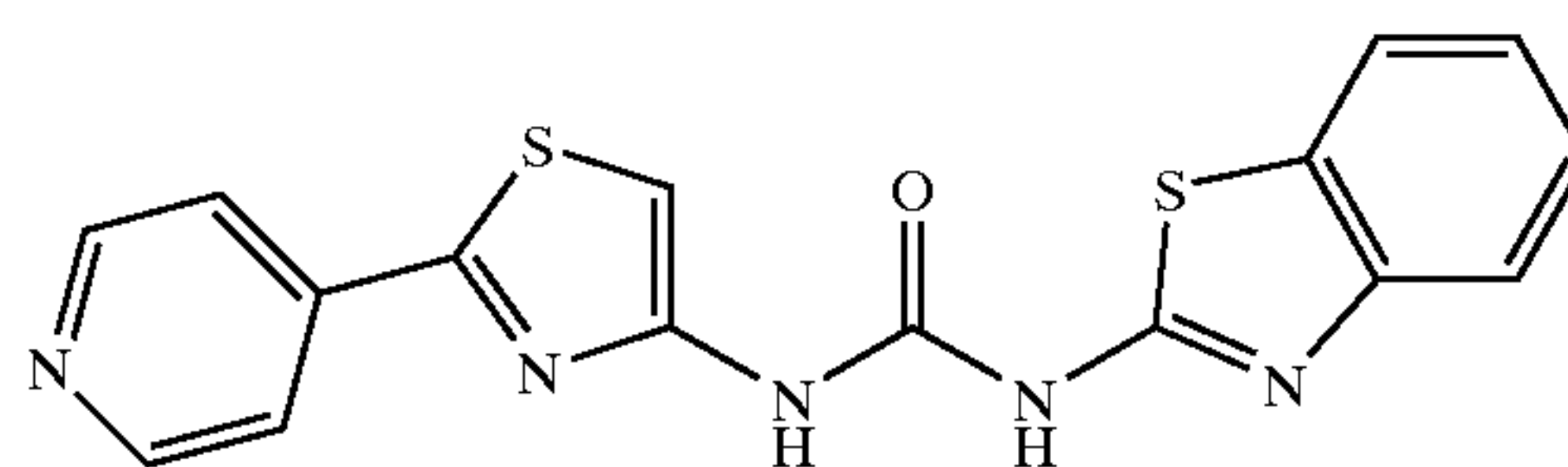
N-[2-(4-Pyridinyl)-4-thiazolyl]-N'-2-benzthiazolylurea
