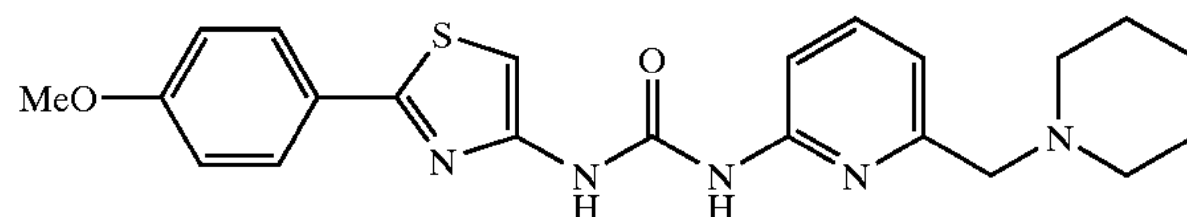
1-[2-(4-Methoxyphenyl)thiazol-4-yl]-3-(6-piperidin-1-ylmethylpyridin-2-yl)urea
