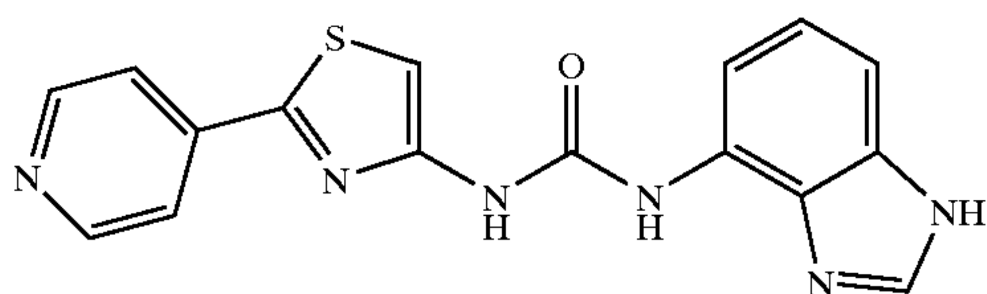
N-[2-(4-Pyridinyl)-4-thiazolyl]-N'-4-benzimidazolylurea
