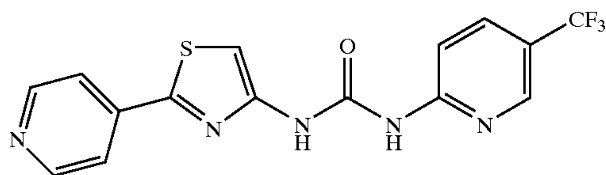
N-[2-(4-Pyridinyl)-4-thiazolyl]-N'-2-(5-trifluoromethylpyridinyl)urea
