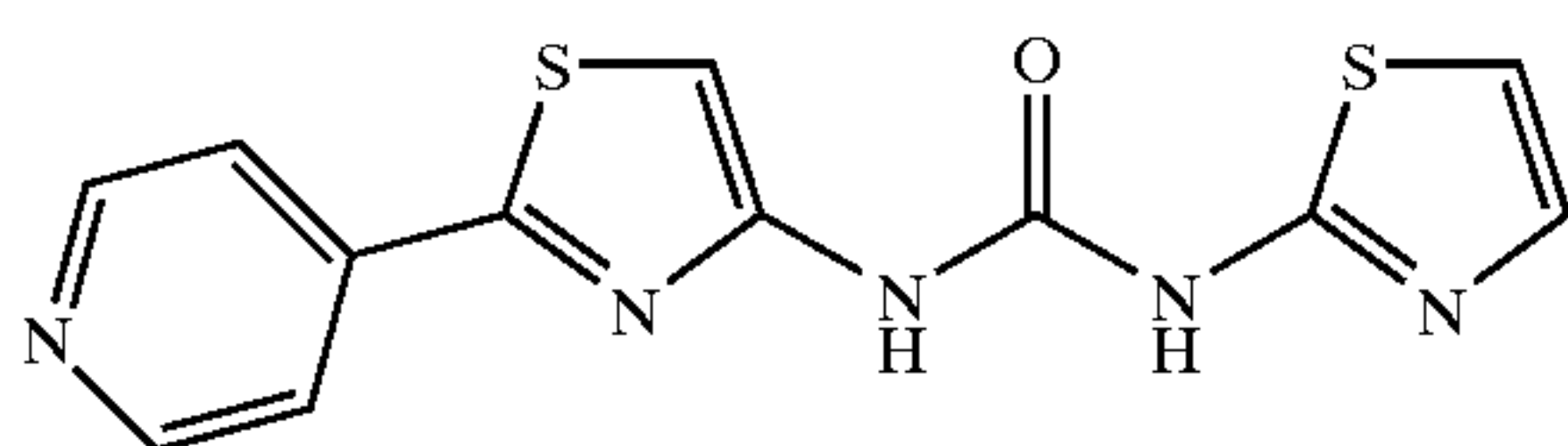
N-[2-(4-Pyridinyl)-4-thiazolyl]-N'-2-thiazolylurea
