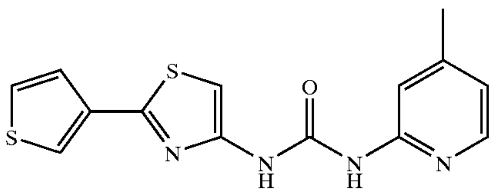
N-[2-(3-Thienyl)-4-thiazolyl]-N'-2-(4-methylpyridinyl)urea
