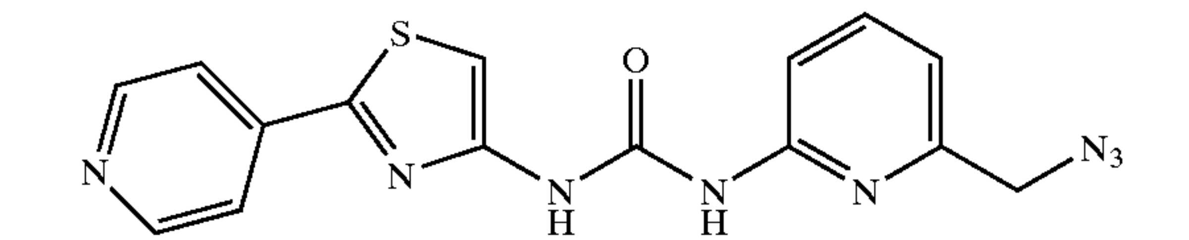
N-(6-azidomethyl-2-pyridyl)-N'-[2-(4-pyridinyl)-4-thiazolyl]urea
