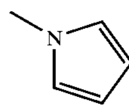
pyrroles
