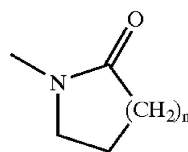
lactam
