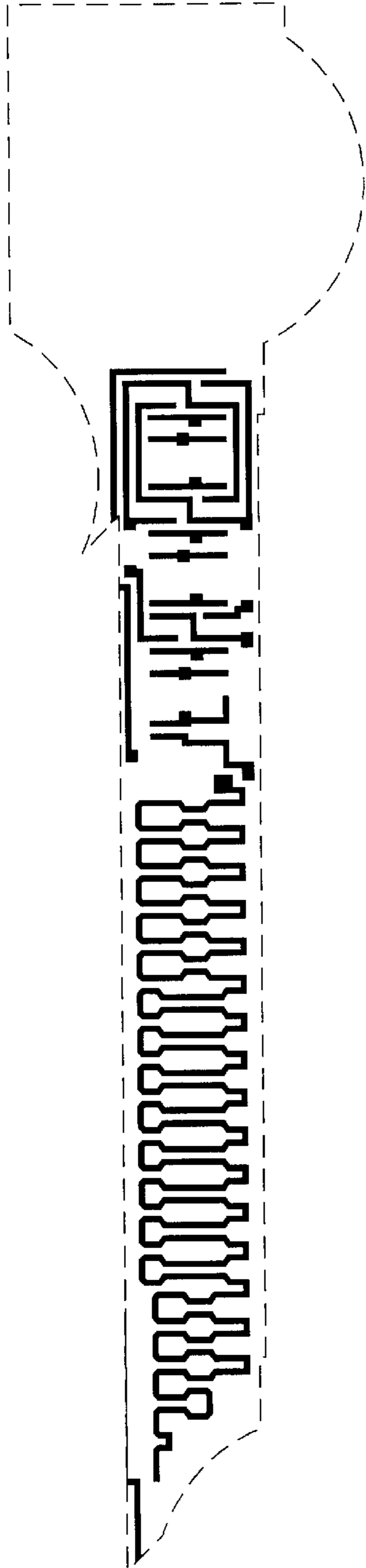
Poly mask
