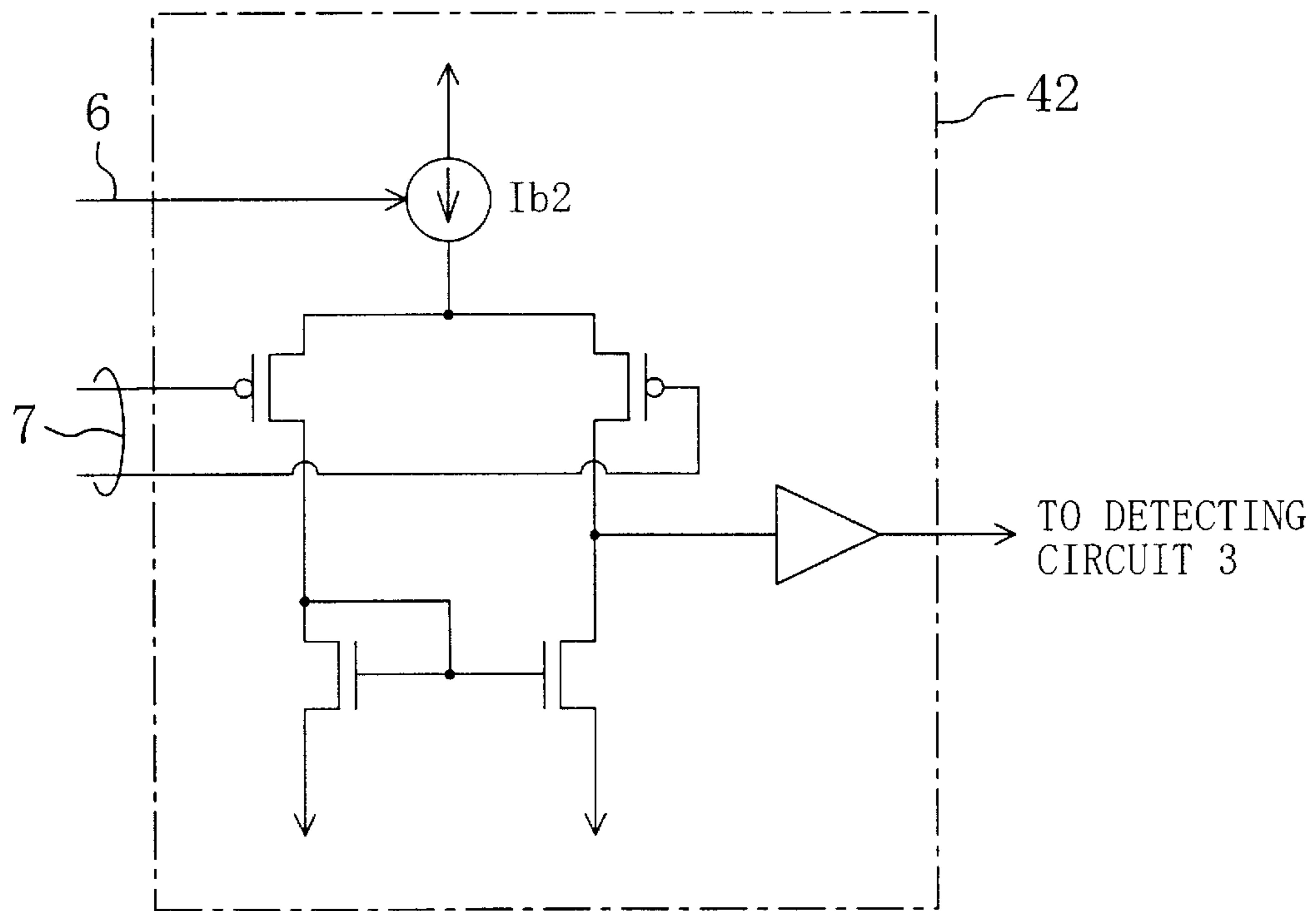
Fig. 2B
