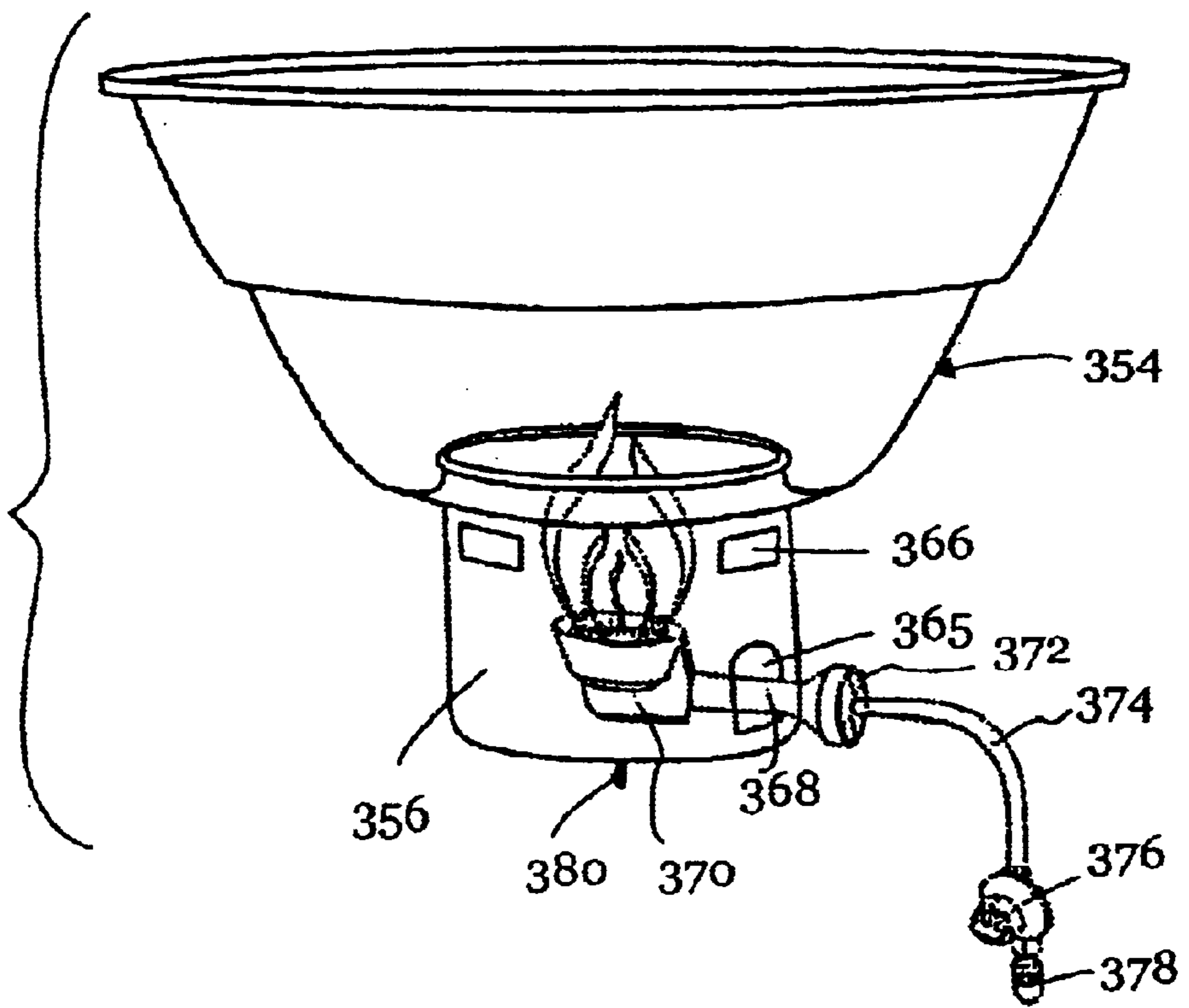
Fig. 15B
