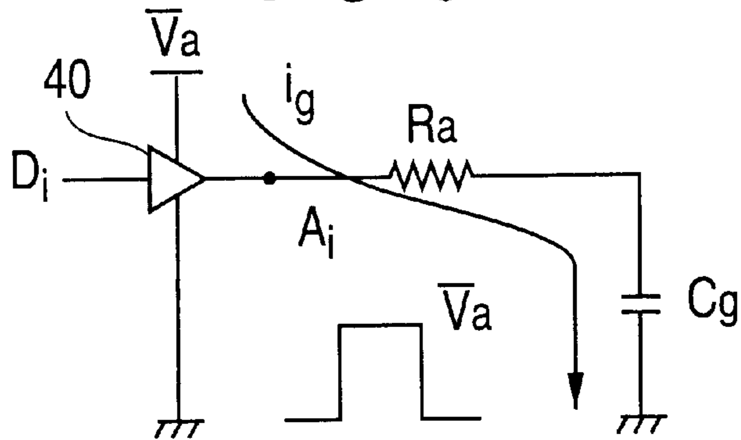
FIG. 9
