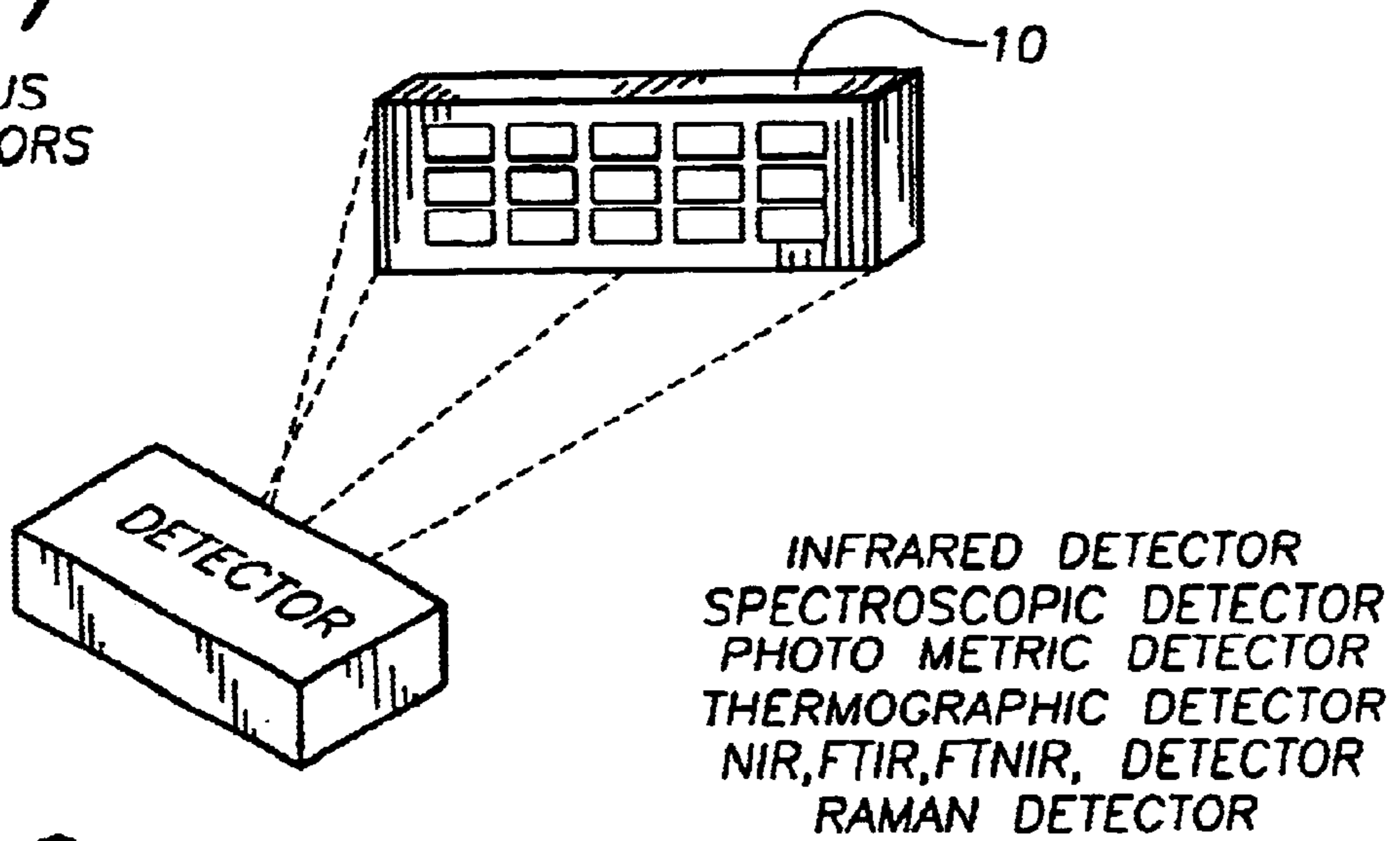
FIG. 8 THERMAL TESTING
