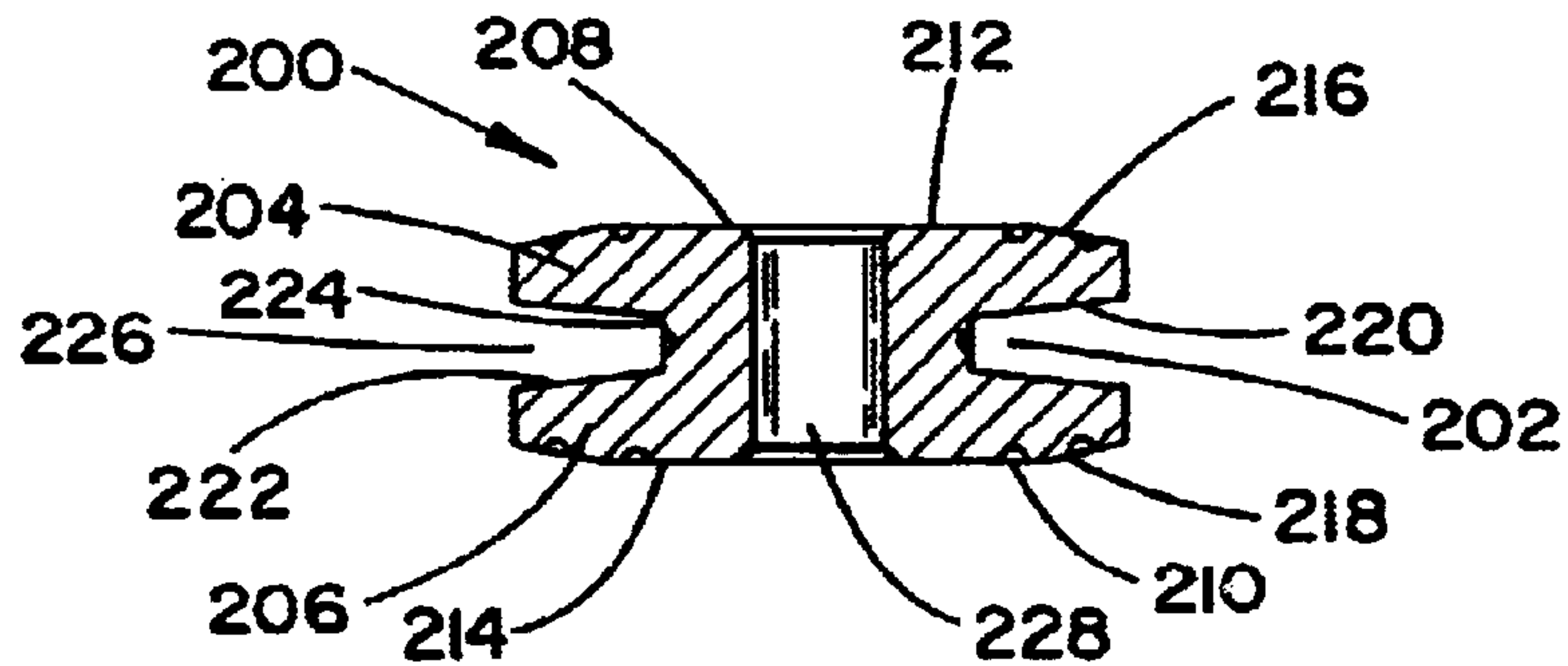
Section A-A
