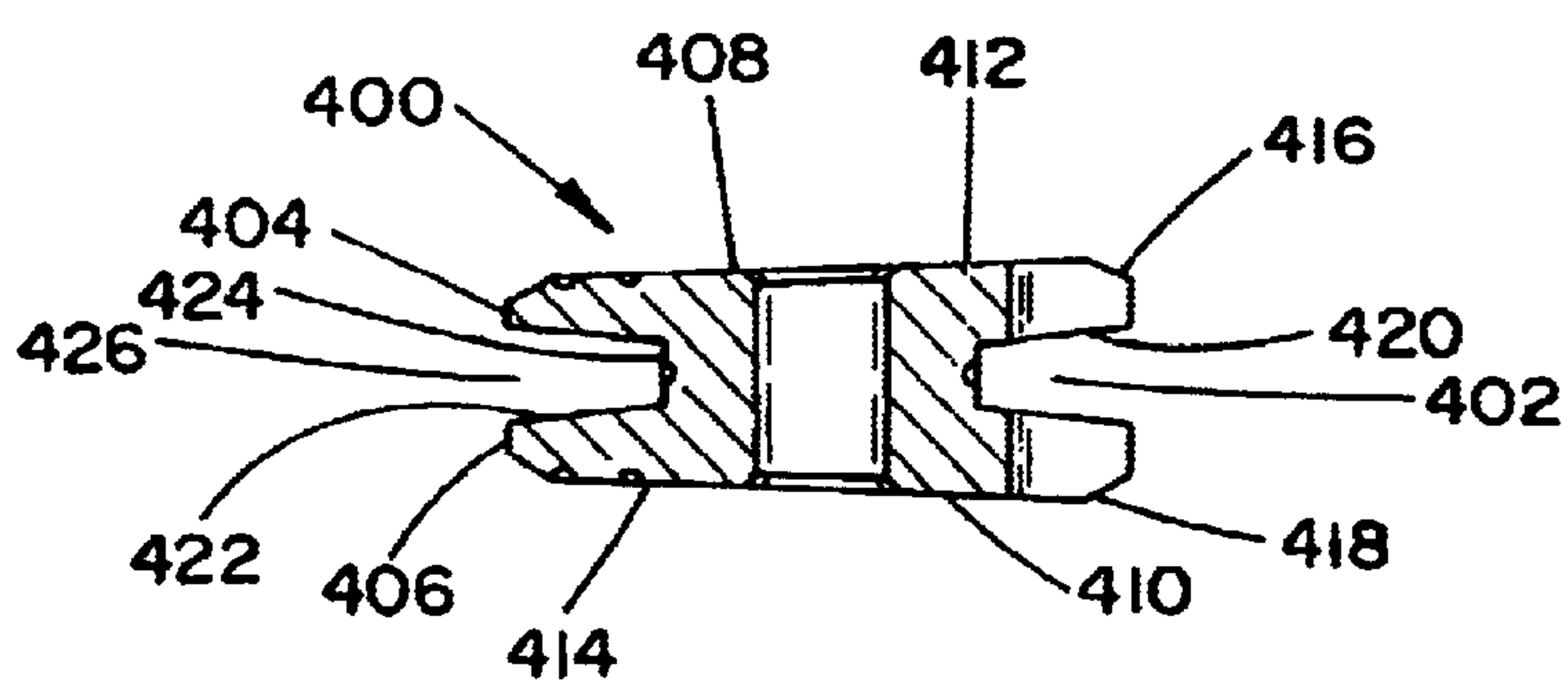
Section A-A
