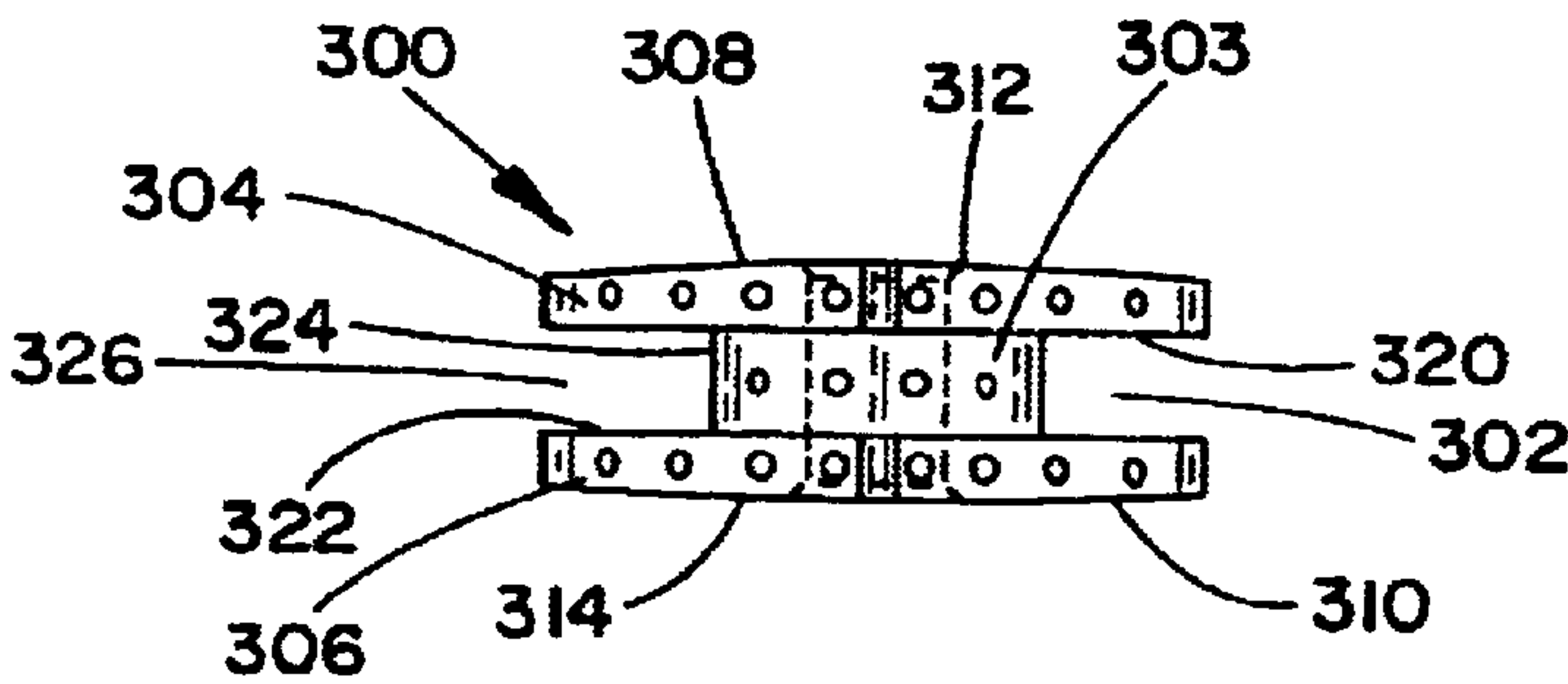
Section B-B FIG. 3b
