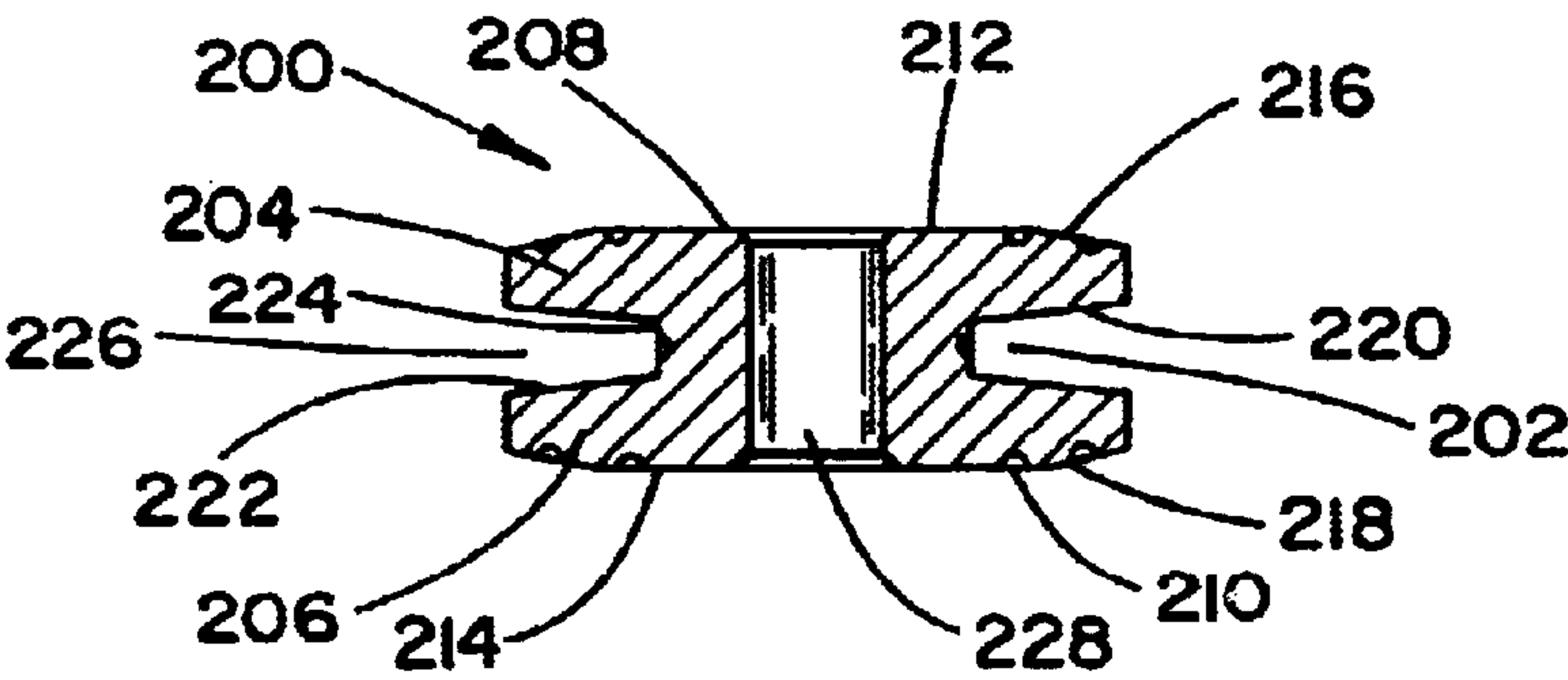
Section A-A FIG. 2c
