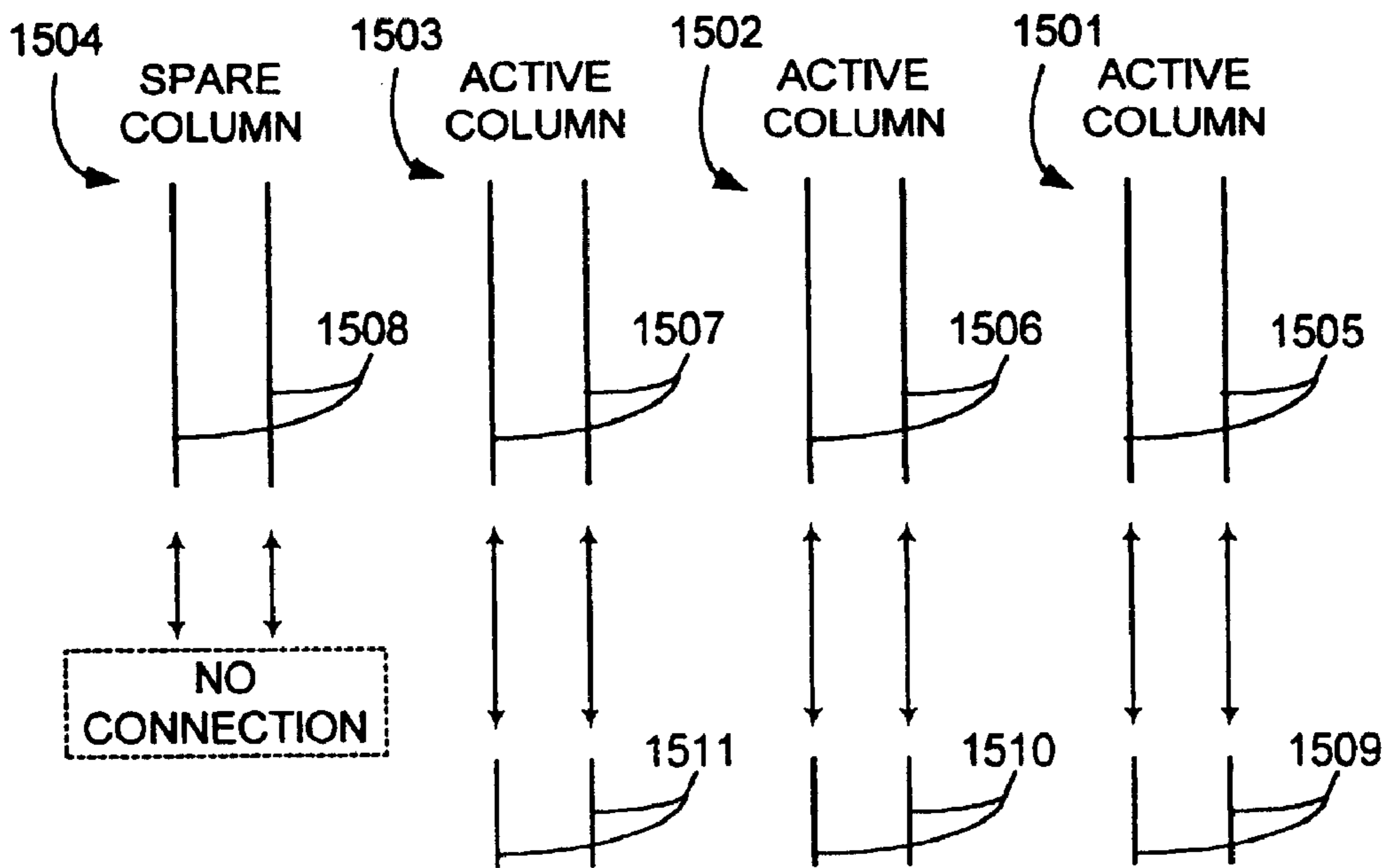
FIG. 15A
