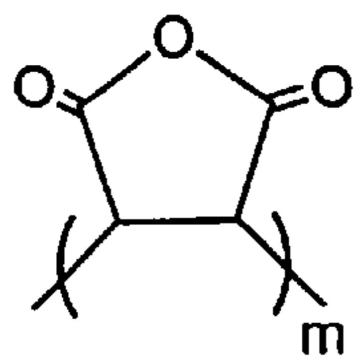
Poly(maleic anhydride)
