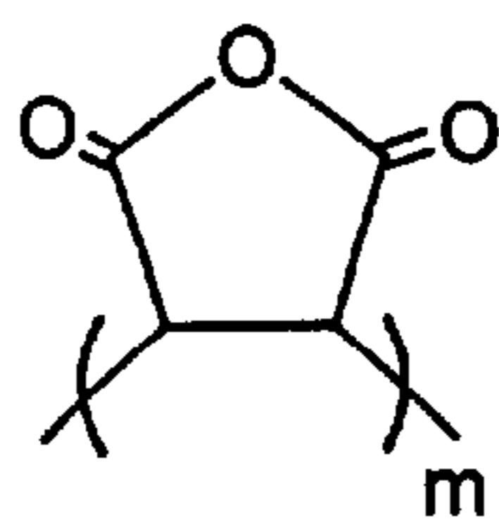
Poly(maleic anhydride)
