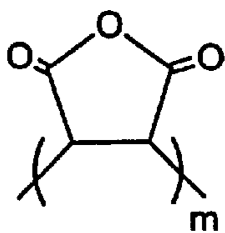
Poly(maleic anhydride)
