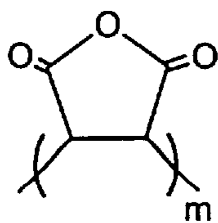
Poly(maleic anhydride)
