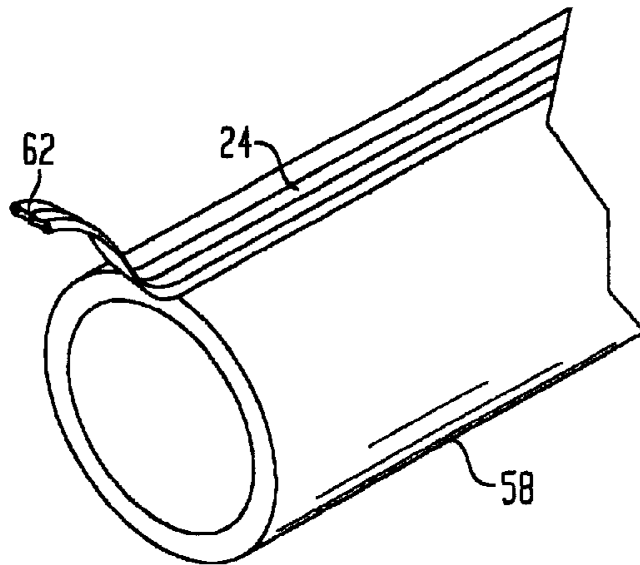
FIG. 3A
