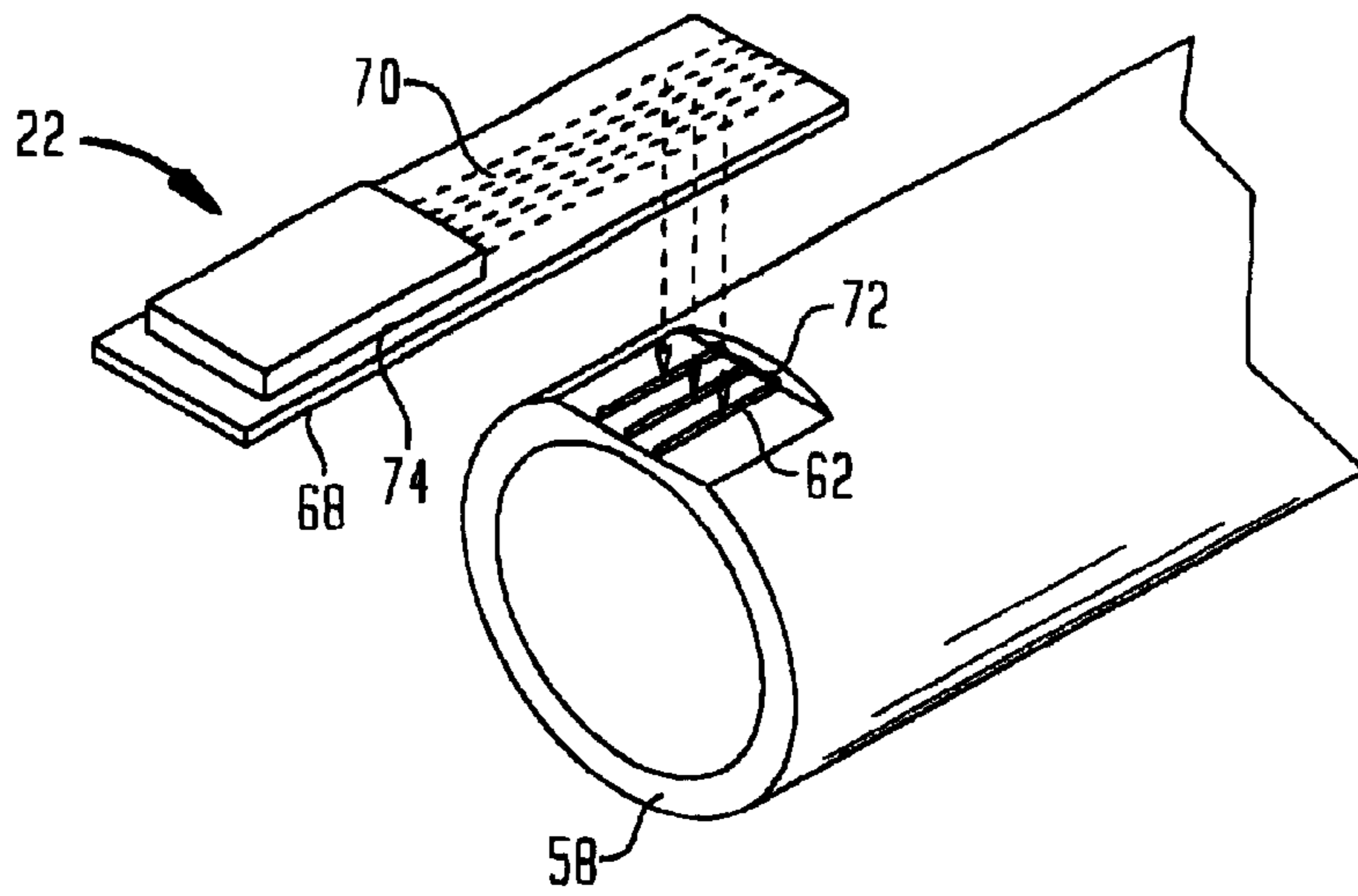
FIG. 5C
