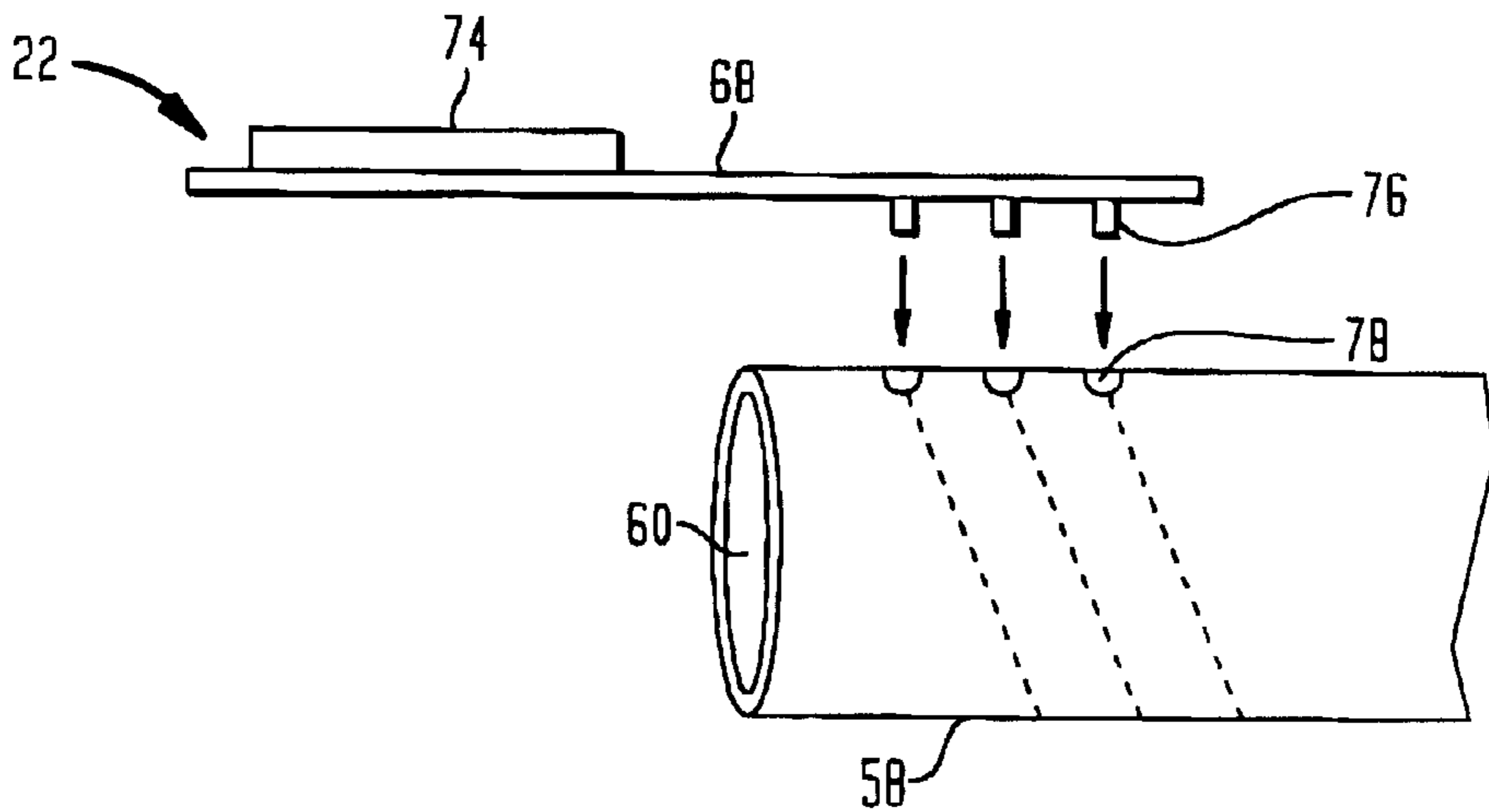
FIG. 5C
