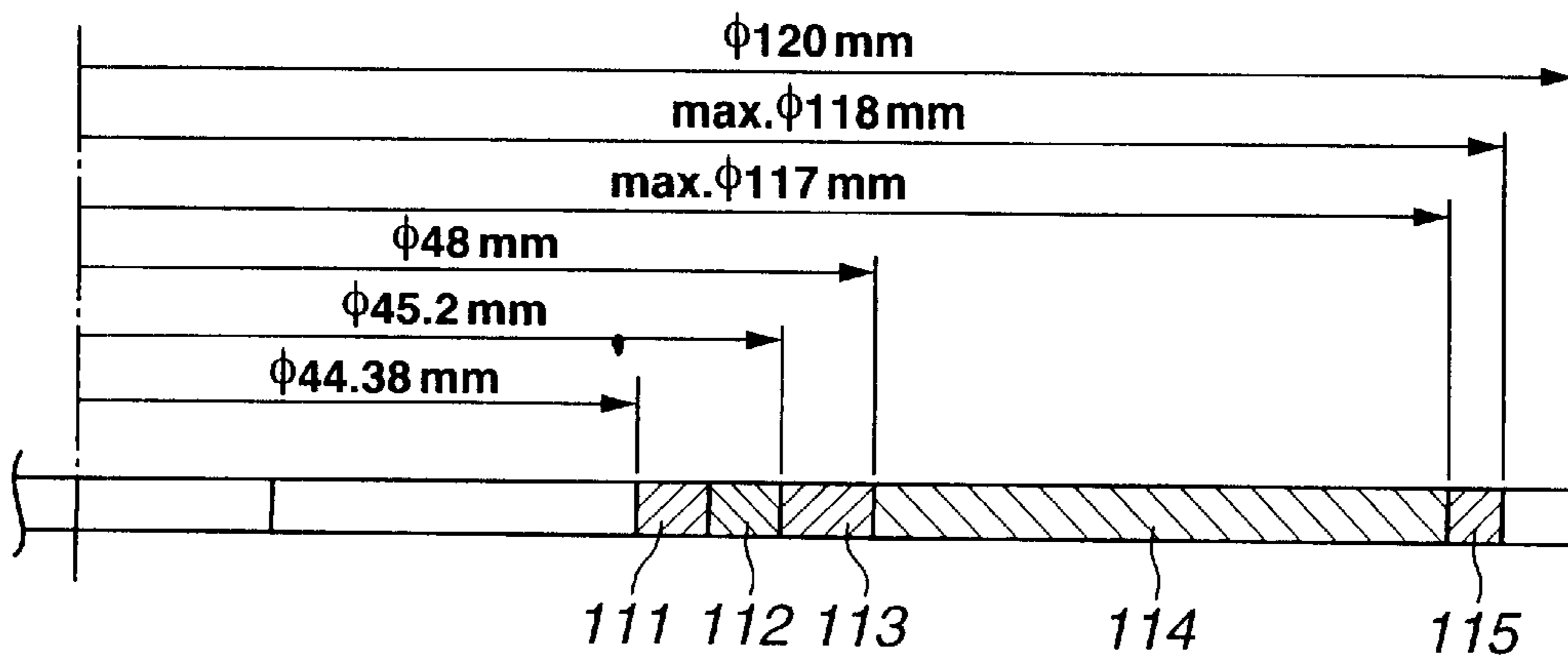
FIG.2B
