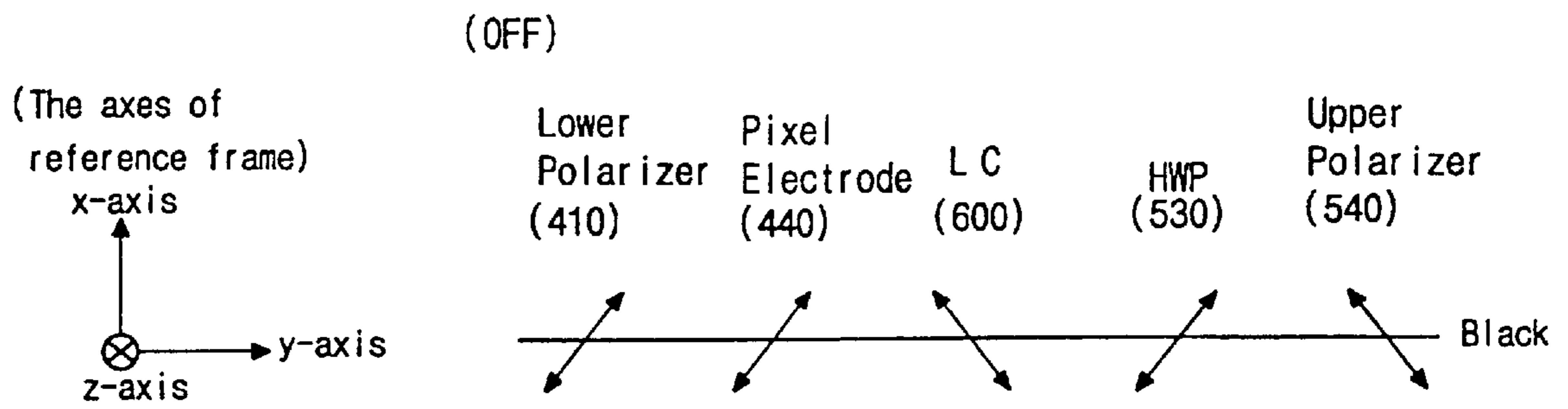
FIG. 8A
