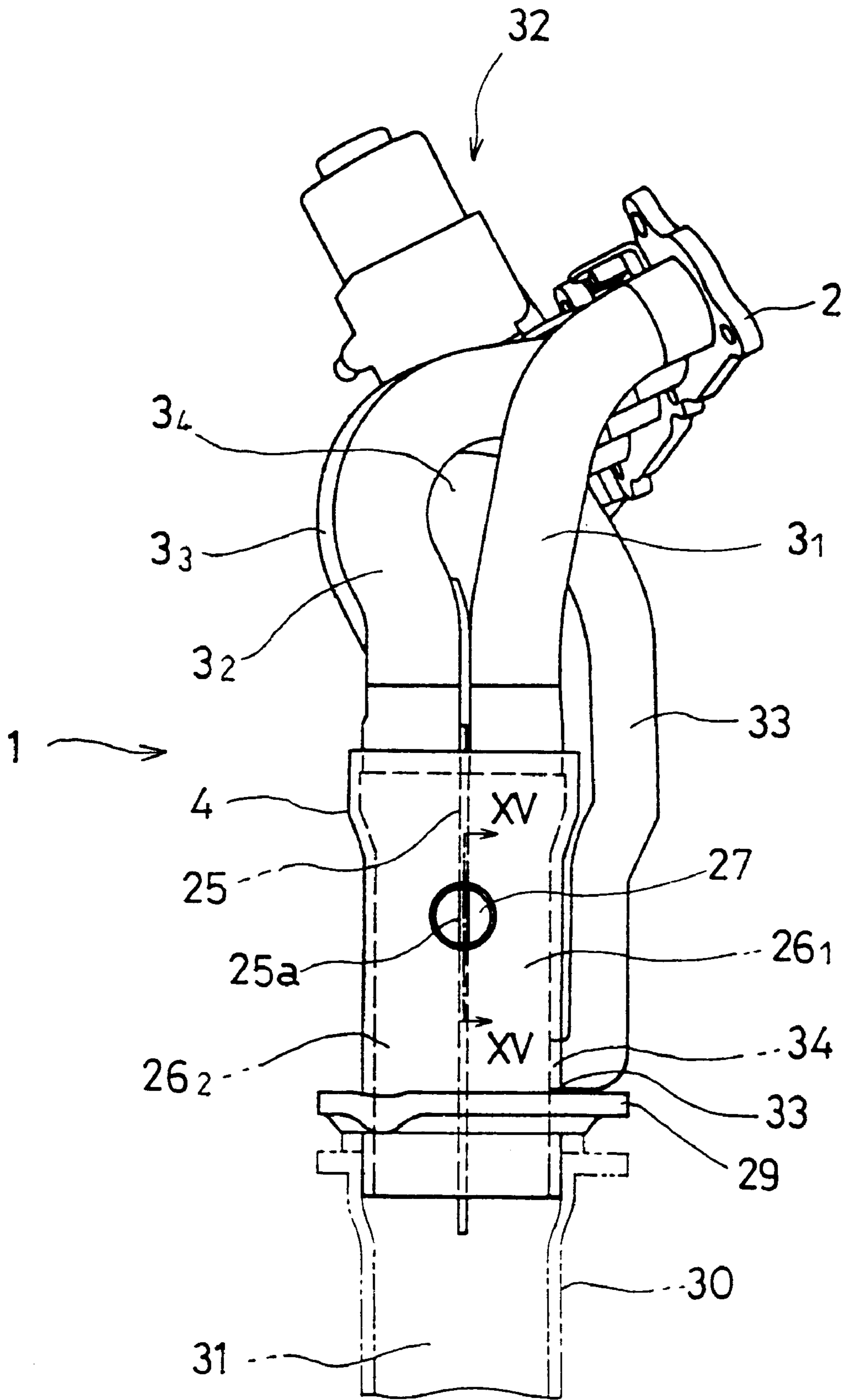
Fig.14
