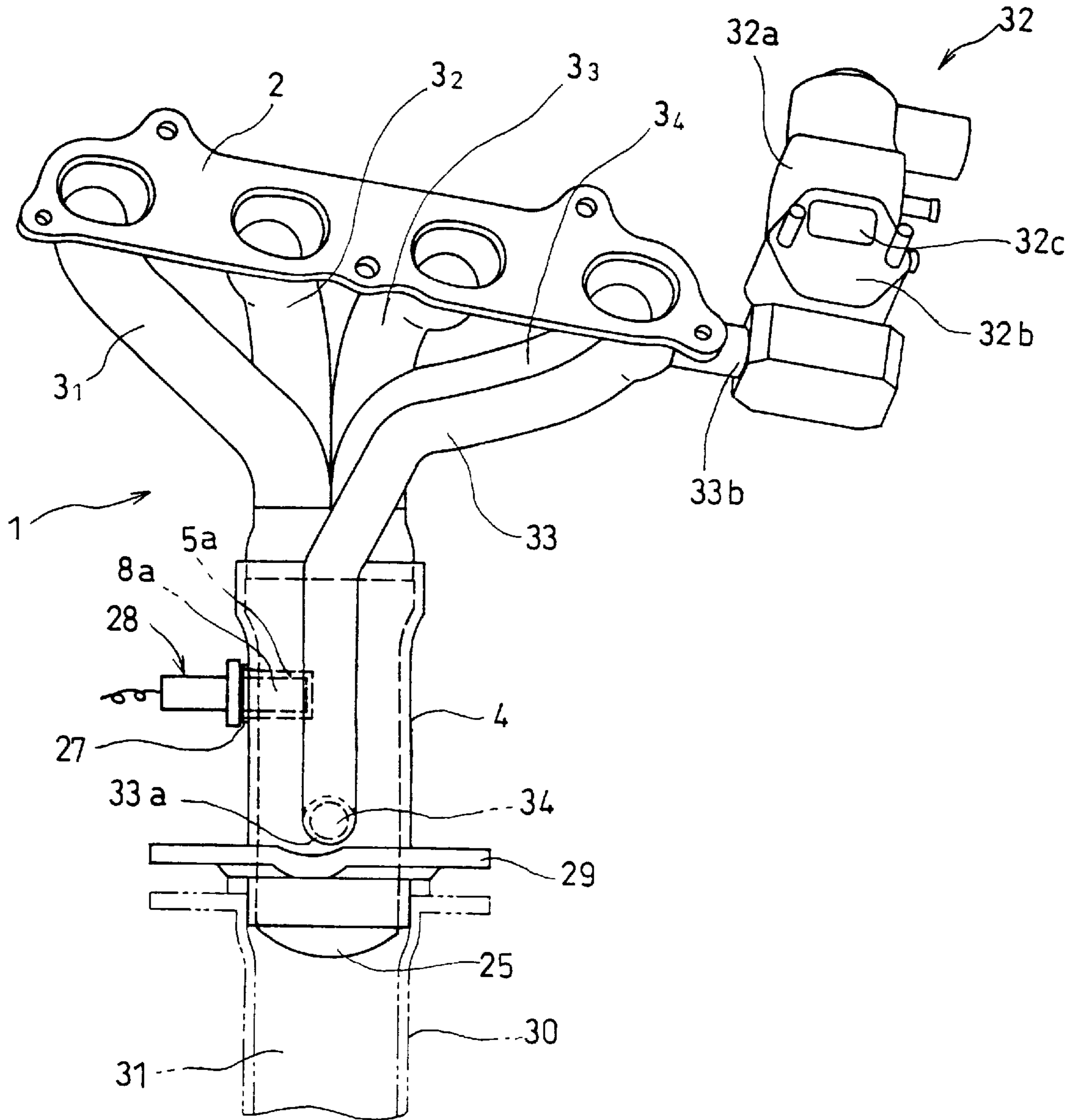
Fig.13
