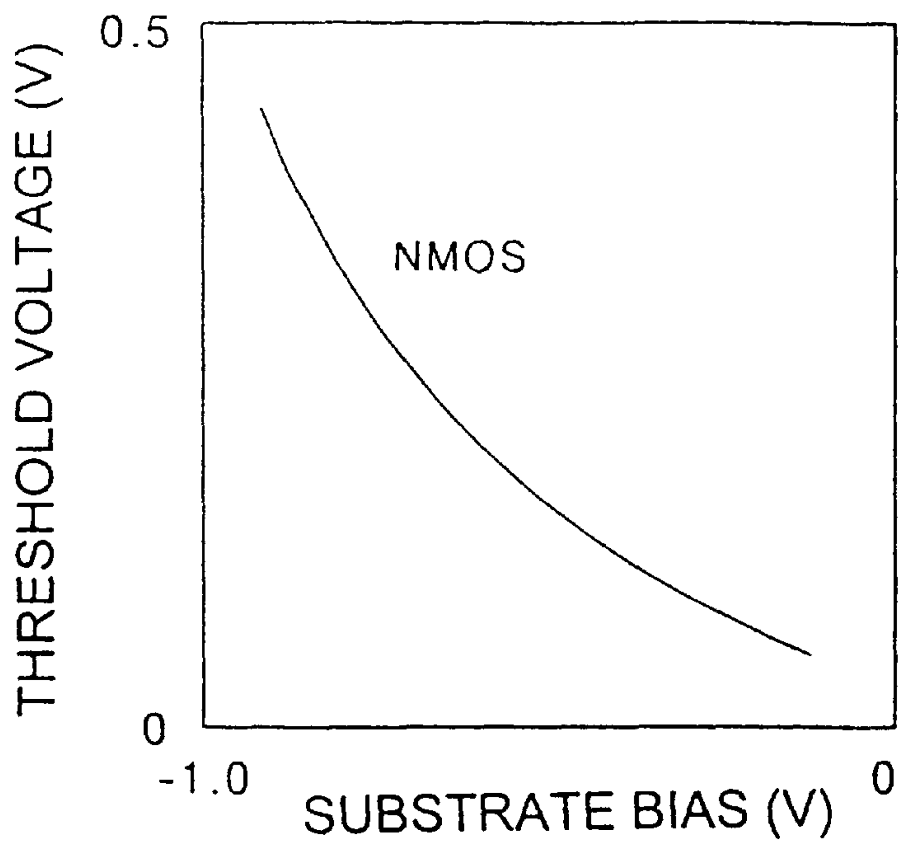
FIG. 7A
