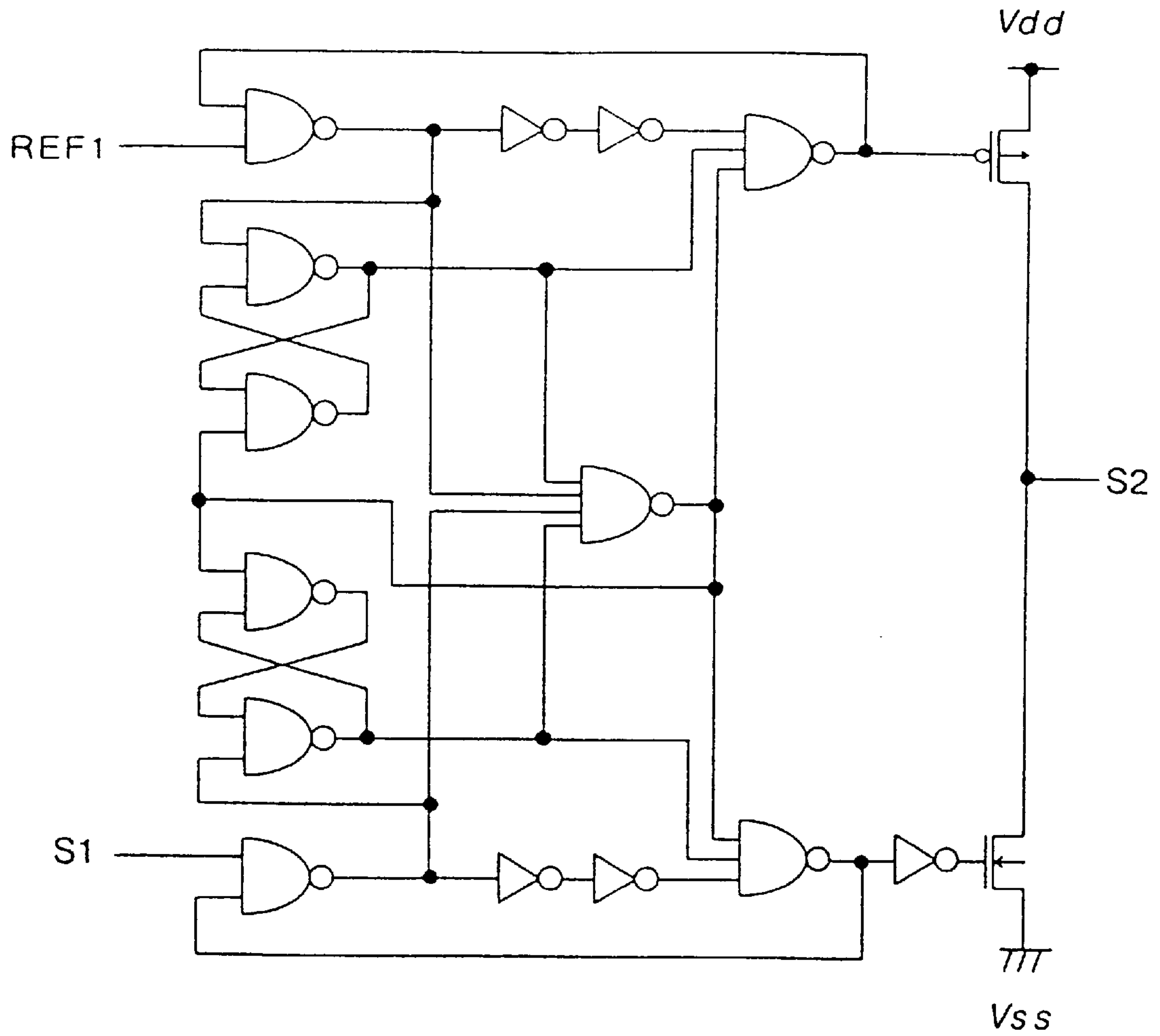
FIG. 5A
