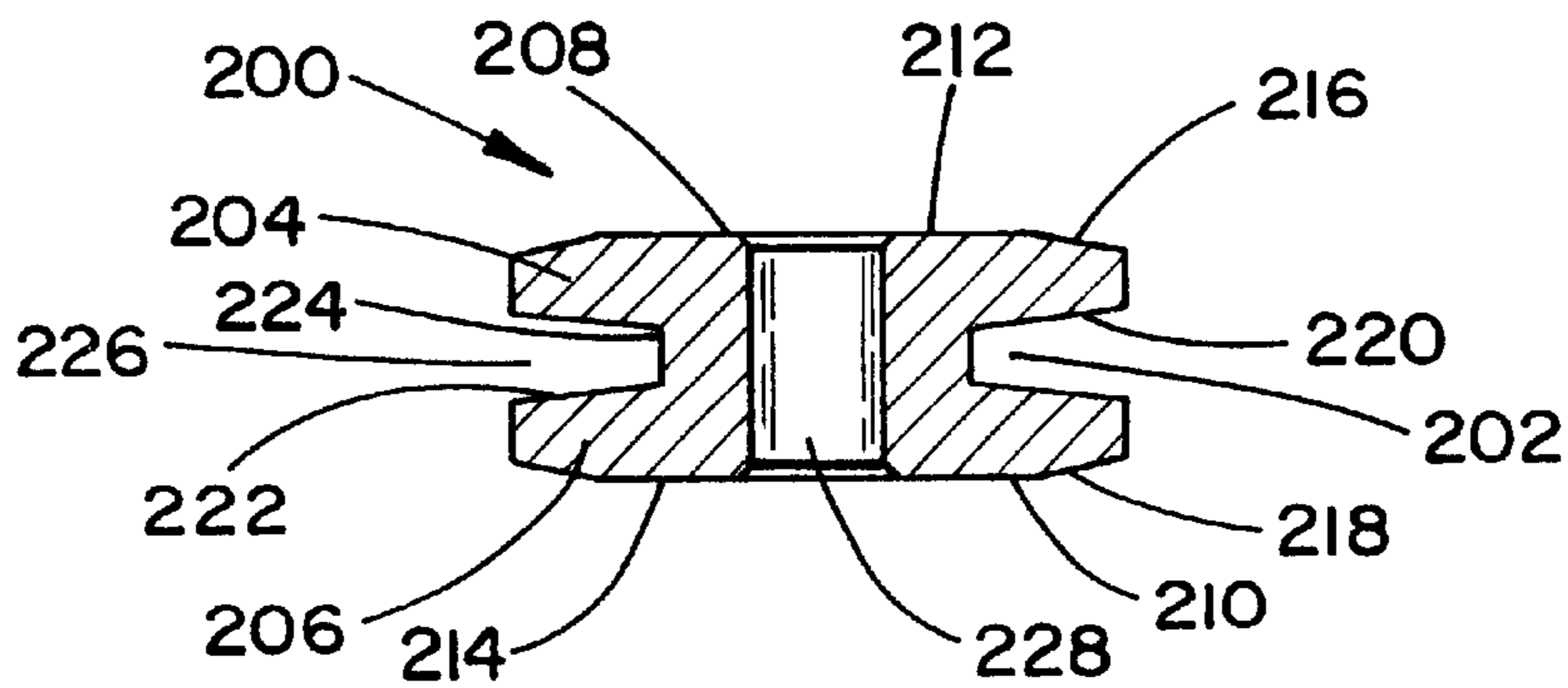
Section A-A
