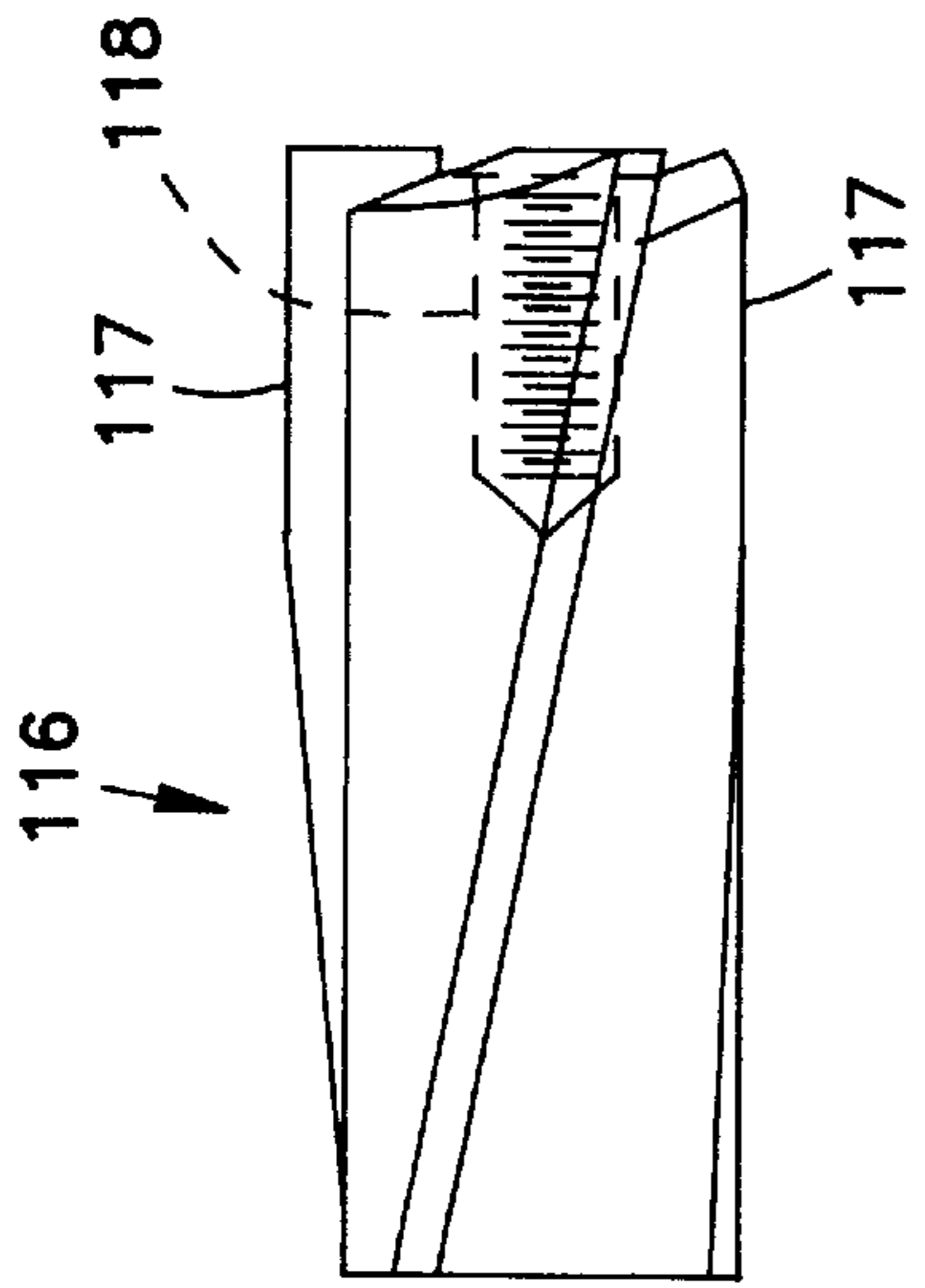
FIG. 17
