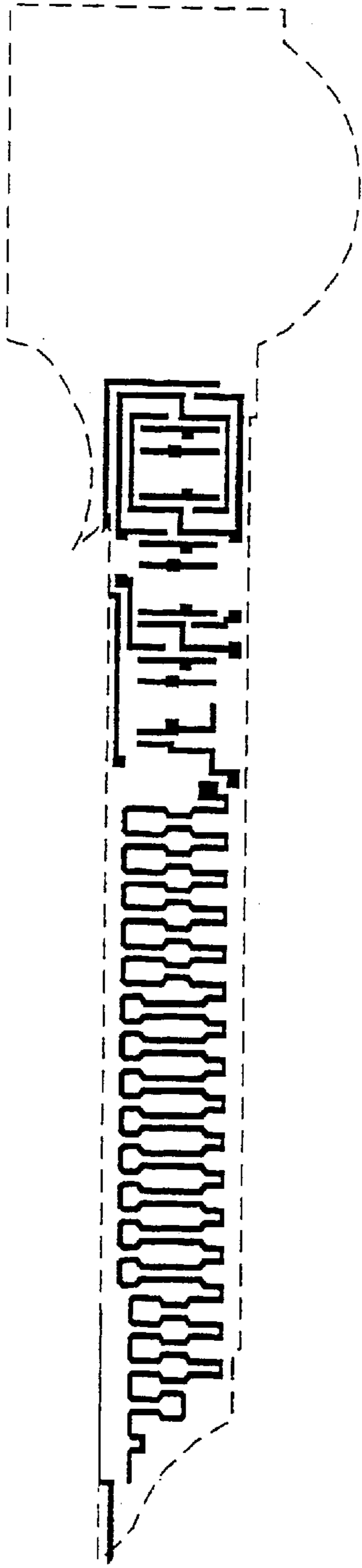
Poly mask
